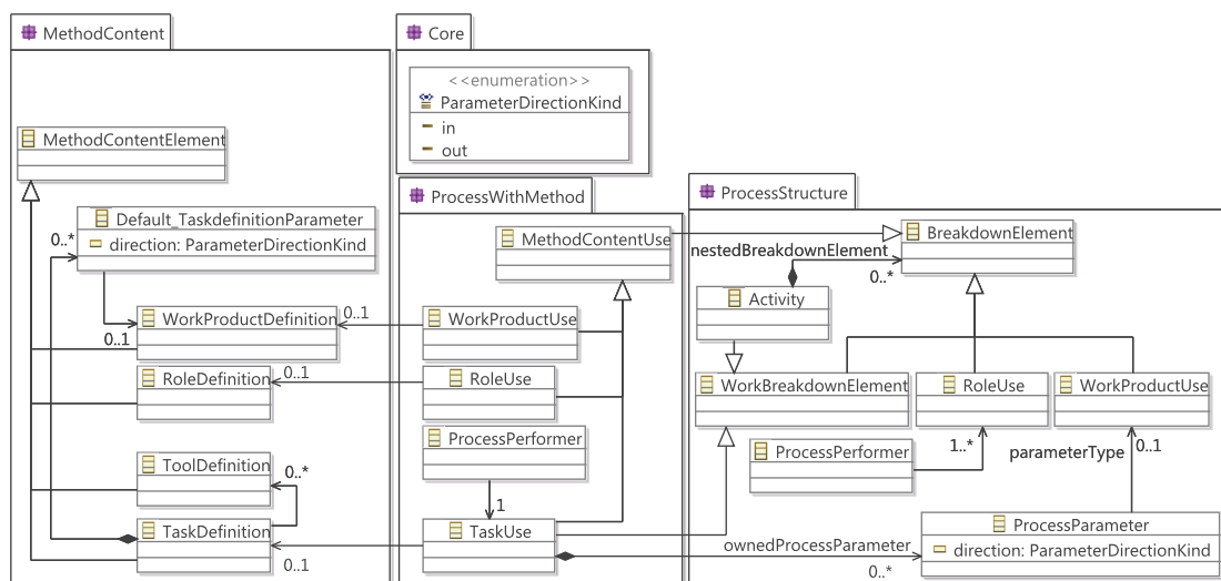
FIGURE 2.3 – Extraits de certains paquets du métamodèle de SPEM 2.0
