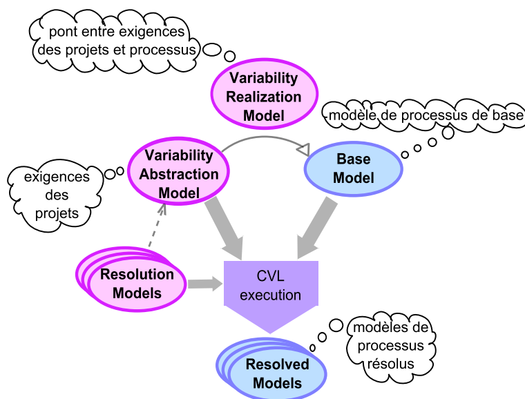
FIGURE 4.4 – Aperçu de l'approche consistant à utiliser CVL pour gérer la variabilité dans les processus de développement logiciel
