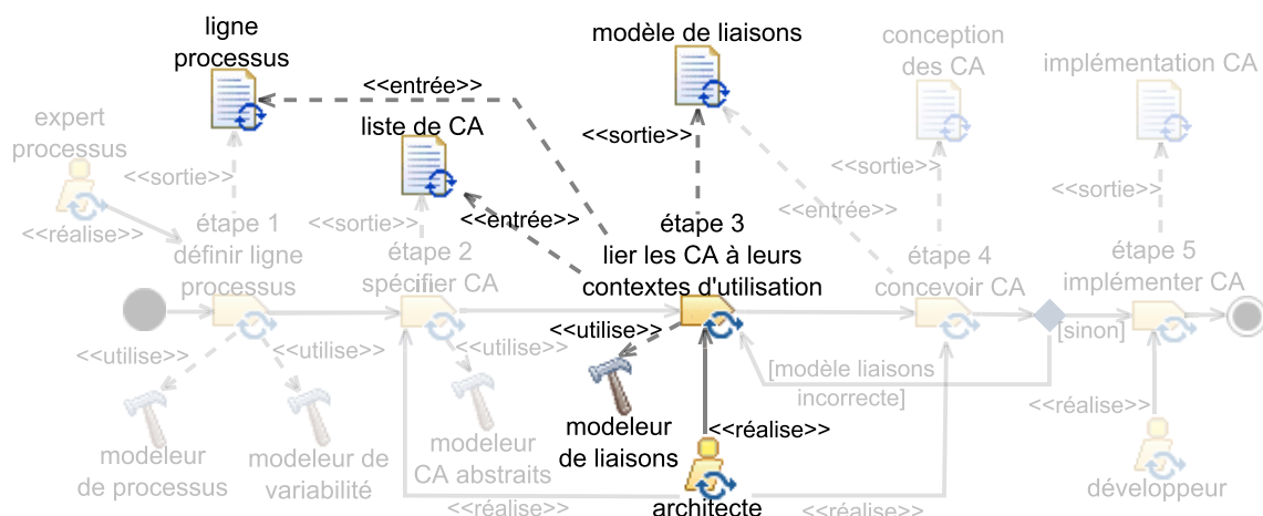
FIGURE 5.7 – Troisième étape de M4RAC
