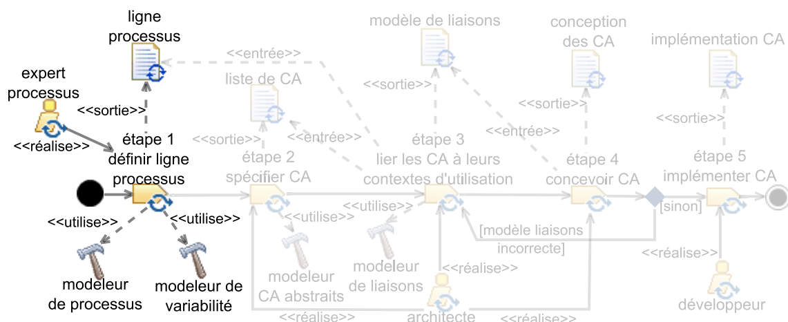
FIGURE 5.4 – Première étape de M4RAC
