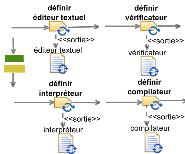
FIGURE 4.8 – Eléments de processus externes de l'exemple illustratif
