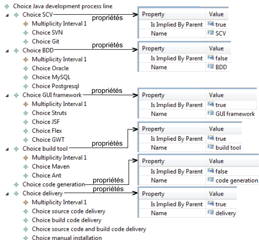
FIGURE B.1 – Extrait du VAM de la famille de processus de développement web Java
