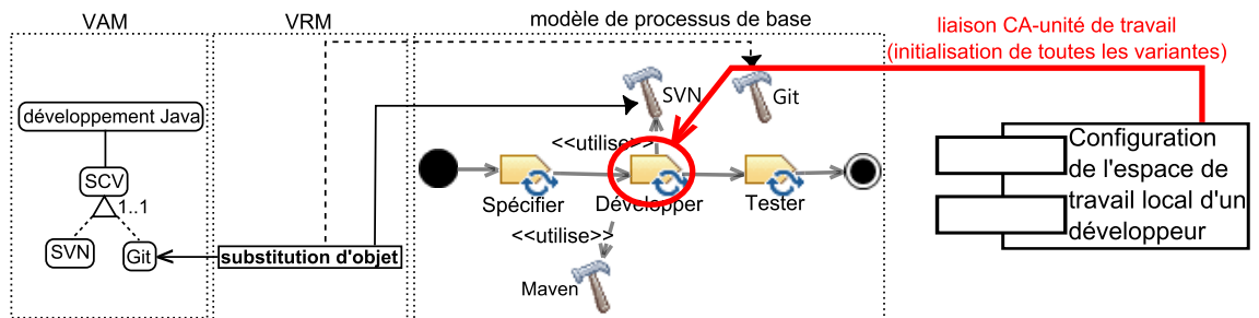
FIGURE 5.8 – Liaison entre le CA configurant l’espace de travail d’un développeur et la ligne de processus de la figure 5.5
