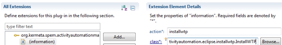
FIGURE B.4 – Déclaration de la classe implémentant l'action Java Eclipse install wtp
