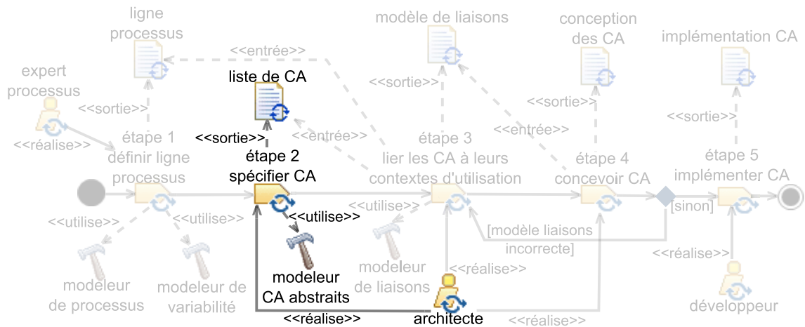
FIGURE 5.6 – Deuxième étape de M4RAC
