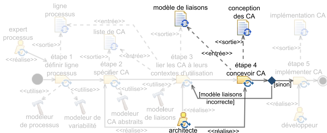
FIGURE 5.9 – Quatrième étape de M4RAC
