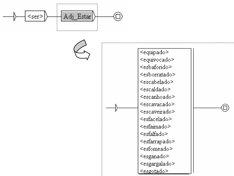
Figura 4. Grafo para identificação de sequências constituídas por um potencial Adj Hum que, nas matrizes , se encontra marcado como admitindo exclusivamente o Vcop estar (subgrafo Adj_Estar ), precedido de uma potencial forma do verbo ser .
