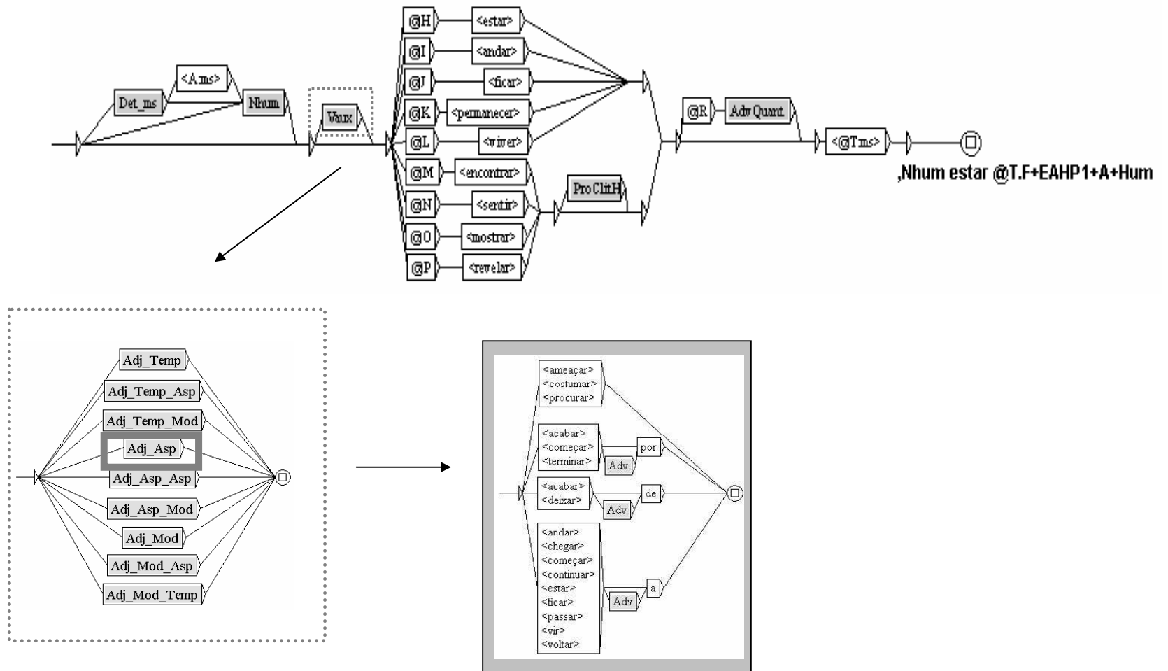
Figura 6. Fragmento da gramática EAH_ms.grf e respectivas chamadas aos subgrafos Vaux (caixa à esquerda) e Adj_Asp (caixa mais à direita)
