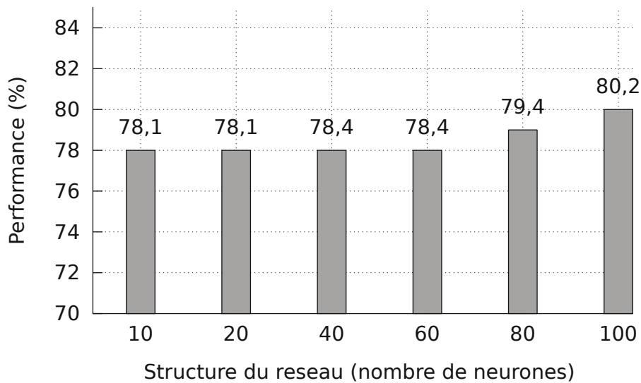
FIGURE 3.14: Performances des RNA simple couche en fonction de leur structure
