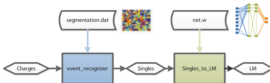
FIGURE 3.15: Représentation de la chaîne logicielle de reconstruction des événements et de ses dépendances
