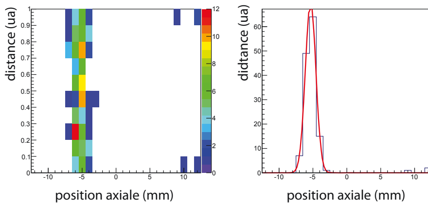
FIGURE 6.3: Représentation de l'histogramme de distance (gauche), et ajustement gaussien sur une projection selon z (droite)
