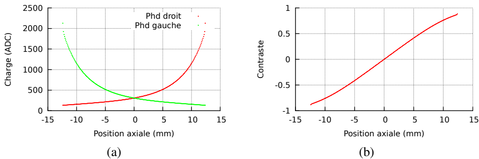
FIGURE 1.12: Information de charge en fonction de la position axiale : (a) Charges du photodétecteur (PhD) droit et gauche en fonction de la position axiale z , (b) Contraste en fonction de la position axiale (0 correspond au centre du cristal)
