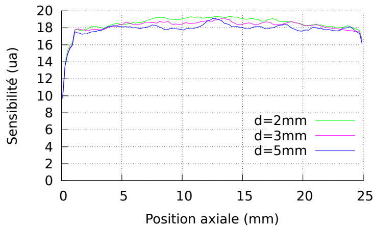
FIGURE 5.16: Profil de la sensibilité pour d = 2 mm et d = 5 mm
