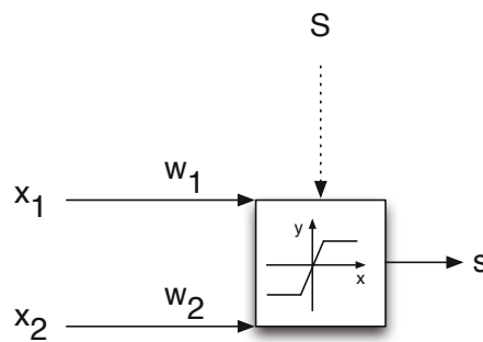
FIGURE 3.12: Représentation d'un neurone artificiel avec : deux entrées (x_1, x_2) pondérées par deux poids (w_1, w_2) , un seuil ( S ) et une sortie s
