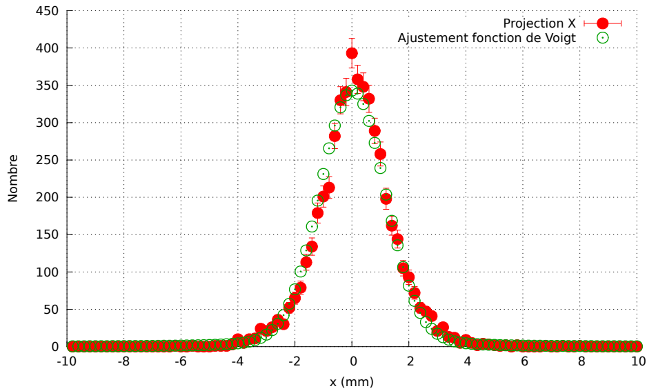
FIGURE 2.7: Projection 1-D selon l'axe des abscisses de la distribution 2-D de diffusion optique et ajustement avec la fonction de Voigt
