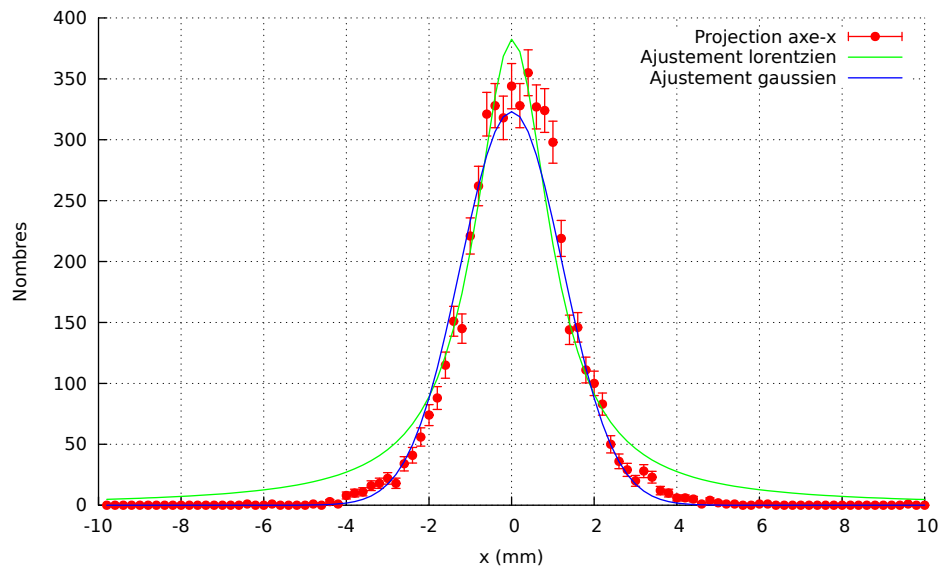
FIGURE 2.6: Projection 1-D selon l'axe des abscisses de la distribution 2-D de diffusion optique
