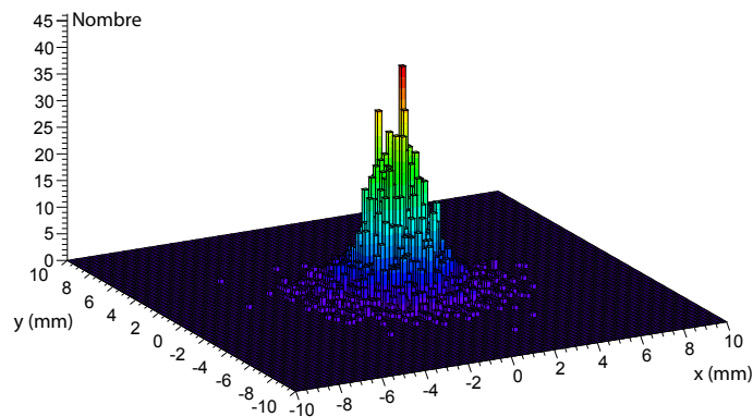
FIGURE 2.5: Distribution optique sur le plan d'entrée du photo-détecteur pour une réalisation à la position z = 0 mm
