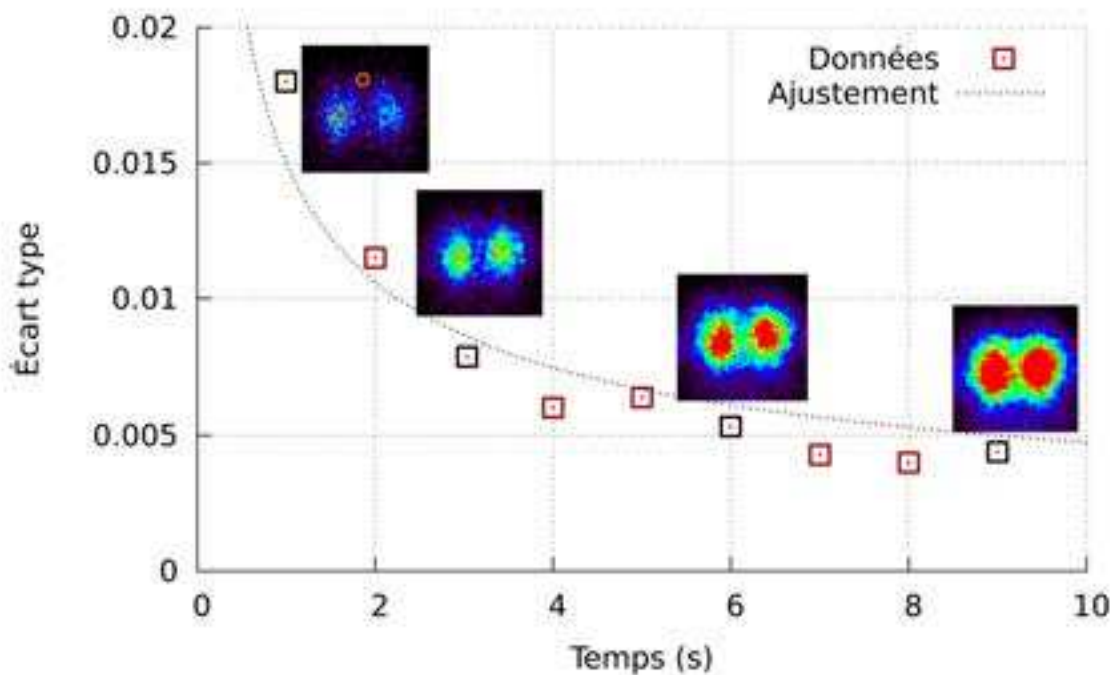
FIGURE 5.12: Évolution de l'écart type en fonction du temps d'acquisition avec un ajustement de type f(x) = a/\sqrt{x} (ajusté avec a = 0,015 )
