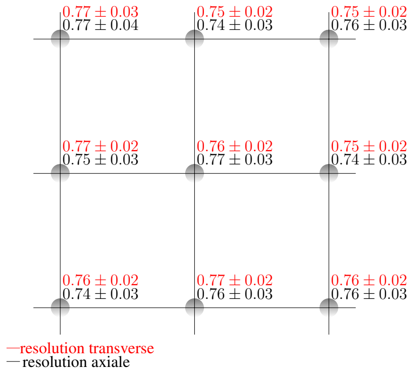
FIGURE 5.18: Résolutions spatiales axiale et transverse pour chaque point du fantôme de résolution pour d = 2 mm
