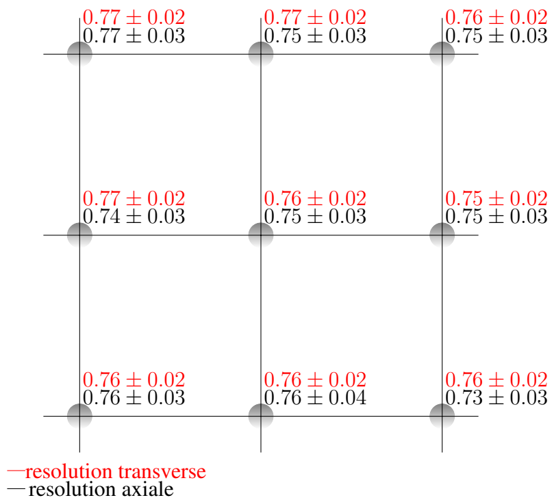
FIGURE 5.20: Résolutions spatiales axiale et transverse pour chaque point du fantôme de résolution pour d = 5 mm
