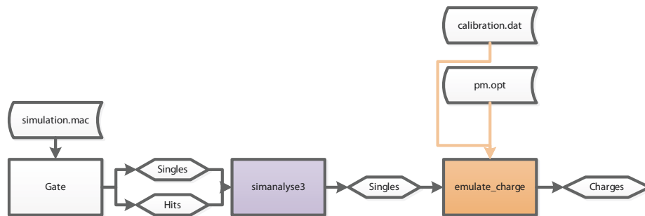
FIGURE 2.10: Représentation de la chaîne logicielle de simulation et de ses dépendances
