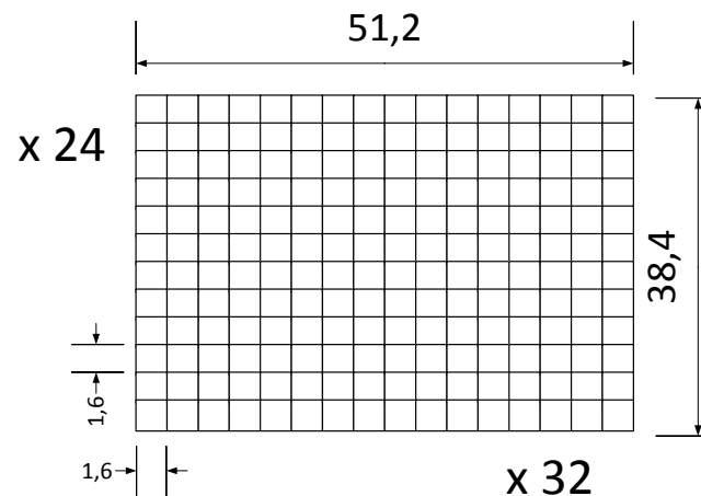
FIGURE 5.1: Représentation de la matrice de cristaux (toutes les dimensions sont en millimètres)
