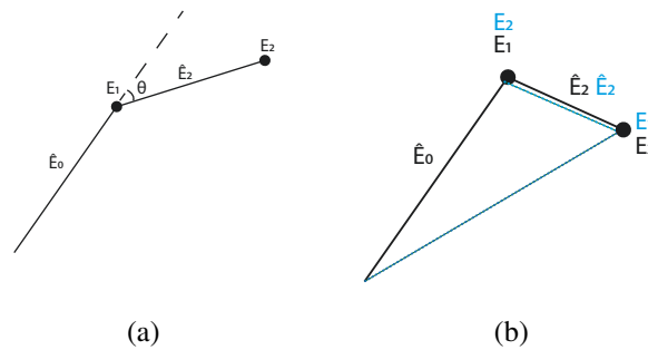
FIGURE 3.10: Cinématique Compton : (a) Région 1, (b) Région 2 cas ambigu
