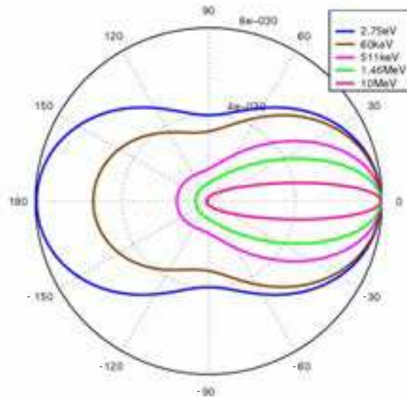
FIGURE 1.3: Diffusion angulaire Compton
