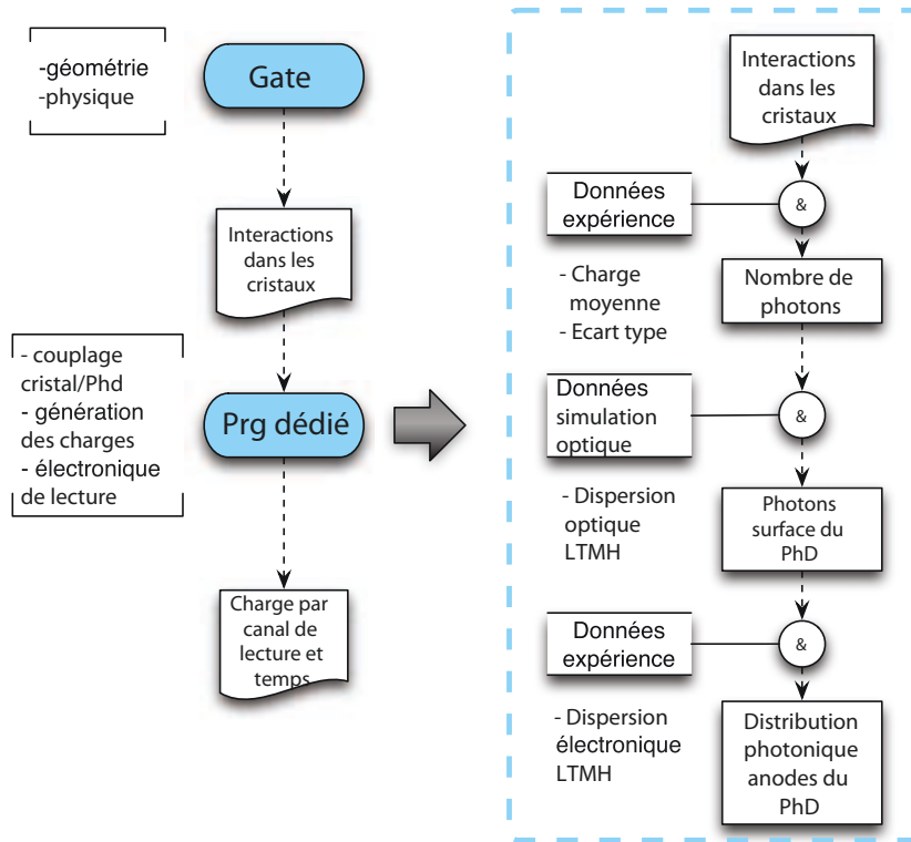
FIGURE 2.3: Chaîne des processus de la simulation complète de l'imageur
