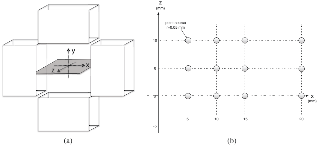
FIGURE 5.3: (a) Localisation du plan du fantôme de résolution, (b) Répartition des points sources dans le plan y = 0
