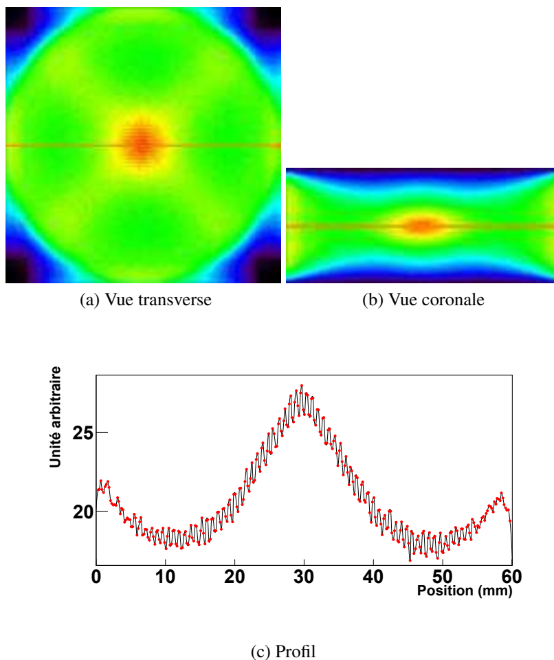
FIGURE 4.2: Représentation de l'image de sensibilité
