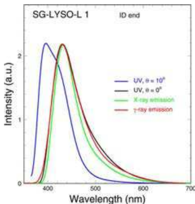
FIGURE 1.4: Spectre d'émission de LYSO : Ce excité par UV, rayon X et gamma (R. Mao et coll. 2008)
