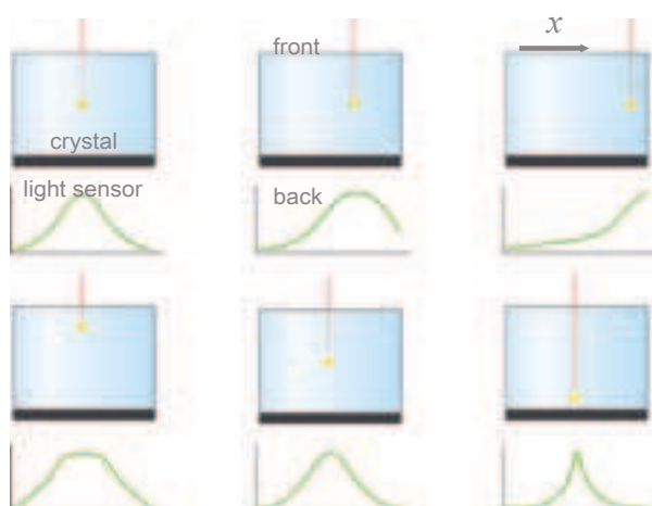
FIGURE 1.10: Variation de la distribution optique en fonction de la position de l'interaction dans un module mono-bloc
