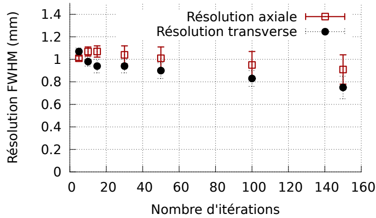
FIGURE 5.6: Résolution spatiale en fonction du nombre d'itérations (MLEM)
