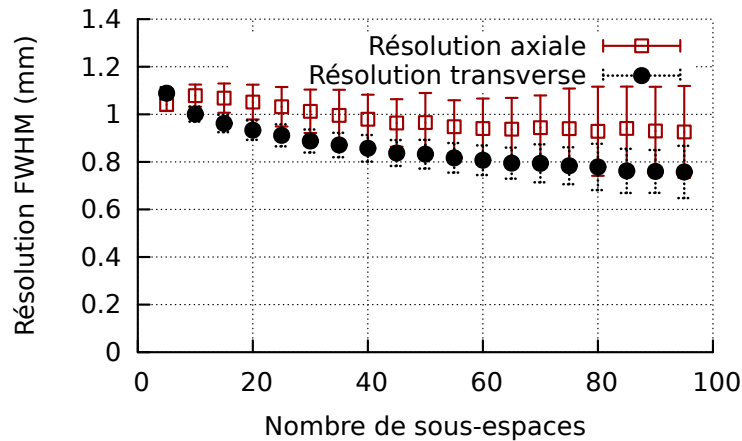
FIGURE 5.7: Résolution spatiale en fonction du nombre de sous-ensemble (OPL-EM)
