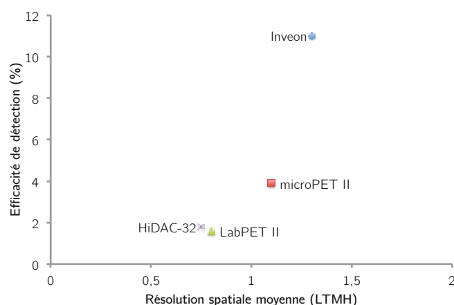
FIGURE 1.15: Distribution des tomographes haute-résolution ainsi que de l'Inveon en fonction de leur efficacité de détection
