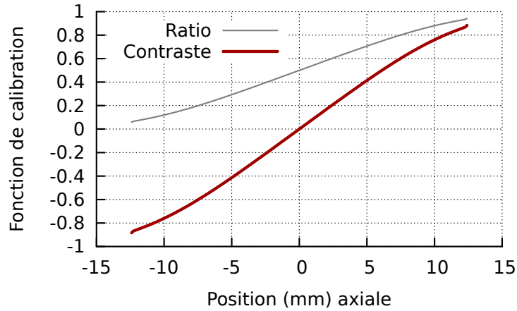
FIGURE 3.6: Fonctions de calibration : rapport entre l'une des charges et la somme et contraste
