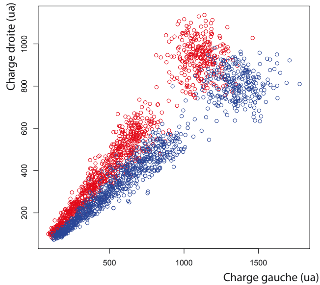
FIGURE 6.2: Représentation de l'espace des attributs pour deux positions axiales z = 1 mm (rouge) et z = 3 mm (bleu)
