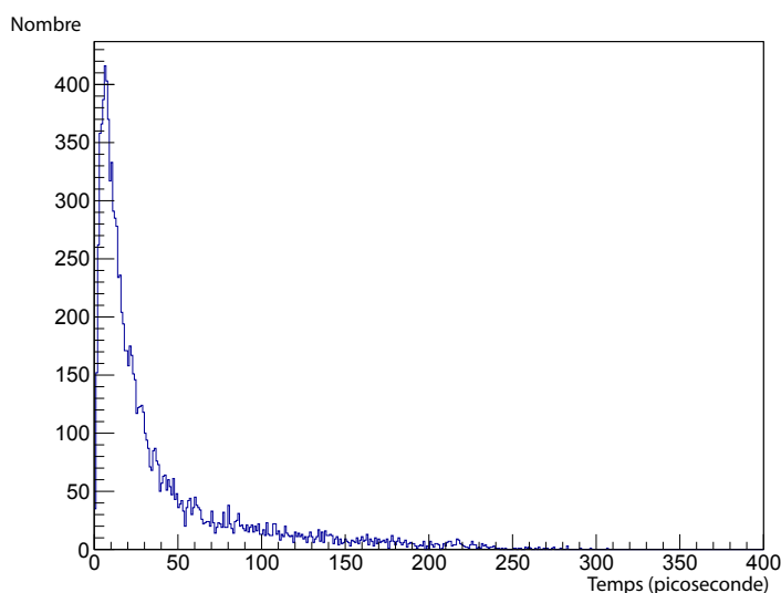
FIGURE 3.11: Distribution de la différence en temps pour deux interactions successives dans un module
