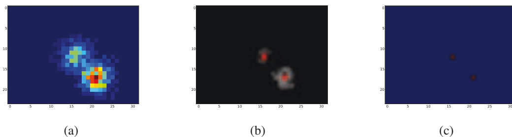
FIGURE 3.2: Étapes principales de l'algorithme de recherche des maxima : (a) Distribution originale de charges, (b) conversion en niveau de gris et recherche des maxima, (c) après application des contraintes
