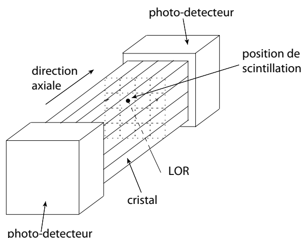
FIGURE 1.11: Matrice de cristaux orientés de façon axiale
