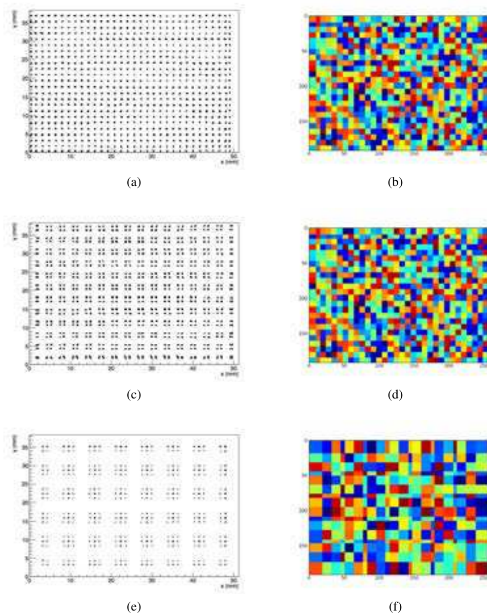
FIGURE 3.4: Histogramme de positions et matrice de correspondance en fonction du couplage cristal–photo-détecteur : (a) Histogramme de position couplage (1 :1), (b) Matrice de correction des positions couplage (1 :1), (c) Histogramme de position couplage (4 :1), (d) Matrice de correction des positions couplage (4 :1), (e) Histogramme de position couplage (8 :1), (f) Matrice de correction des positions couplage (8 :1)
