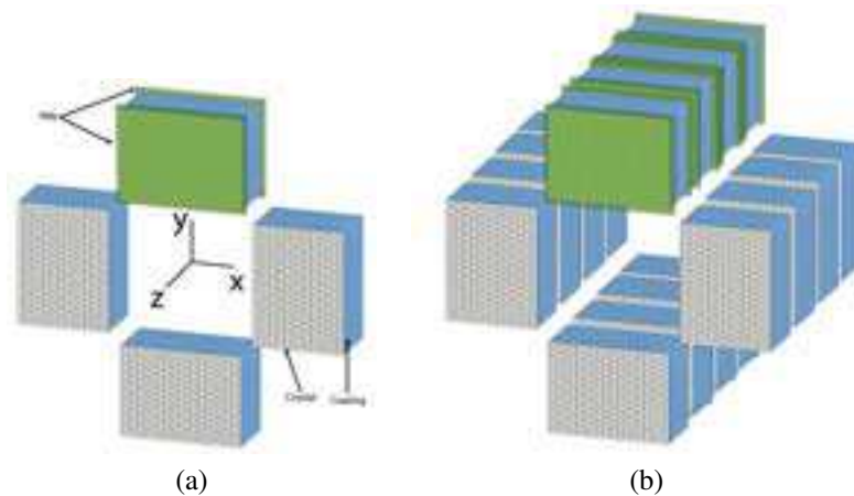
FIGURE 2.1: Prototypes simulés : (a) Configuration géométrique à 4 modules (seul un module est représenté avec ses deux photo-détecteurs), (b) Configuration géométrique à 16 modules (seuls 4 modules sont représentés avec leurs deux photo-détecteurs respectifs)
