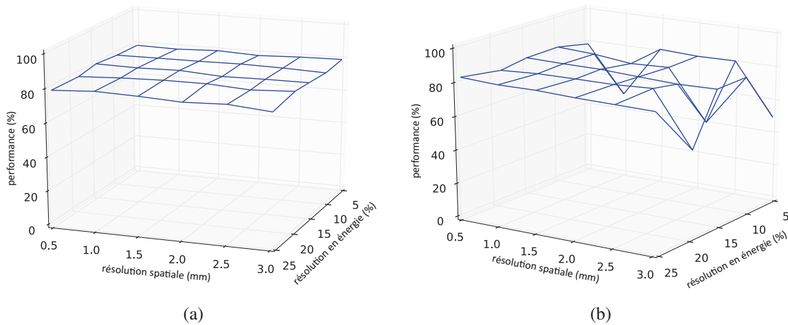
FIGURE 3.13: Performances d'un RNA en fonction des paramètres de résolution : (a) : RNA simple couche de 100 neurones (b) : RNA double couches de (100,100) neurones
