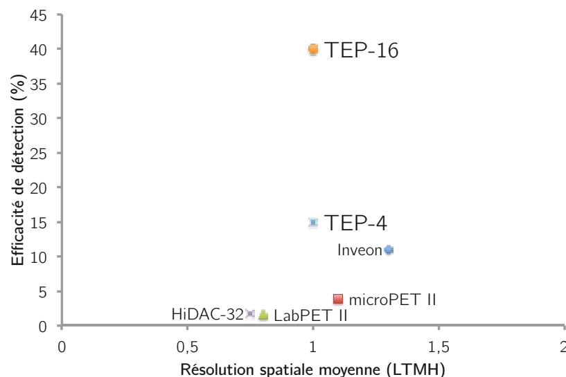
FIGURE 5.21: Performances simulées des prototypes à 4 et 16 modules (études spécifiques) par rapport à l'état de l'art en imagerie préclinique (études NEMA-NU4)
