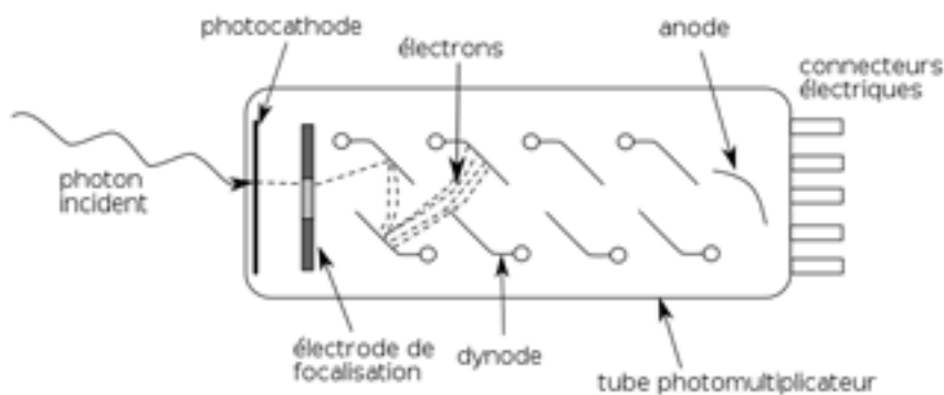
FIGURE 1.5: Schéma d'un tube photomultiplicateur
