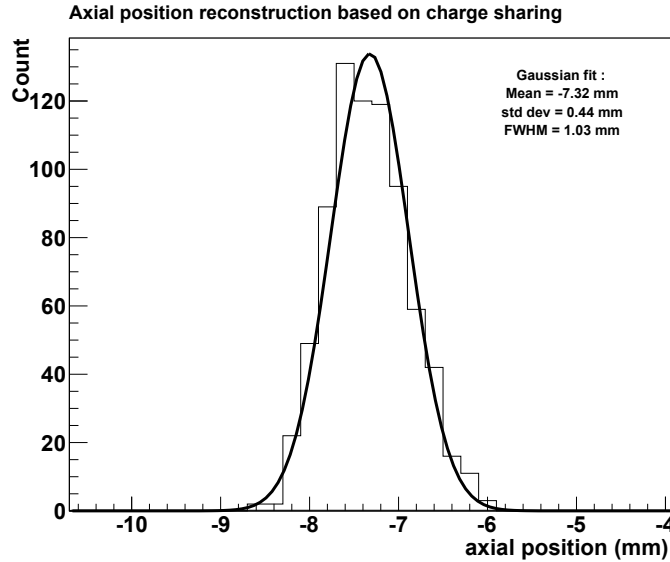
FIGURE 3.5: Reconstruction de la position axiale avec la méthode du contraste
