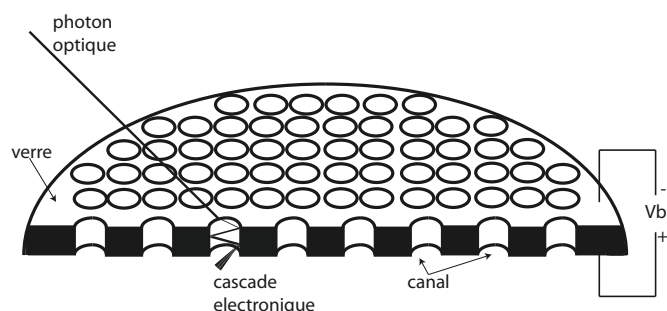
FIGURE 1.6: Schéma d'une matrice de galette de micro-canaux avec multiplication électronique
