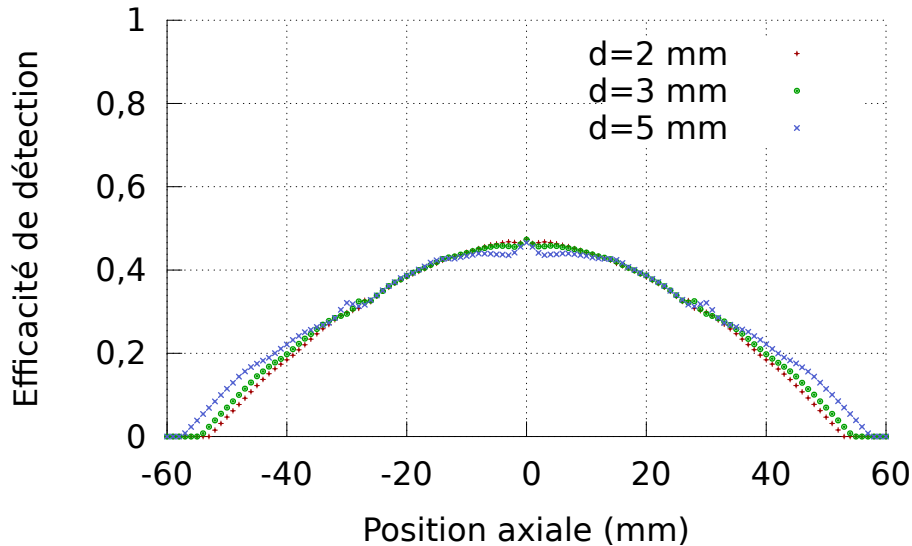
FIGURE 5.15: Profil de l'efficacité de détection absolue pour x = 0 et y = 0
