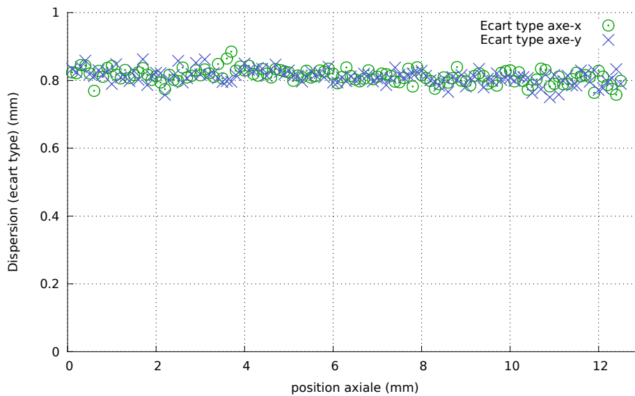
FIGURE 2.8: Écart type selon l'axe x et y de l'ajustement gaussien de la projection de la distribution optique en fonction de la position axiale
