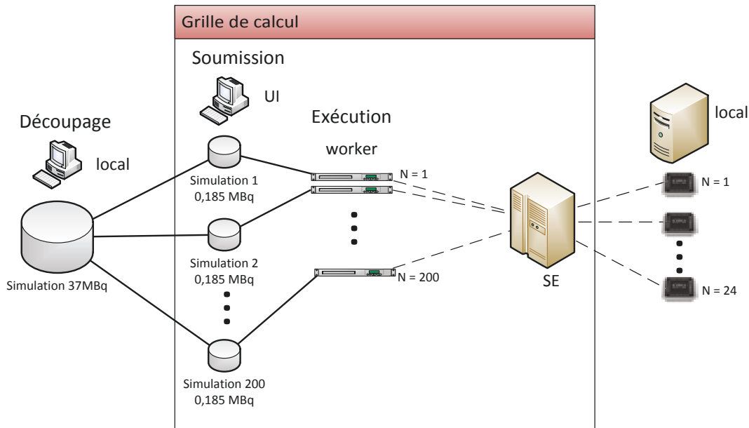
FIGURE 2.9: Architecture de la simulation du tomographe
