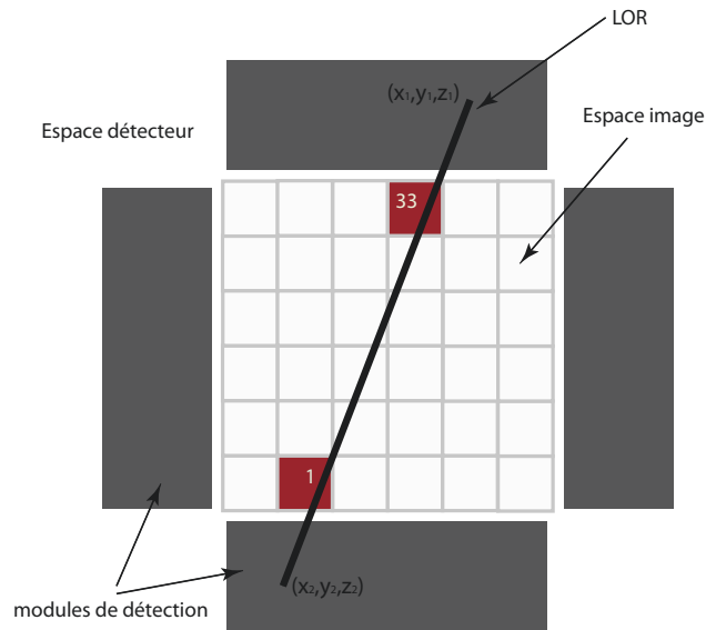
FIGURE 4.3: Projection de la LOR dans l'espace image
