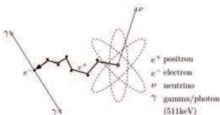
FIGURE 1.1: Émission et annihilation du positron
