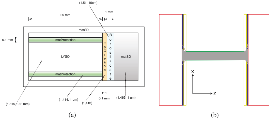
FIGURE 2.4: Simulation optique : (a) Géométrie de la simulation avec la valeur de l'indice de réfraction et la longueur d'absorption du milieu (seul le photo-détecteur droit est représenté), (b) Capture d'écran d'une simulation en cours d'exécution
