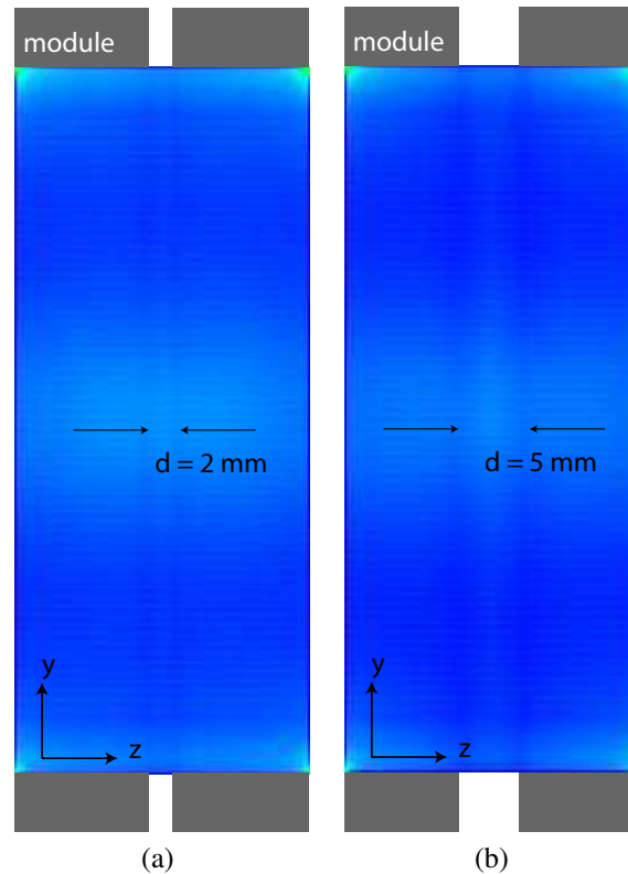
FIGURE 5.17: Vue sagittale de l'image de sensibilité : (a) d = 2 mm, (b) d = 5 mm
