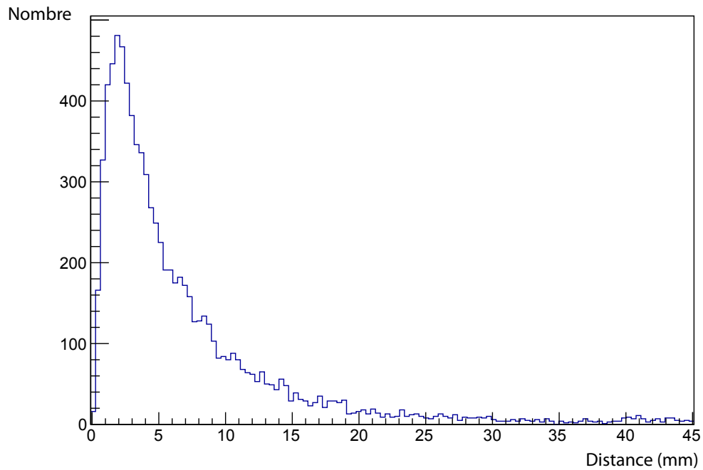
FIGURE 3.9: Distribution de la distance inter-cristaux entre deux interactions (deux interactions détectées dans le module)
