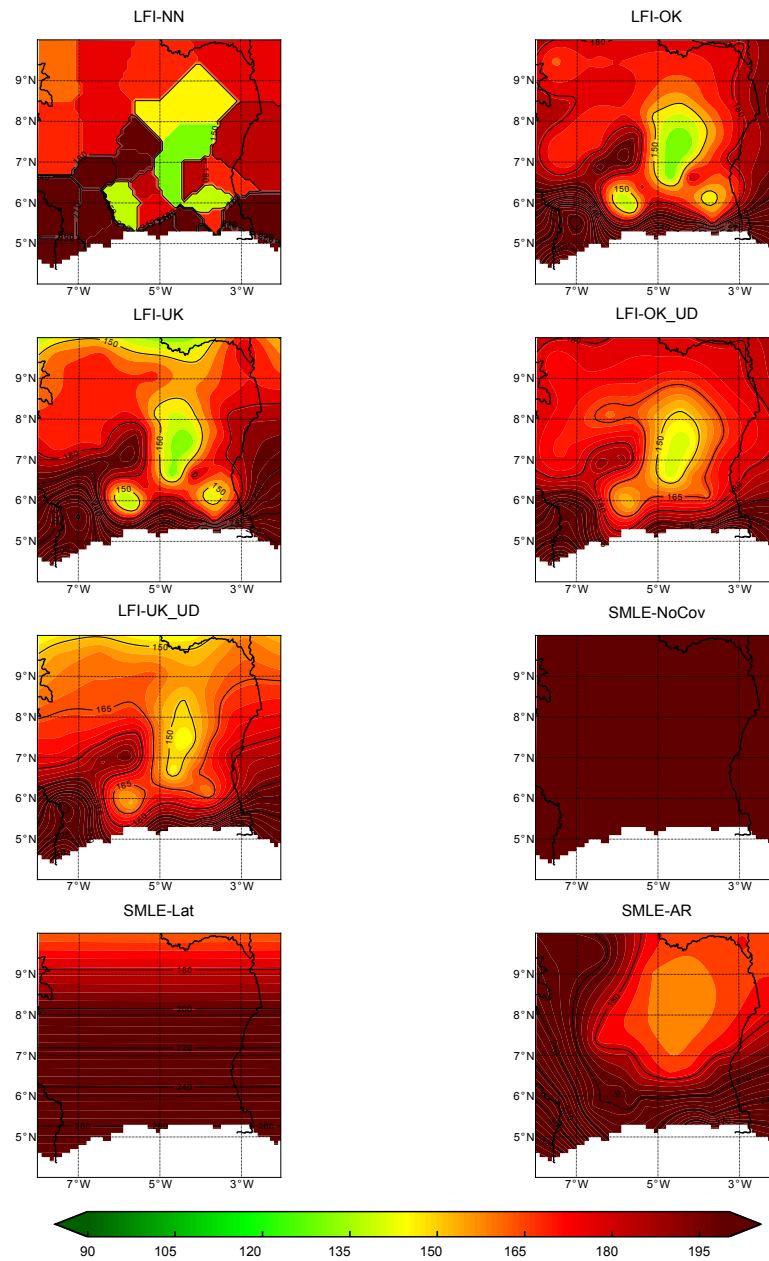
FIGURE D.13 – Niveaux de retour estimés par les modèles SMLE et LFI pour la période de retour T_r = 100 ans
