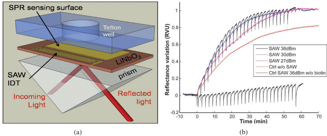
FIGURE 1.26: Schéma de principe montrant l'intégration de la surface sensible à l'SPR et des peignes interdigués du dispositif SAW sur un même substrat LiNbO 3 - Extrait de [18]
