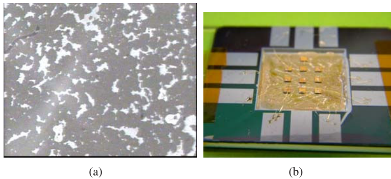
FIGURE 2.50: (a) Répartition de la colle sur la membrane (b) Des piézocéramiques miniatures collées sur la membrane en silisium
