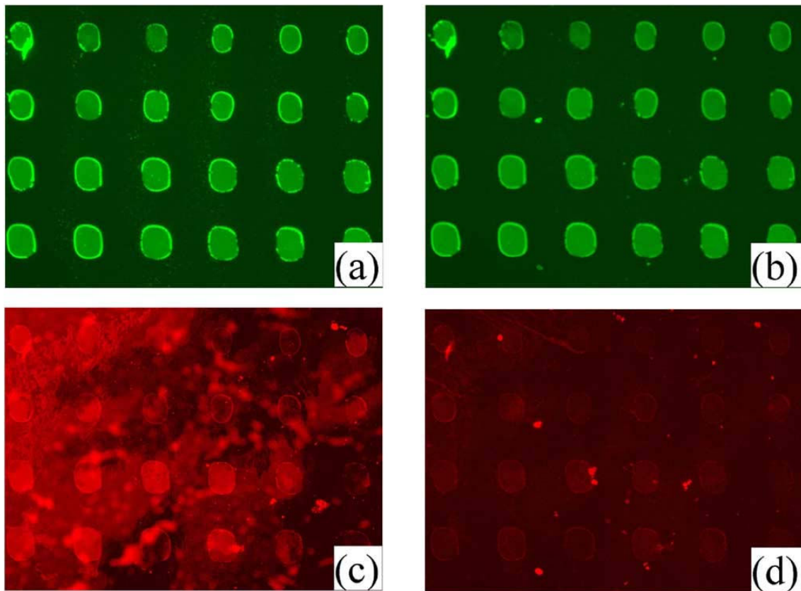
FIGURE 1.29: Images d'une marice de spots immobilisés en anticorps (a) avant et (b) après le rinçage acoustique. Matrice de spots d'antigène (c) immobilisés de façons spécifique et non spécifique (d) après le rinçage acoustique - Extrait de [20]
