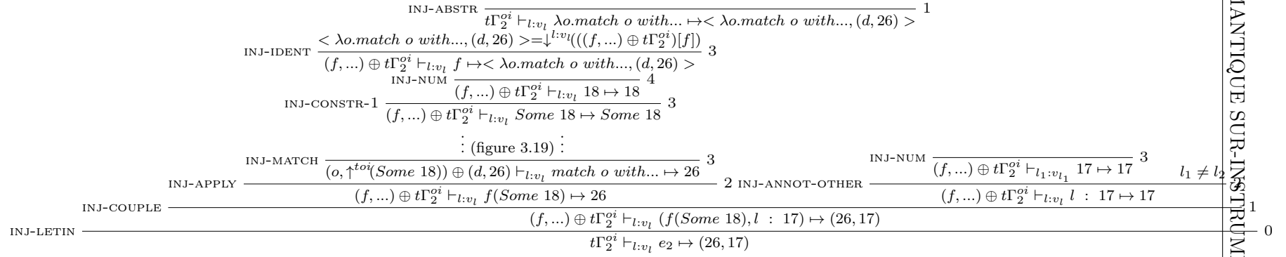
FIGURE 3.18 – Exemple 2 : arbre de dérivation du jugement d'évaluation avec injection sur l \notin \{l_1, l_2\}
