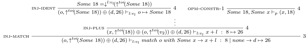
FIGURE 3.19 – Exemple 2 : sous-arbre de dérivation du filtrage avec injection sur l \notin \{l_1, l_2\}
