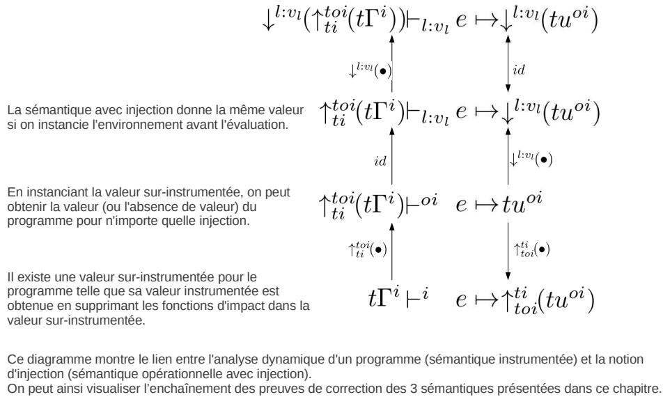
FIGURE 3.2 – Enchaînement des preuves des sémantiques intermédiaires pour l'analyse dynamique
