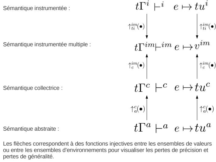
FIGURE 4.1 – Sémantiques intermédiaires pour l'analyse statique
