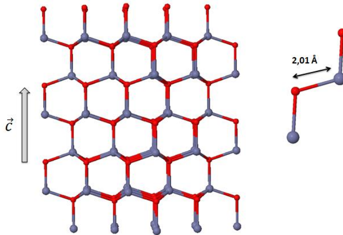
Figure 5.3 : ZnO sous phase wurtzite calculée avec VASP en DFT-GGA
