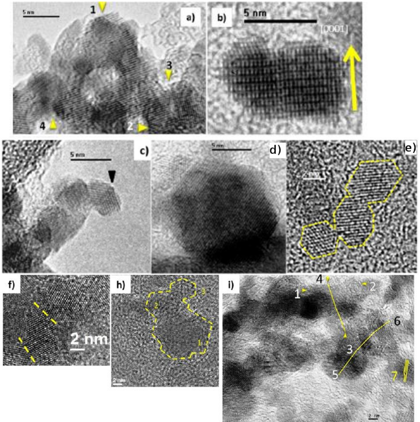
Figure 3.17 : Illustrations en HRTEM d'amas de nanoparticules de ZnO stœchiométriques en ultra-haut vide non triées en taille.
