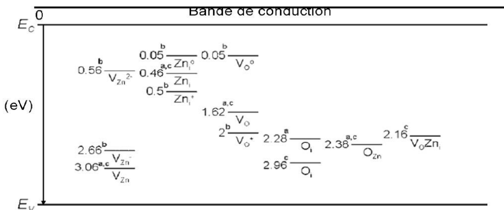
Figure 1.15 : Répartition des niveaux d'énergie profonds dus aux défauts
