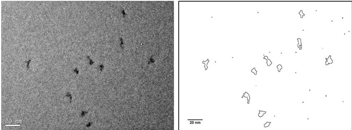
Figure 3.4 : Illustration du seuillage effectué sur Image J ( V_D=1000V )
