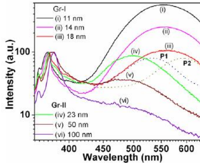
Figure 1.31 : Evolution de la luminescence visible de nanoparticules en fonction de leur taille et de leur forme (groupe 1, particules sphériques de taille inférieure à 20 nm ; groupe 2, nanocolumnes, de taille supérieure à 20 nm). La contribution P2 disparaît à la transition 154
