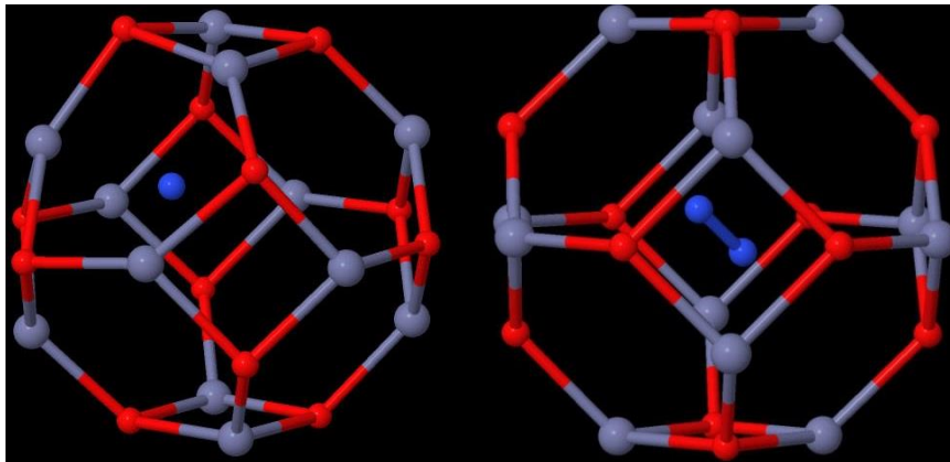
Figure 5.17 : A gauche, cage élémentaire d'un réseau de ZnO sodalite dopé à 1% avec N et contenant un seul dopant. A droite, cage élémentaire d'un réseau de ZnO sodalite dopé à 2% avec N aussi et contenant un dimère de dopants
