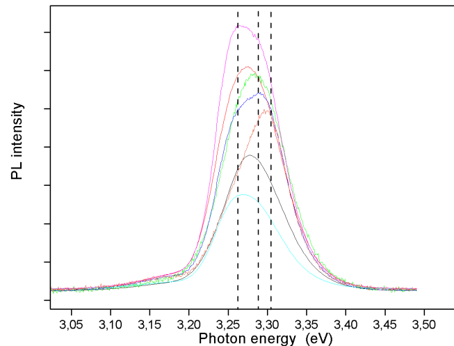
Figure 4.24 : Spectres de photoluminescence en mode confocal à température ambiante de différentes zones d'un échantillon stœchiométrique de 207 nm d'épaisseur équivalente. Sont représentées les contributions du FX non confiné (la plus énergétique), FX-1LO (la moins énergétique) et d'une autre contribution encore non identifiée (position intermédiaire).
