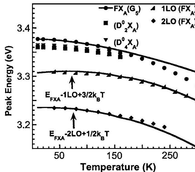
Fig 1.19 : Position du pic associé à FX_A et à ses répliques 1LO et 2LO ainsi que de deux pics DBE majeurs
