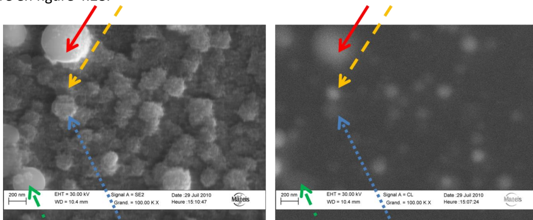
Figure 4.28 : Image MEB (à gauche) et cartographie en cathodoluminescence à 380 nm (à droite) d'une même zone de 2,5 \mu\text{m} \times 2 \mu\text{m} d'un film nanostructuré de 207 nm d'épaisseur équivalente stœchiométrique à température ambiante.
