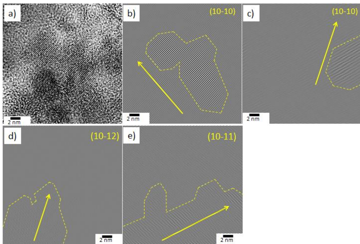
Figure 3.19 : Partie a) Plusieurs domaines cristallins coexistent au sein d'échantillons de nanoparticules de stœchiométriques non triées en taille. La partie b) illustre la transformée de Fourier de cette image et les parties c) à f) illustrent quelques plans cristallins détectés par filtrage de la transformée de Fourier. Les flèches jaunes indiquent la direction d'extension des domaines.
