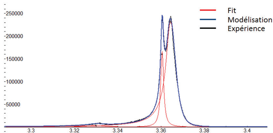
Figure 4.5 : Modélisation à l'aide de distributions lorentziennes symétriques et asymétriques des excitons liés à 15 K dans l'échantillon non stœchiométrique de 150 nm d'épaisseur équivalente
