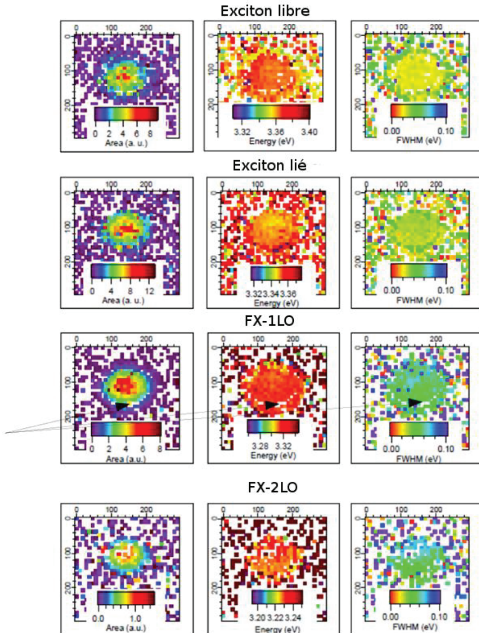
Figure 4.36 : Cartographie d'une particule de ZnO d'environ 150 nm de diamètre pour chacune des 4 contributions (FX, DX,FX-1LO, FX-2LO) que nous avons relevées dans les figures précédentes. La colonne la plus à gauche correspond à des cartographies de l'intensité de chacune des contributions. La colonne du milieu illustre les cartographies des positions énergétiques de chaque contribution. Enfin la colonne de droite indique les cartographies des largeurs à mi-hauteur de chacune des contributions.
