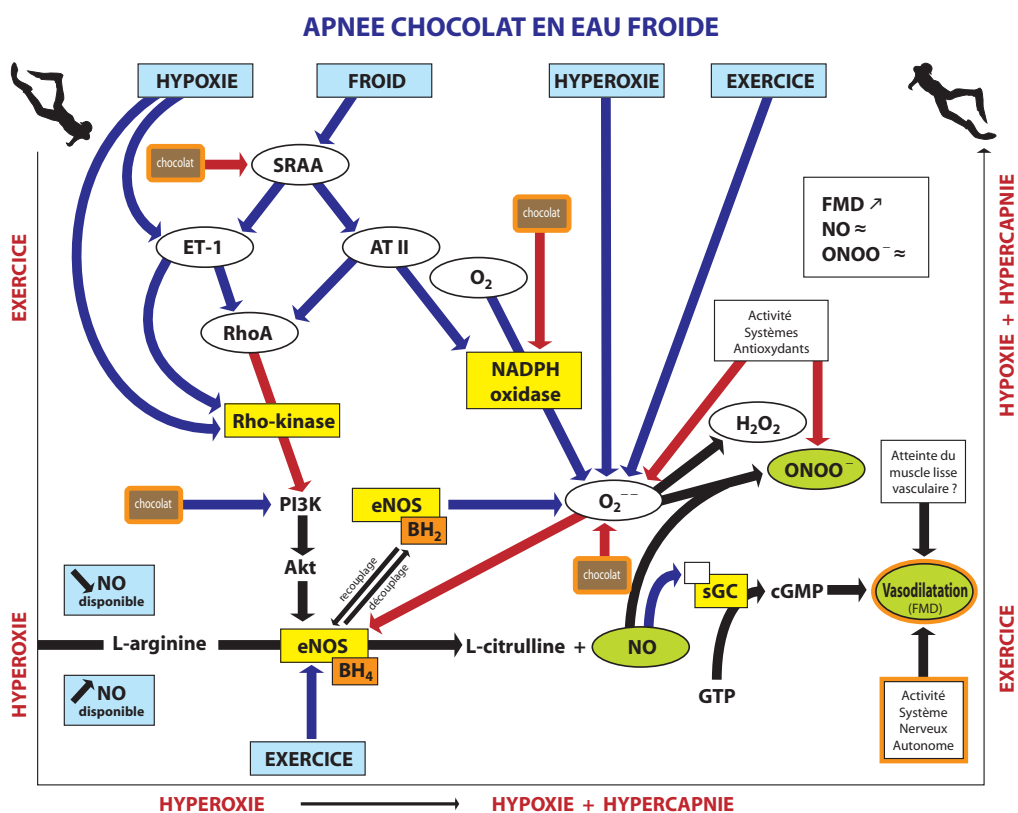
FIGURE 20 - MECANISMES SOUS-JACENTS A LA PLONGEE EN APNEE APRES INGESTION DE CHOCOLAT NOIR.
