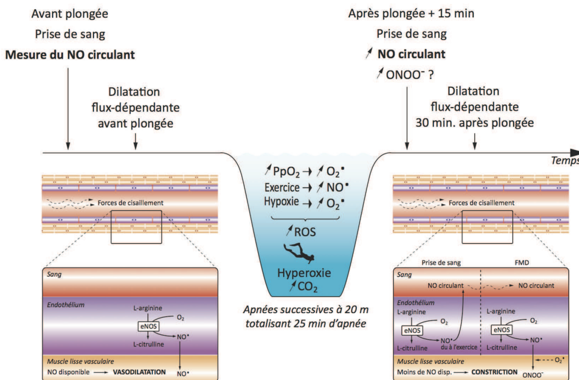
FIGURE 11 – RESUME DES MECANISMES PROPOSES DURANT LA PLONGEE EN APNEE.
