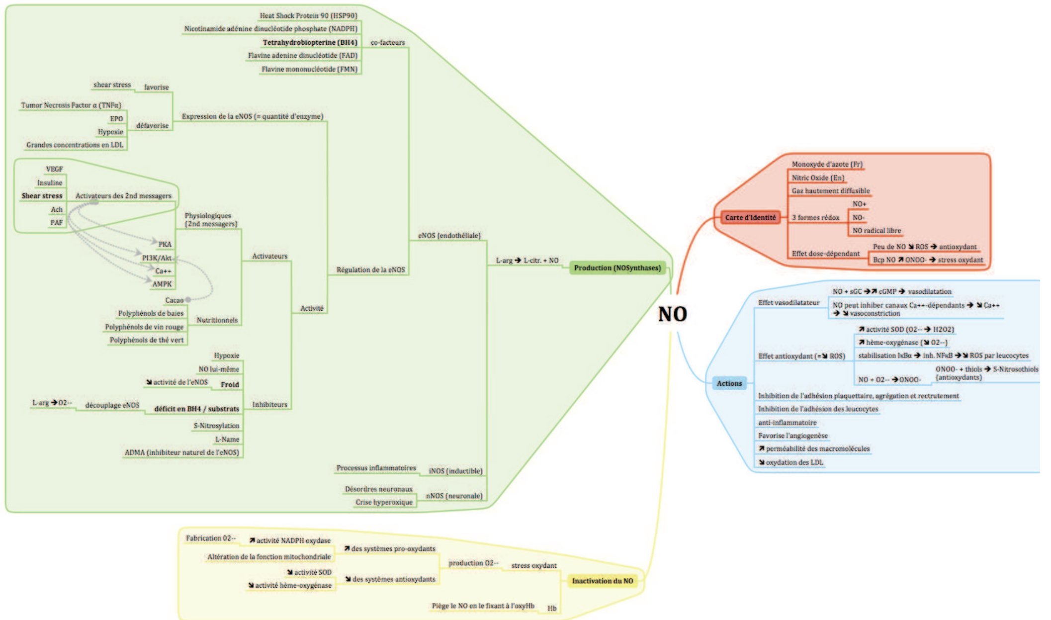
FIGURE 3 – CARTE MENTALE REPRESENTANT LA CARTE D'IDENTITE DU MONOXYDE D'AZOTE, SA PRODUCTION, SON INACTIVATION ET SES ACTIONS.
