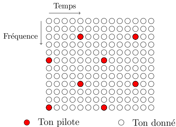
FIGURE 2.16 – Répartition des tons pilotes dans une communication descendante du standard LTE avec 1 antenne.
