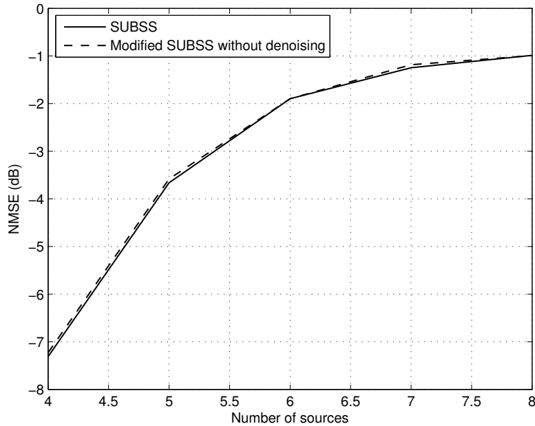
FIGURE 4.9 – Comparaison des performances entre les algorithmes SUBSS et SUBSS modifié sans débruitage pour un SNR=10dB : l’erreur quadratique moyenne normalisée en fonction du nombre de sources.
