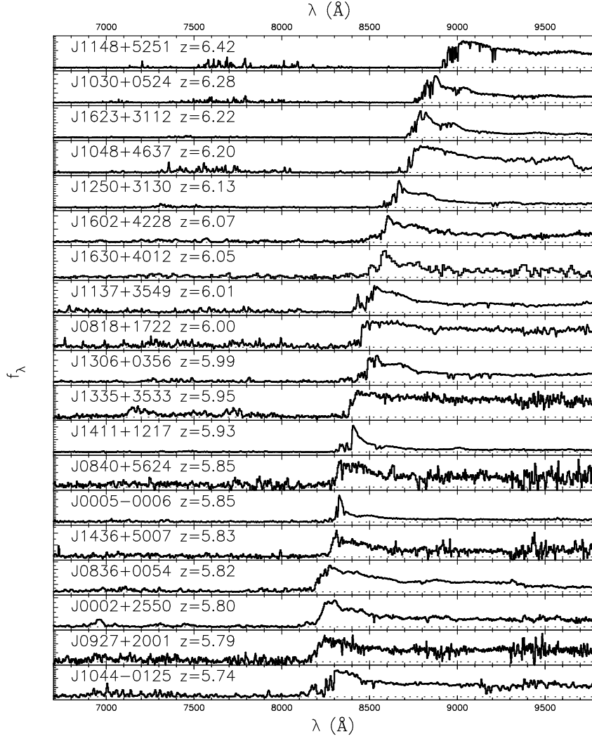
Figure 8.1 – Intensité en fonction de la longueur d’onde mesurée pour 19 quasars. On voit que par exemple pour le quasar à z = 6.22 , l’intensité tombe à zéro pour \lambda \lesssim \lambda_{\text{Ly}\alpha}(1+z) = 8777 \text{ \AA} , ce qui n’est pas le cas pour le quasar à z = 5.79 , où il n’y a que des raies d’absorption pour \lambda \lesssim \lambda_{\text{Ly}\alpha}(1+z) = 8254 \text{ \AA} . Entre les deux, la tendance n’est pas monotone : des raies d’absorption continuent à apparaître sur des spectres de quasars plus lointains que d’autres pour lesquels l’intensité est strictement nulle. Cela indique un certain niveau d’inhomogénéité de la Réionisation. Figure de [Fan et al., 2006b].
