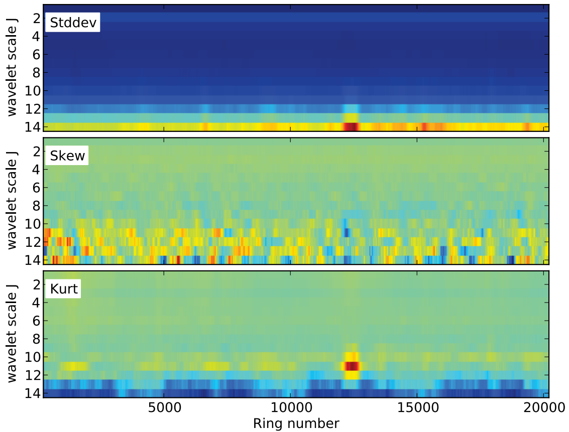
Figure 3.12 – Décomposition en ondelettes des TOIs de bruit du bolomètre 10_143_5, pour chaque ring de la mission nominale. Les hautes fréquences sont en haut, et les basses fréquences en bas.
