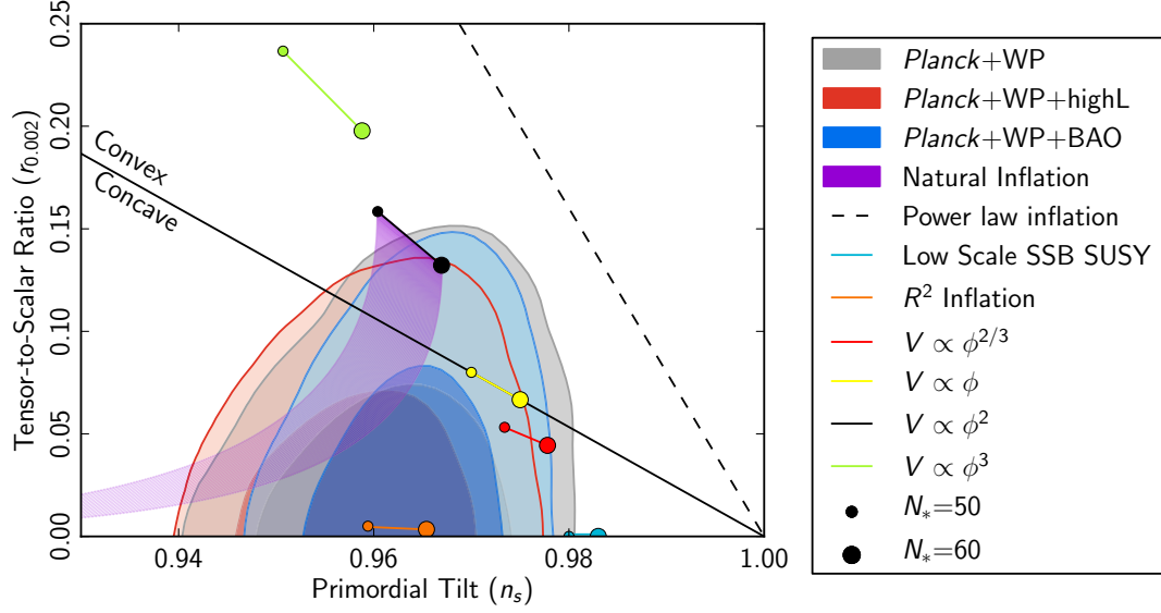
Figure 6.7 – Dans l'espace n_s - r , niveau de confiance à 68% et 95% de trois ensembles de données, ainsi que les prédictions théoriques pour différents modèles d'inflation. Figure de [Planck Collaboration, 2013i].
