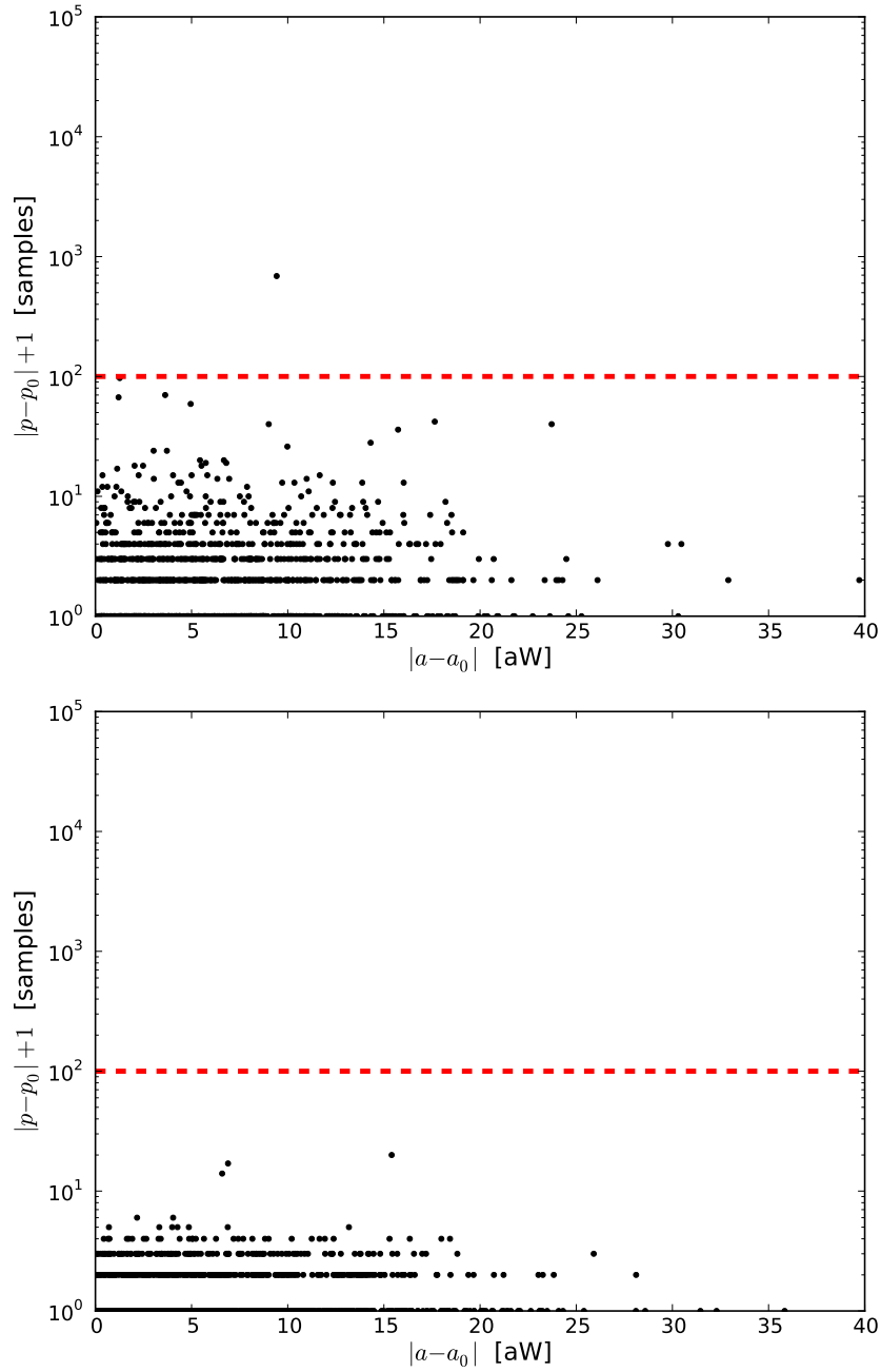
Figure 2.13 – Erreurs sur la reconstruction de sauts simulés dans le plan (a, \alpha) , pour un bolomètre à 143 GHz, à 1\sigma (haut) et 2\sigma (bas). Dans les deux cas, 99.9% des 1001 sauts sont retrouvés (et montrés sur cette figure).
