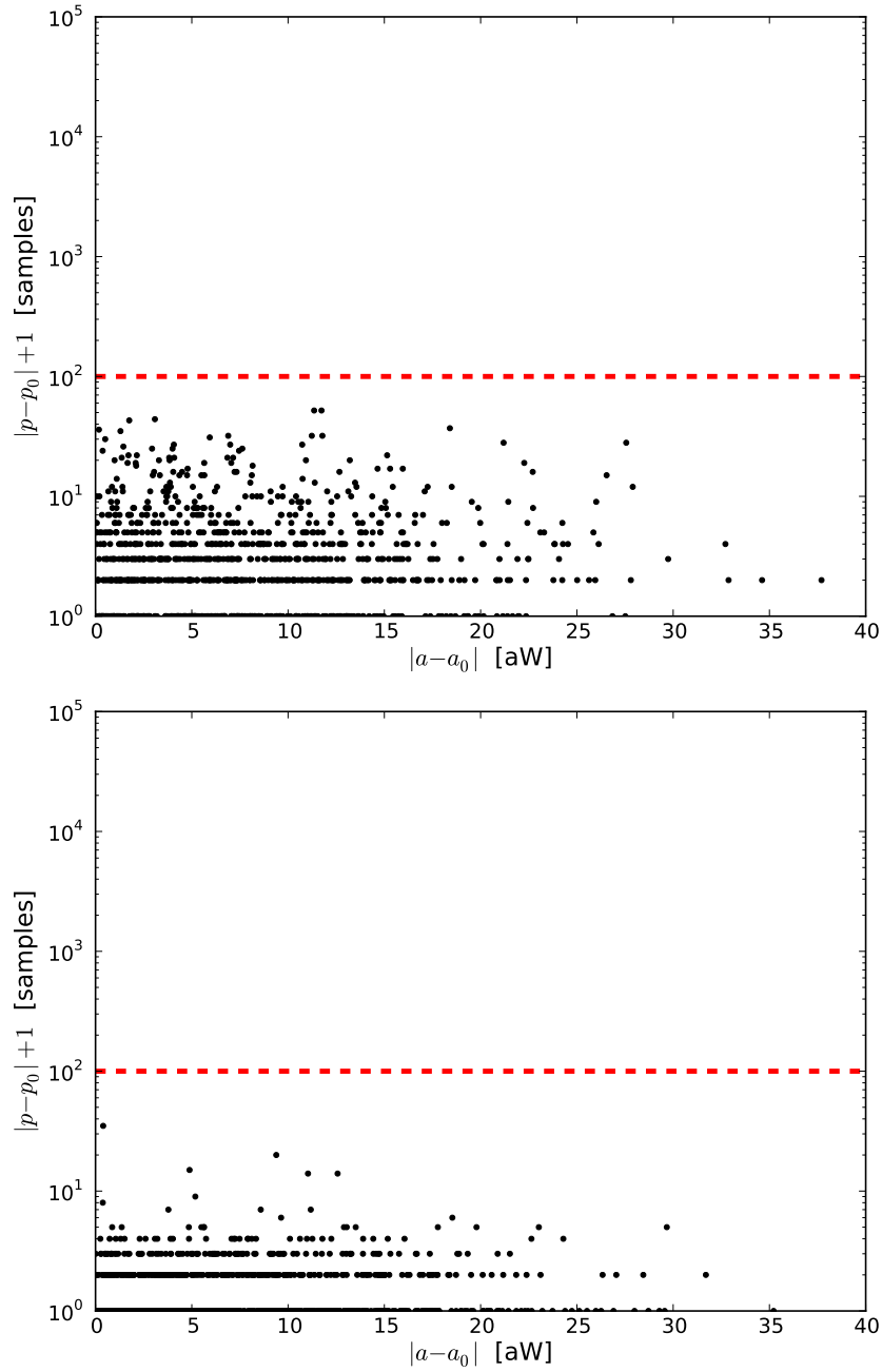
Figure 2.14 – Erreurs sur la reconstruction de sauts simulés dans le plan (a, \alpha) , pour un bolomètre à 353 GHz, à 1\sigma (haut) et 2\sigma (bas). Dans les deux cas, 99.9% des 1001 sauts sont retrouvés (et montrés sur cette figure).
