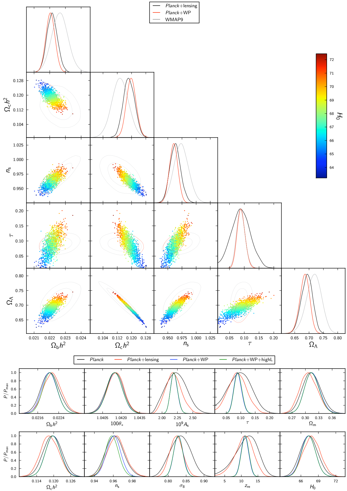
Figure 6.4 – Haut : Comparaison des paramètres de base du modèle \Lambda CDM pour Planck + lentille, Planck + WMAP, et pour WMAP seul. Les contours à 2D sont à 68 et 95%. Bas : illustration de la cohérence des données sur les paramètres de base pour plusieurs combinaisons. Figures de [Planck Collaboration, 2013f].
