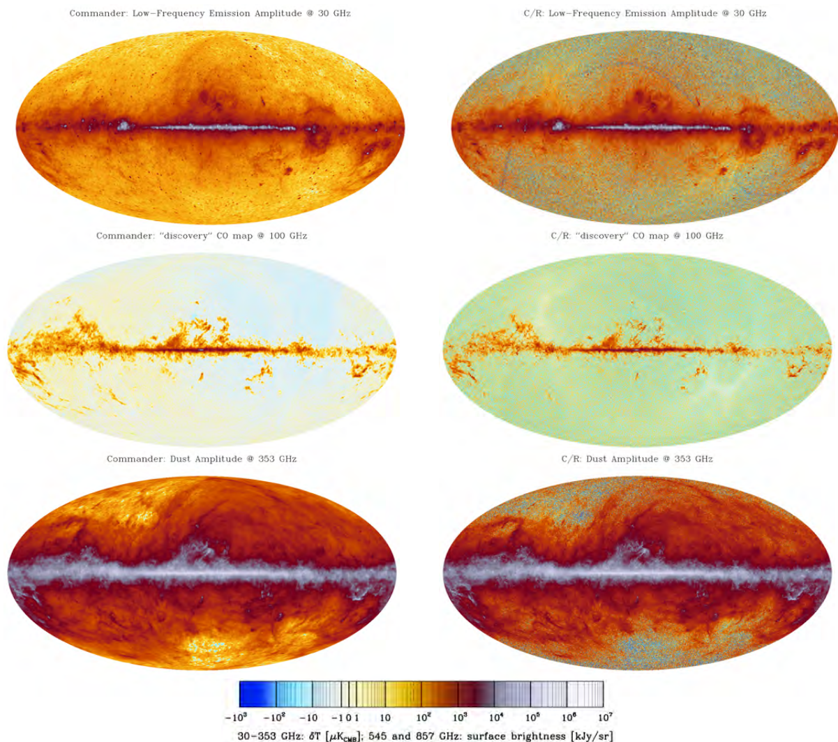
Figure 5.4 – Quelques avant-plans galactiques retrouvés par la séparation de composantes de Commander (colonne de gauche, résolution de \approx 1^\circ ) et Commander-Ruler (colonne de droite, résolution de \approx 7' ). Haut : Avant-plans de basse fréquence (synchrotron, rayonnement de freinage, et émission anormale) à 30 GHz. Milieu : Monoxyde de carbone (obtenu par la méthode du rapport d'émission des raies) à 100 GHz. Bas : Avant-plans à haute fréquence (émission thermique de la poussière et CIB).
