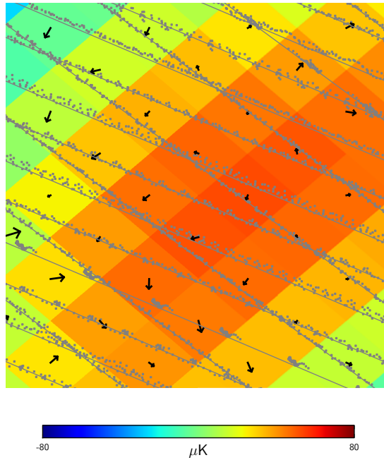
Figure 4.18 – Illustration de la pixélisation du CMB (simulation convoluée par une gaussienne de 7 minutes d'arc de largeur à mi-hauteur et pixélisée à n_{side} = 2048 ) et de l'échantillonnage des TOI le long des rings (en gris). Les flèches représentent la déflexion induite par la non-uniformité de la couverture et le gradient du signal. Figure de [Planck-HFI Collaboration, 2013b]
