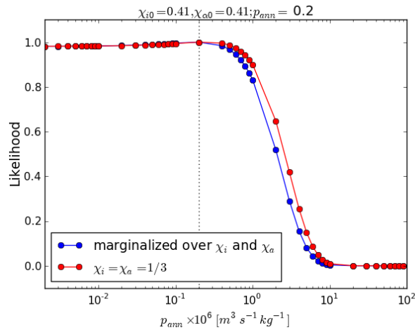
Figure 7.14 – Reconstruction de p_{\text{ann}} en marginalisant sur les fractions \chi_{i,\alpha,h}^0 (bleu), ou avec l’hypothèse 1/3 (rouge).
