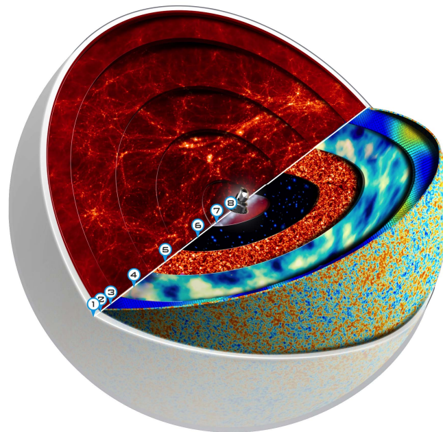
Notre Univers observable : d'un côté les simulations de l'évolution des structures ; de l'autre, les observations réalisées par Planck (8) : notre Galaxie (7), amas de galaxies (6), poussières extra-galactiques (5), distribution de matière (4), Réionisation (3), CMB (2), big-bang (1). Crédit : ESA-Collaboration Planck, S. Colombi, Canopée.
