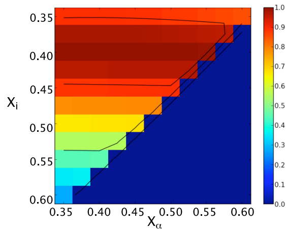
Figure 7.9 – Vraisemblance dans la tranche p_{\text{ann}} = p_{\text{ann,max}} . Les isocourbes sont \mathcal{L}_i = [5\%, 50\%, 95\%]
