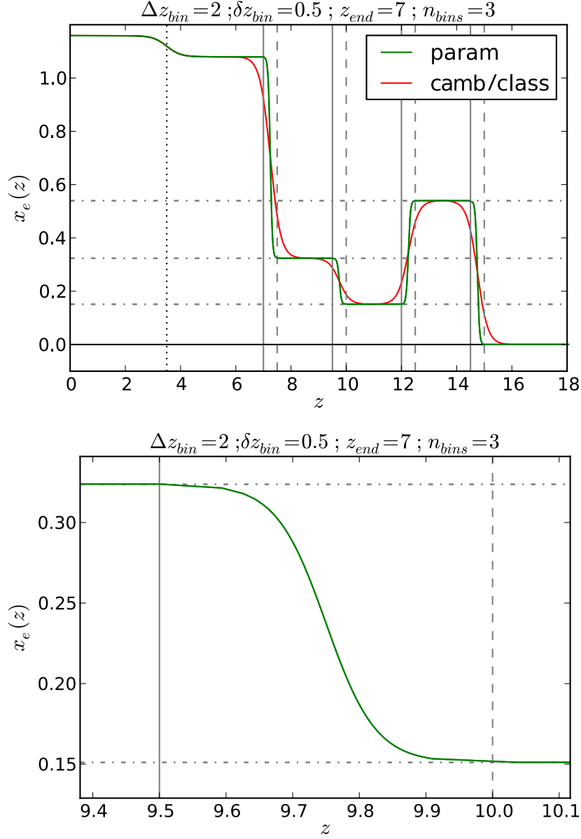
Figure 8.9 – Haut : Illustration de notre choix de binning pour la Réionisation (vert) comparé à ce qui est implémenté dans CLASS (rouge). Le début de la Réionisation a lieu à z_{début} = z_{fin} + n_{bins} \times (\Delta z_{bin} + \delta z_{bin}) . Bas : Détail d’une transition en tangente hyperbolique. Dans notre paramétrisation, x_e(z) est exactement constant hors de la transition.
