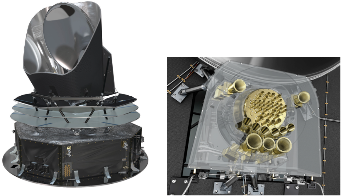
Figure 1.5 – Le satellite Planck et son plan focal. Gauche : Vue d'artiste du satellite. On voit de haut en bas : le télescope et son baffle, les trois ailettes de refroidissement, le module de service et les panneaux solaires (de dessous). Droite : Vue d'artiste du plan focal. Les cornets internes correspondent à l'instrument HFI, les cornets externes sont ceux de LFI. Crédits : ESA-Medialab.
