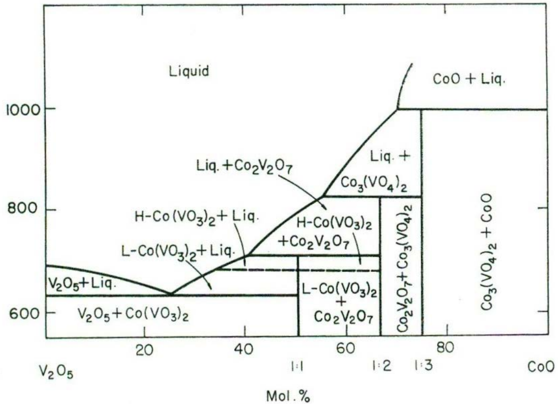
Figure 6 : Diagramme de phase du système \text{CoO-V}_2\text{O}_5 par C. Brisi [19] mettant en évidence deux phases de \text{CoV}_2\text{O}_6 en fonction de la température de synthèse.
