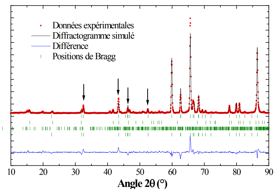
Figure 26 : Diffractogramme de neutrons de \alpha \text{CoV}_2\text{O}_6 enregistré à 5 K sous un champ de 5 T et son affinement structural et magnétique constitué de trois phases magnétiques. Les flèches indiquent les pics principaux apparaissant lors du passage de 2,5 à 5 T et correspondant à la phase ferromagnétique.
