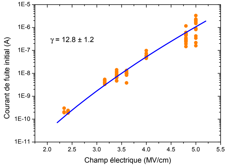
FIGURE 4.8 – Modèle de conduction de Poole-Frenkel appliqué au courant de fuite initial du diélectrique sous différents champs électriques. Une valeur de 12,8 \pm 1,2 (\text{cm/MV})^{0.5} est extraite de la modélisation pour \gamma . [S=50 nm, W=50 nm, L=2 mm, T=125°C]
