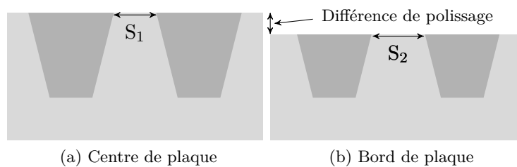
FIGURE 5.14 – Modification de l'espacement intermétallique par l'étape de polissage chimico-mécanique. Le sur-polissage constaté en bord de plaque amène à un espacement intermétallique plus important.
