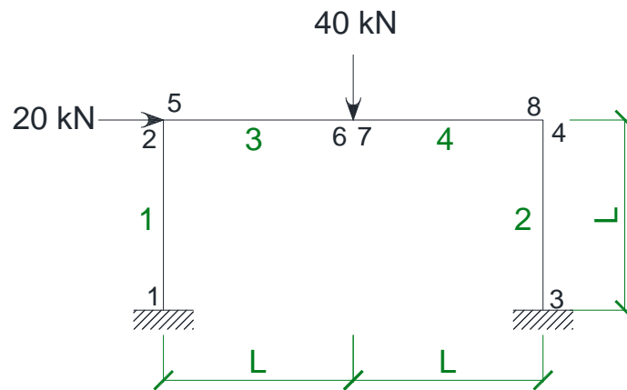
Figure 3.40. Numérotation des éléments structurels.
