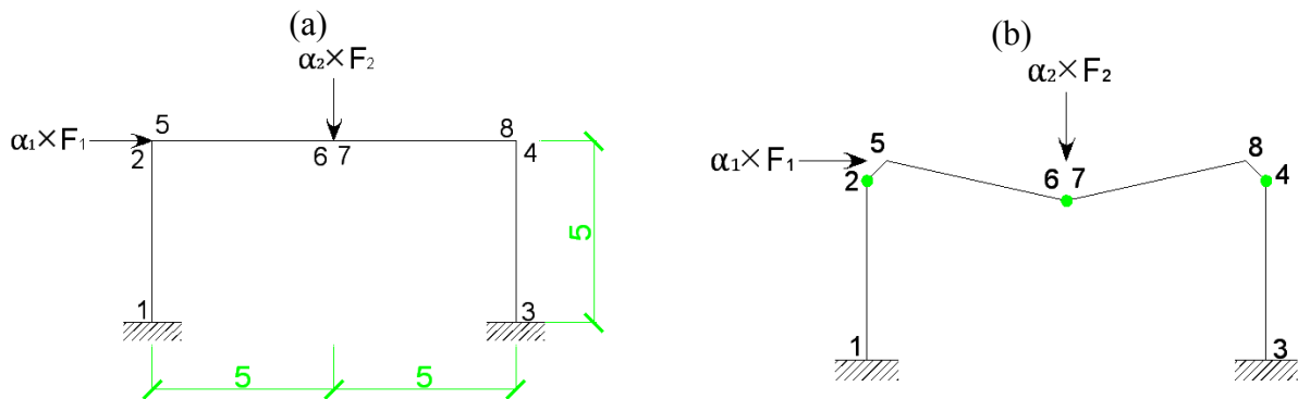
Figure 4.10. (a) coefficients de charge appliqués, (b) mécanisme de défaillance le plus probable. Les Figures 4.11a et 4.11b représentent les variations des indices de robustesse I_{r,1} et I_{r,2} avec les valeurs des coefficients \alpha_1 et \alpha_2 . On remarque que \alpha_2 est le coefficient qui influence le plus l'indice de robustesse. En d'autres termes, plus la charge verticale est élevée, plus l'indice de robustesse est faible.
