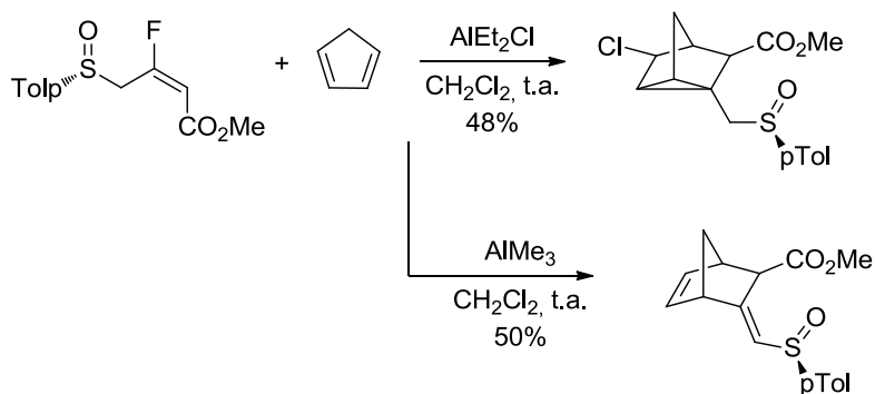
(Esquema 6)
