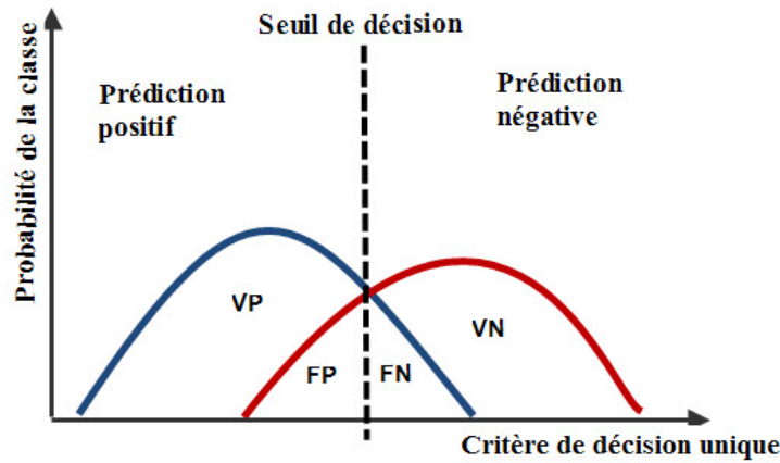
FIGURE 3.9 – Les quatre états possibles lors de la prédiction d'un modèle de classification binaire. Le seuil de décision choisi détermine les états correspondants aux VP, FN, FP, et VN.
