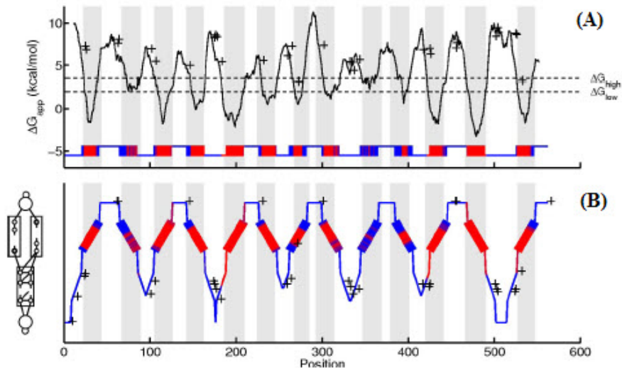
FIGURE 2.11 – Topologie d'une protéine en utilisant TOPPRED (figure (A)) et SCAMPI (figure (B)) [Bernsel et al., 2008].
