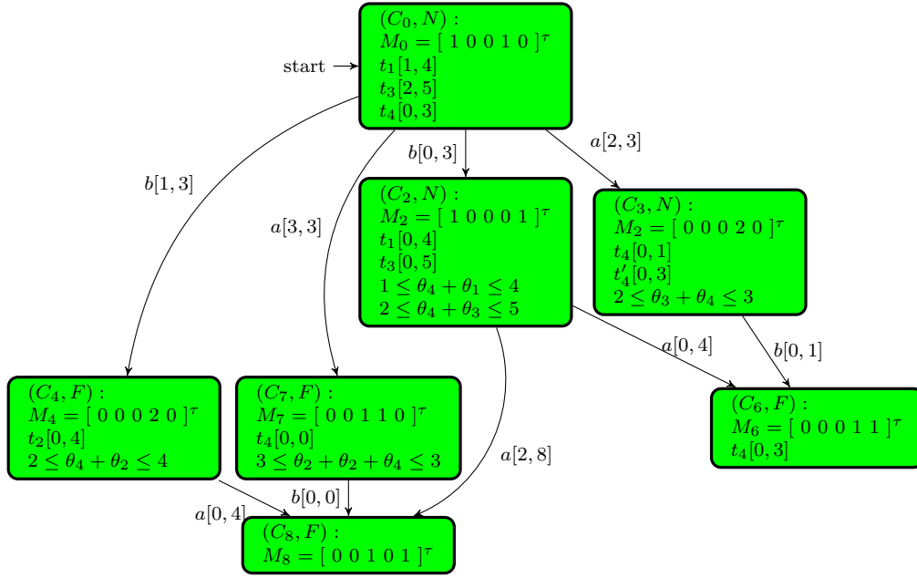
(e) Step 5
