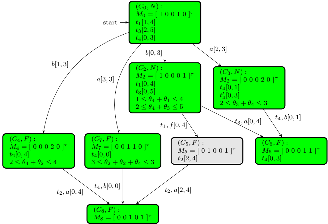
(d) Step 4
