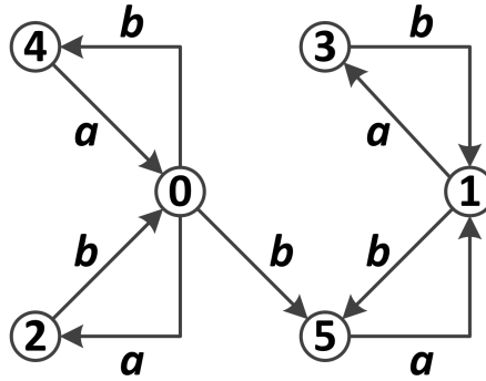
(b) FM^2 -graph
