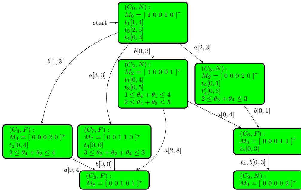
(f) Step 6
