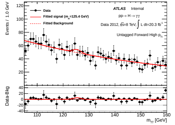
(d) Forward high p_{Tt} 2012
