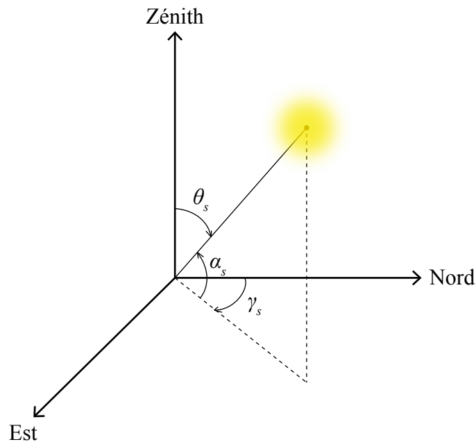
FIGURE 3.4 – Position du soleil dans les coordonnées horizontales du lieu terrestre considéré.
