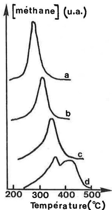
Figure B.43 : Spectres du méthane formé par T.P.R. du catalyseur Fe/Al 2 O 3 après réaction H 2 + CO à 200°C (a), 225°C (b), 250°C (c) et 275°C (d) pendant 20 heures.
