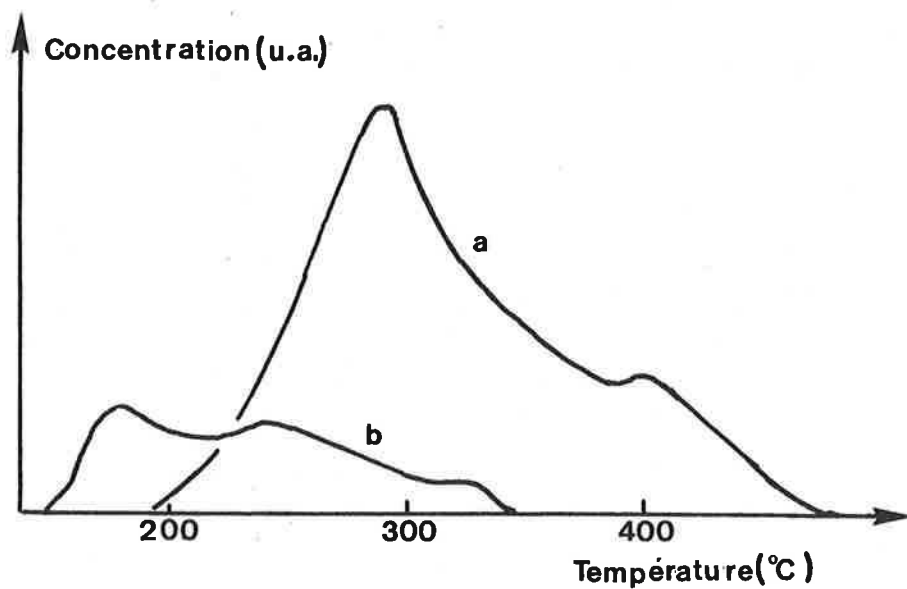
Figure B.45 : Spectres de l'eau (a) et du méthane (b) formés par T.P.R. du catalyseur Fe/Al 2 O 3 après réaction H 2 + CO 2 à 225°C pendant une heure.
