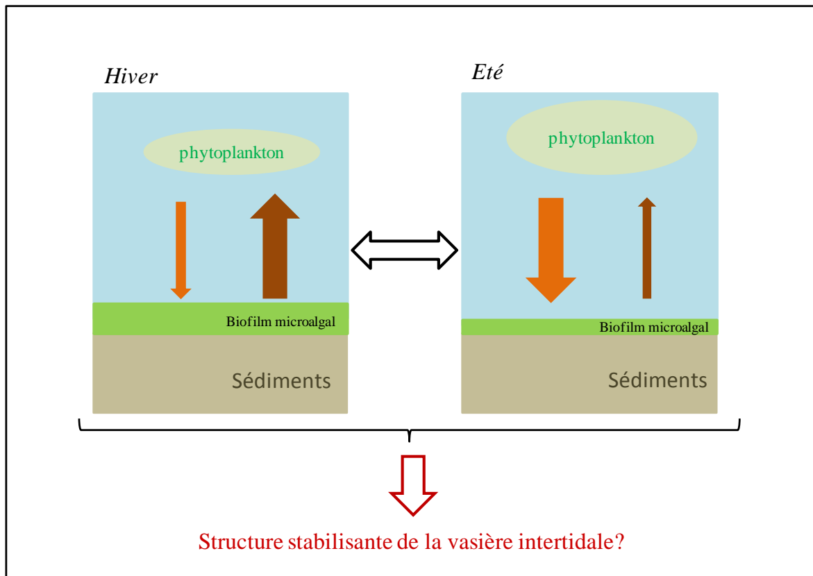
Figure VI-2 : Schéma bilan. Hypothèse d'une saisonnalité de la remise en suspension apportant de la stabilité à l'écosystème vaseuse intertidale.
