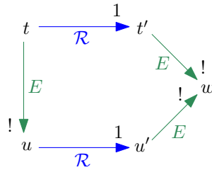
FIGURE 3.9 — Cohérence entre \mathcal{R} et E .
