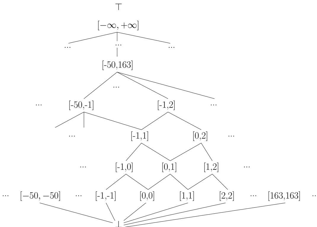
FIGURE 2.16 — Le treillis des intervalles est atomique.
