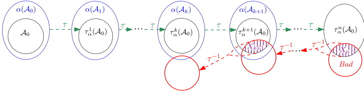
(b) Faux contre-exemple : l'approximation doit être raffinée pour ne plus accepter aucun terme de X_{k+1} .
