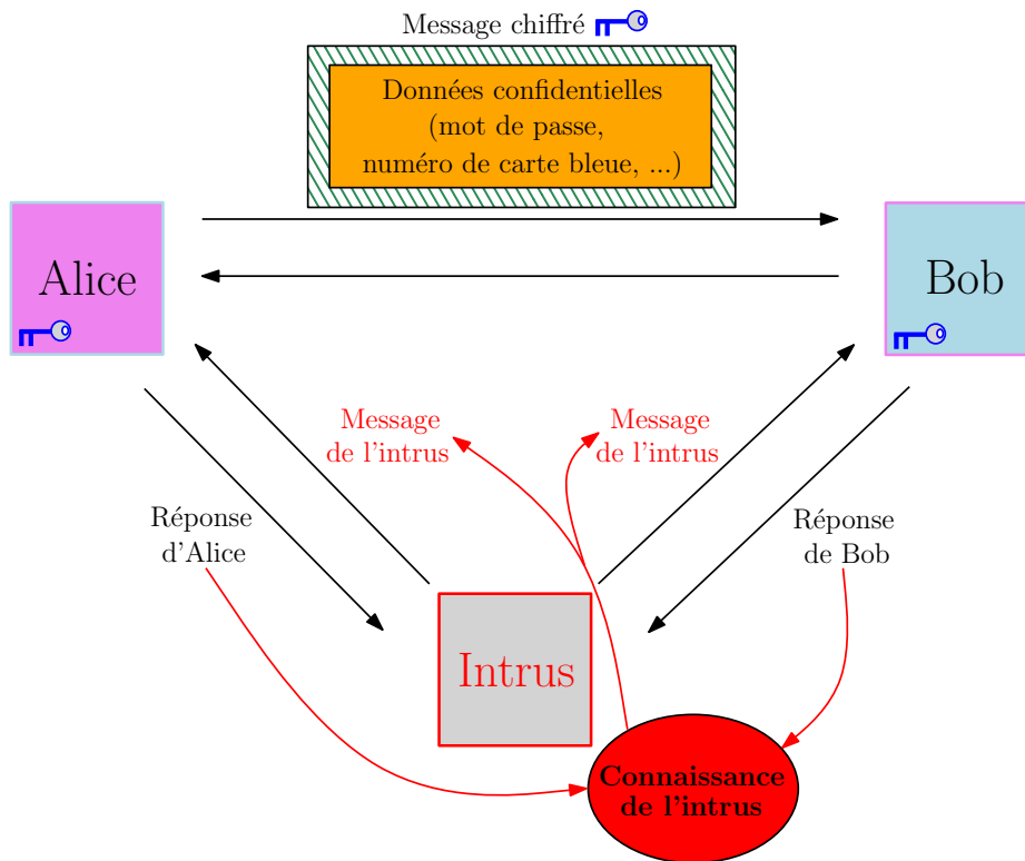
FIGURE 1.4 — Un intrus malveillant peut construire une infinité de messages différents pour tenter de récupérer des données confidentielles.
