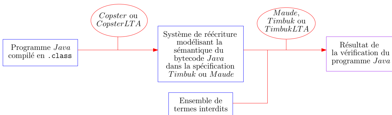
FIGURE 6.1 — Vérification d'un programme Java grâce à Copster et Timbuk.
