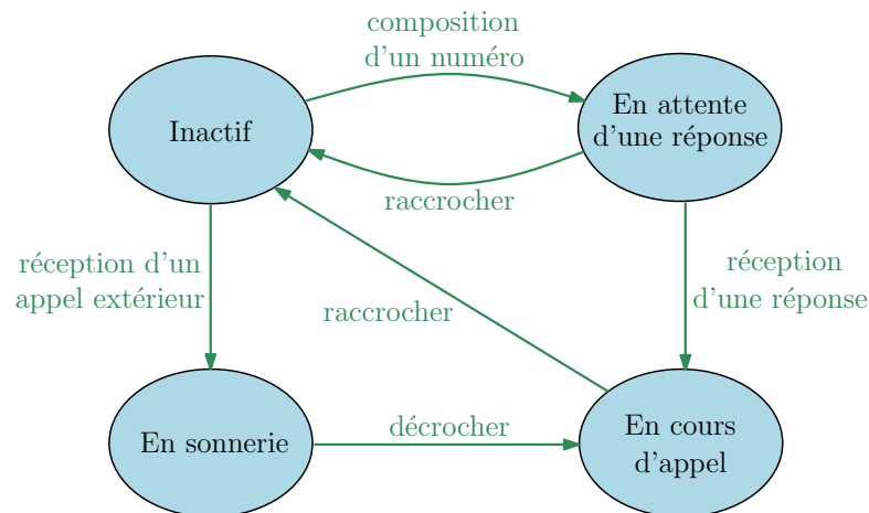
FIGURE 1.2 — Modélisation simplifiée du fonctionnement d'un téléphone sous forme de système état-transition.
