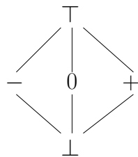
FIGURE 2.15 — Le treillis des signes.
