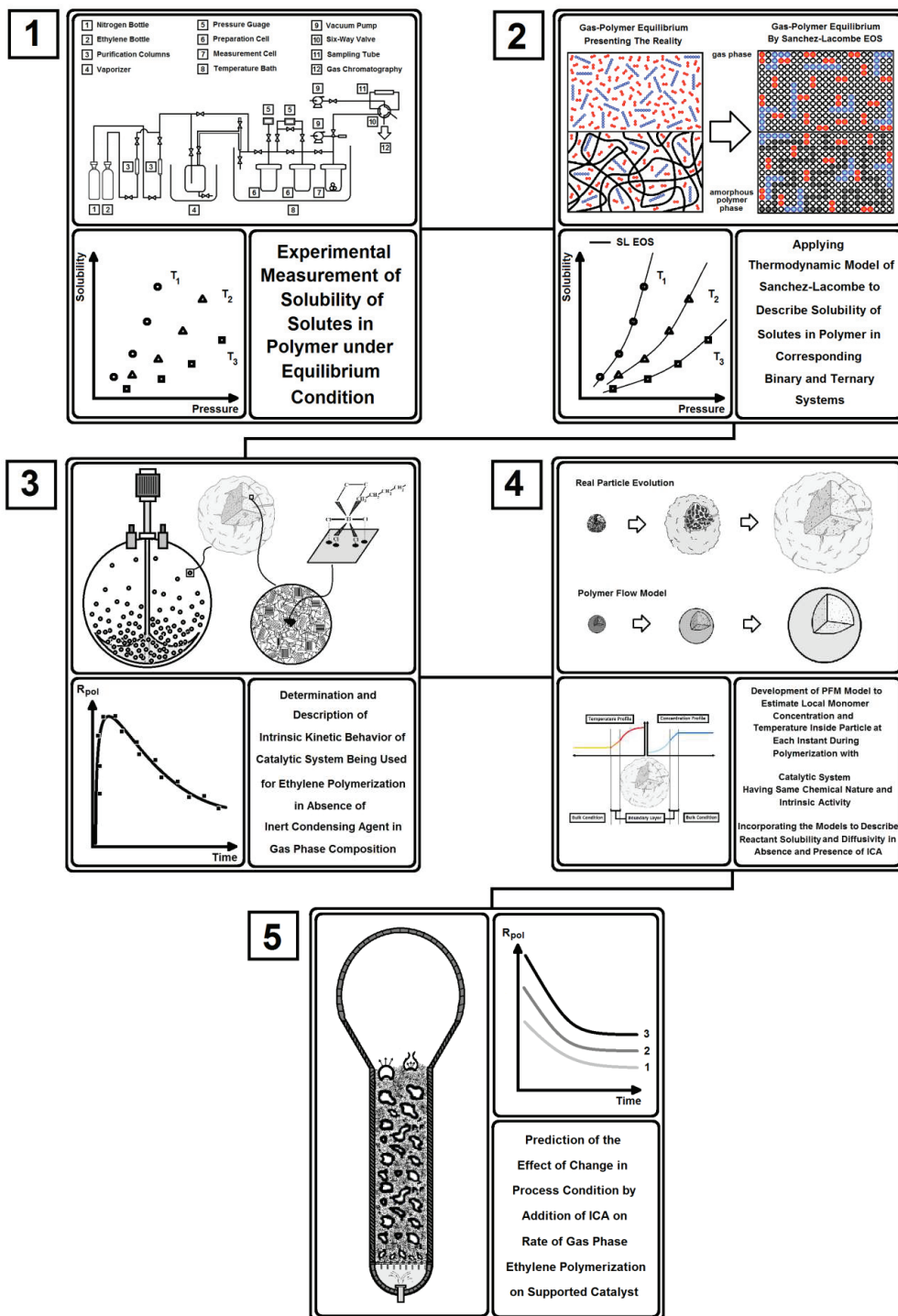
Figure 8. Vue d'ensemble de l'approche phénoménologique désignée pour prédire l'effet du changement des conditions du procédé par addition d'un agent condensant inerte sur la vitesse de polymérisation de l'éthylène en phase gaz.
