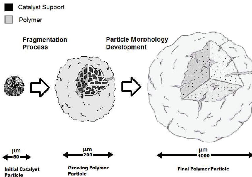
Figure 2. Représentation schématique de l'évolution d'une particule pendant la polymérisation de l'éthylène en phase gaz sur catalyseur supporté.
