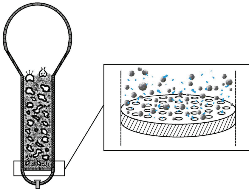
Figure 1. Représentation schématique du procédé de vaporisation de la portion liquéfiée du flux d'alimentation durant le mode d'opération condensé.
