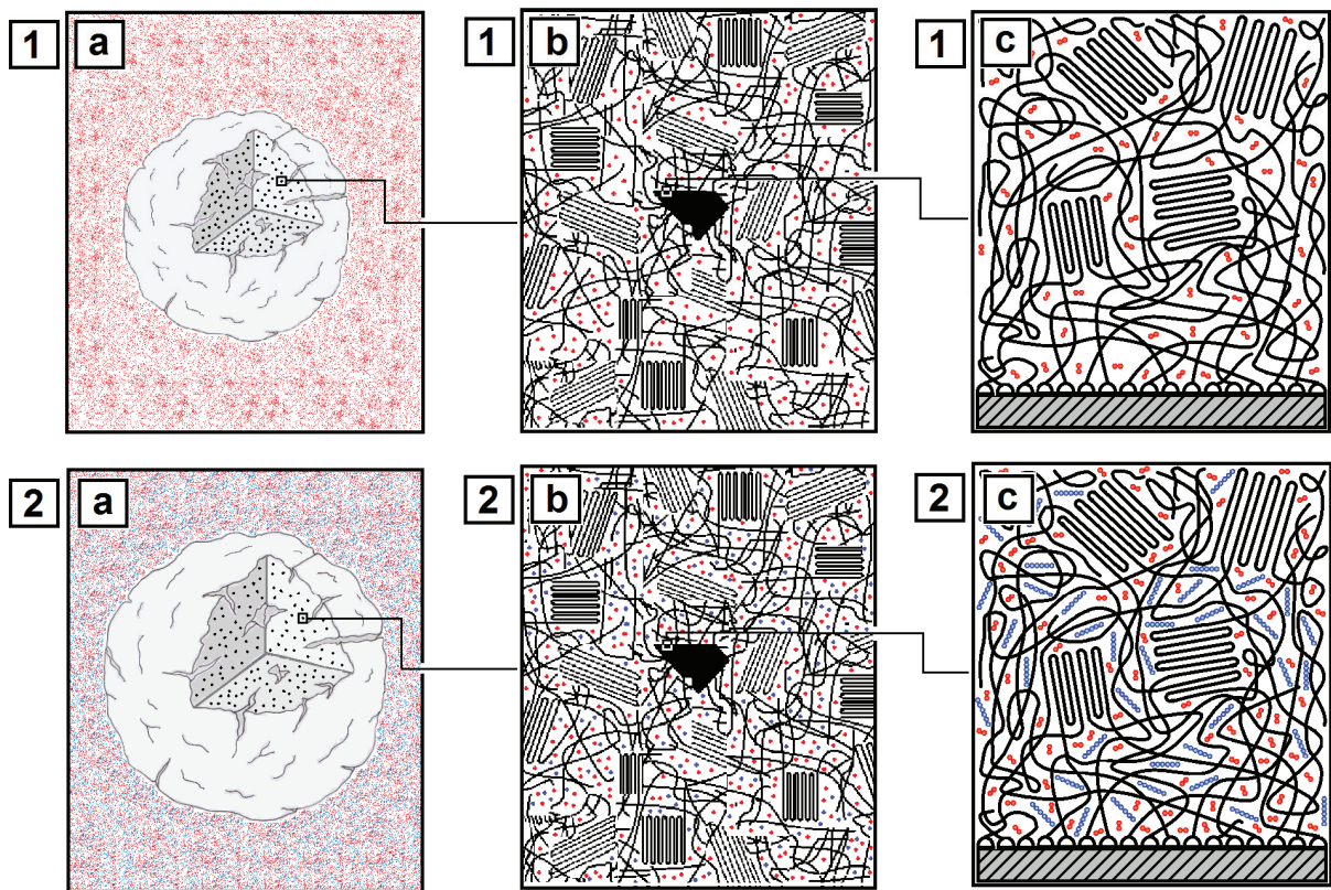
Figure 4. Représentation schématique du système binaire éthylène-polyéthylène (1) et du système ternaire éthylène-hexane-polyéthylène (2) à l'échelle correspondant (a) à une particule, (b) un fragment de catalyseur encapsulé par du polyéthylène semi-cristallin, et (c) des chaînes de polymère initiées à partir de sites actifs immobilisés à la surface d'un fragment du catalyseur.
