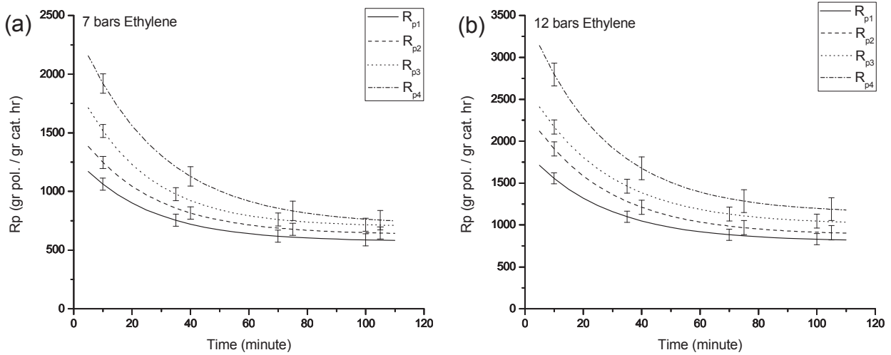
Figure 6. Vitesse instantanée de la polymérisation de l'éthylène à 80 °C en présence de 0.0, 0.3, 0.6, et 0.8 bar de pression partielle d'hexane dans l'environnement du réacteur correspondant à R_{p1} , R_{p2} , R_{p3} , et R_{p4} avec une pression partielle d'éthylène dans l'environnement du réacteur égale à (a)7 et (b)12 bars.
