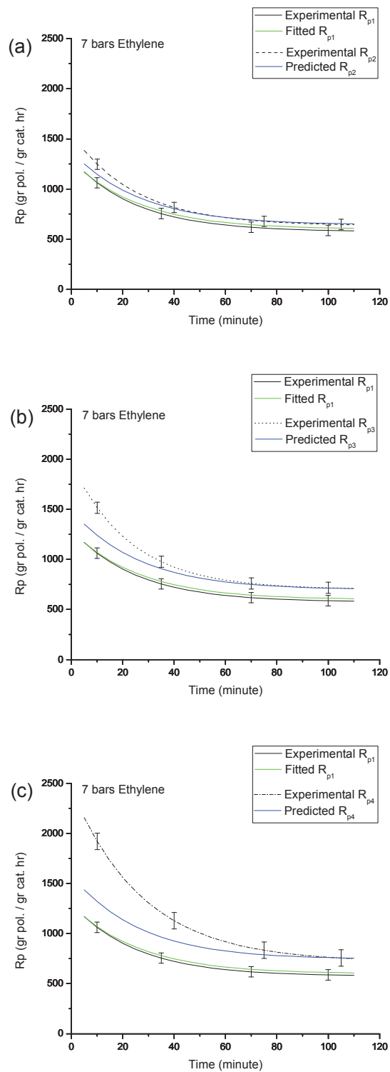
Figure 9. Evaluation de la capacité de prédiction du modèle développée pour l'effet de la présence d'hexane dans la composition de la phase gaz sur la vitesse instantanée de la polymérisation de l'éthylène en phase gaz pour une pression partielle d'éthylène de 7 bars.
