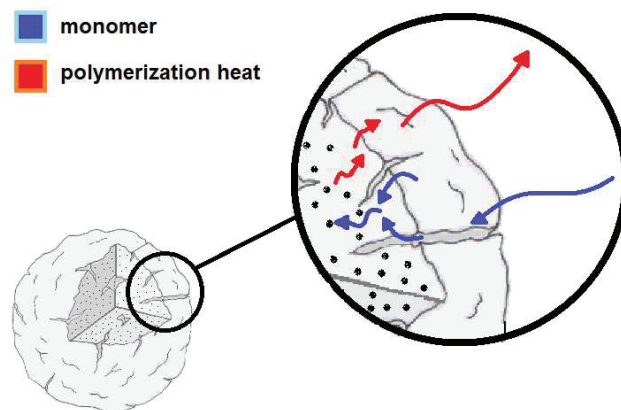
Figure 3. Représentation conceptuelle de la sorption et de la diffusion de l'éthylène dans le polymère produit, et de l'évacuation de la chaleur associée à la polymérisation par un mécanisme de convection à partir d'une seule particule de polymère pendant la polymérisation de l'éthylène en phase gaz sur catalyseur supporté.
