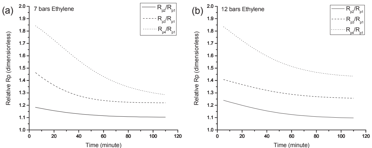
Figure 7. La vitesse instantanée de polymérisation en présence d'hexane moyennée, normalisée avec celle réalisée sans hexane avec une pression partielle d'éthylène dans le réacteur égale à (a)7 et (b)12 bars.
