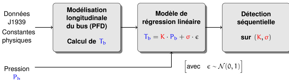
FIGURE 4.8 – Stratégie séquentielle de détection en 3 étapes pour la surveillance du système de freinage.
