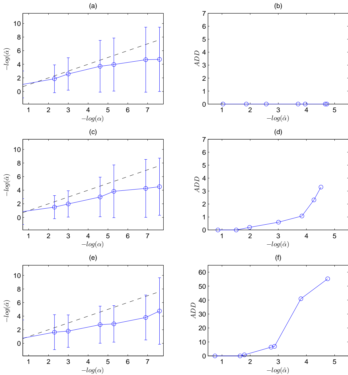
FIGURE 5.13 – Évaluation graphique du détecteur proposé en fonction des taux de fausses alarmes et des délais moyens à la détection. Les figures (a,c,e) représentent les taux de fausses alarmes expérimentaux \hat{\alpha} en fonction des taux théoriques \alpha . Et les figures (b,d,f) représentent les délais moyens de détection ADD en fonction des taux de fausses alarmes expérimentaux \hat{\alpha} .
