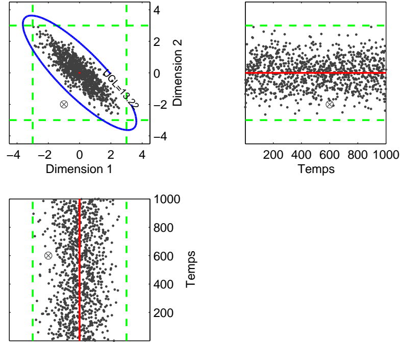
FIGURE 3.5 – Intérêt d’une approche bvariée pour des données en dimension deux. Le point \otimes sort de la région dite « sous contrôle » (ellipse en bleu) mais reste dans l’intervalle de confiance sur chaque dimension.
