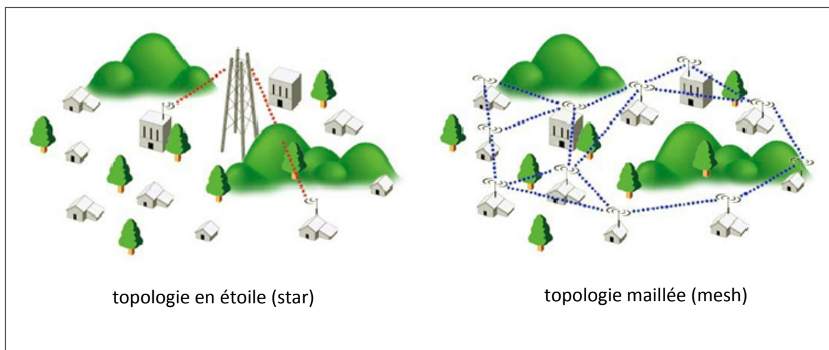
Figure 3 : Topologies réseau 802.16
