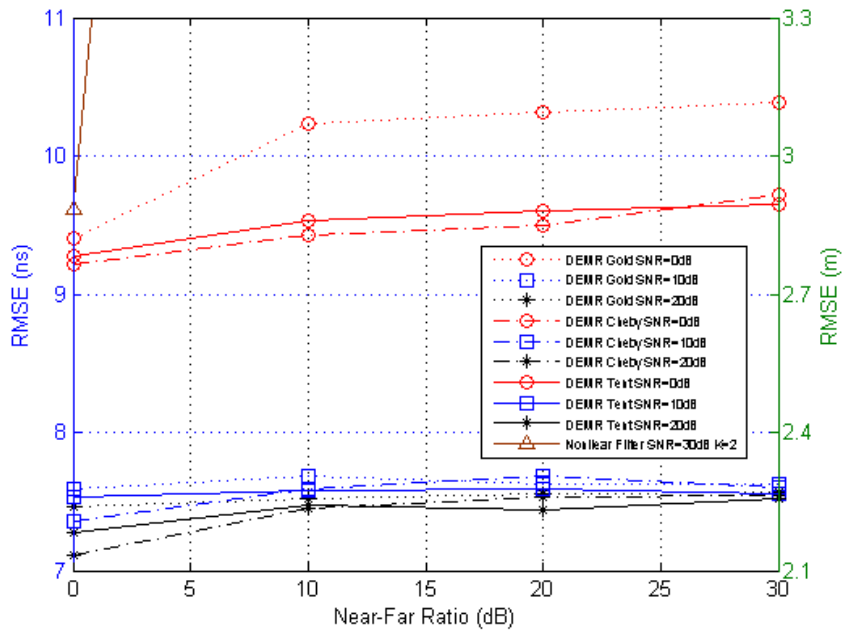
Figure R.15: RMSE en fonction du rapport proche-lointain pour différentes valeurs de SNR avec M = 100 , N = 31 , et K = 10 dans le canal CM1.
