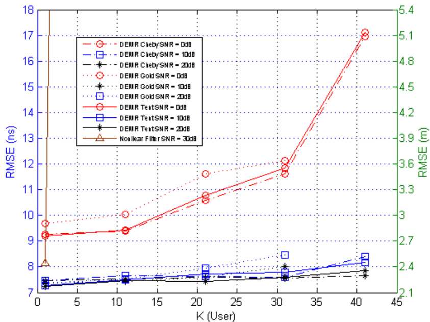
Figure R.16: RMSE en fonction du K pour différentes valeurs de SNR avec M = 100 , N = 31 , and near-far ratio is 10 dB dans le canal CM1.
