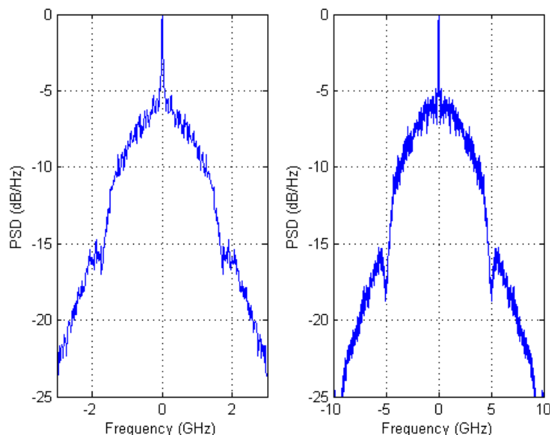
Figure R.6: Densité spectrale de puissance de l'heure exacte échelle des formes d'onde de Lorenz dans la longueur T_c = 31ns .
