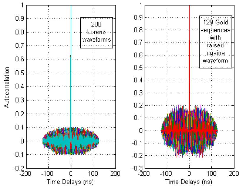
Figure R.8: Fonction d'autocorrélation de l'impulsion Lorenz sélectionné et élevé impulsion de cosinus avec des séquences Gold en T_s = 127ns .
