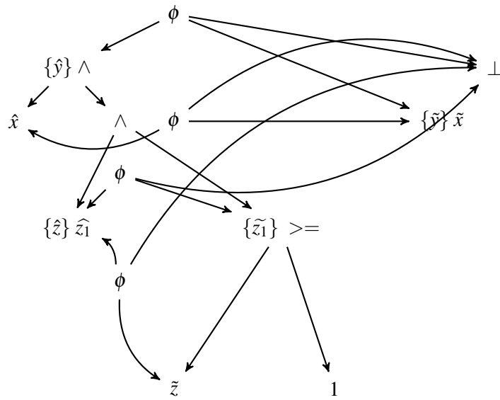
Fig. 6.18 The graph of y := x when (z \geq 1)
