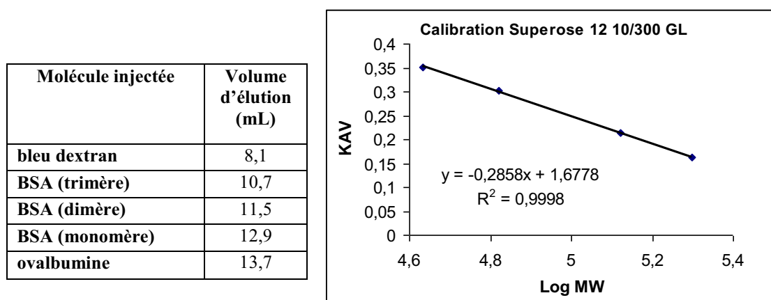
Figure 2.7 : Calibration de la colonne Superose 12 10/300 GL
