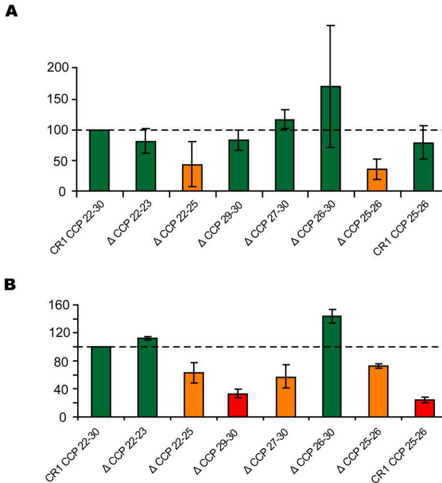
Figure 4.16 : Fixation de C1q sur les différentes constructions de CR1 CCP 22-30
