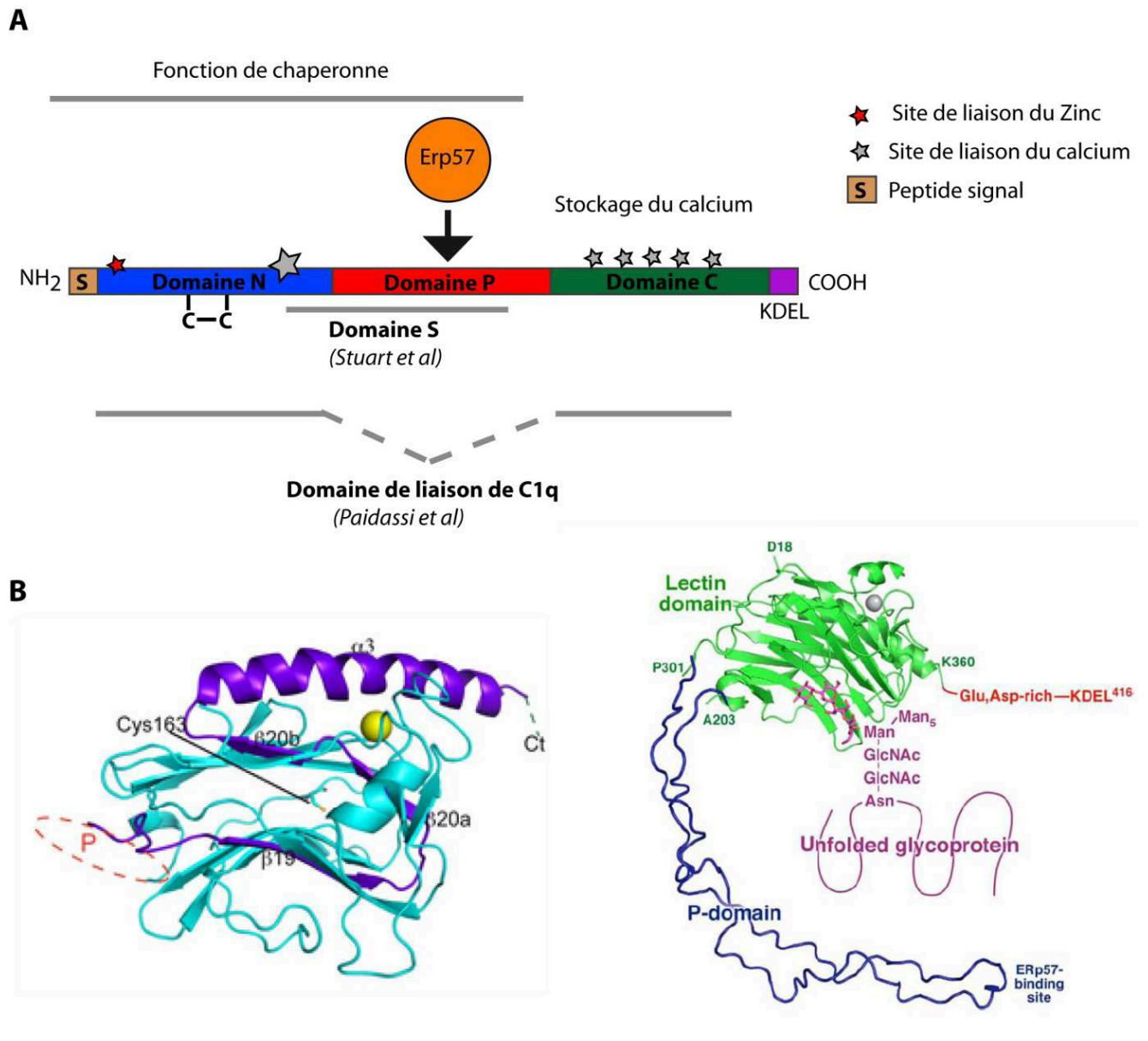
Figure 1.6 : Organisation et structure de la calréticuline
