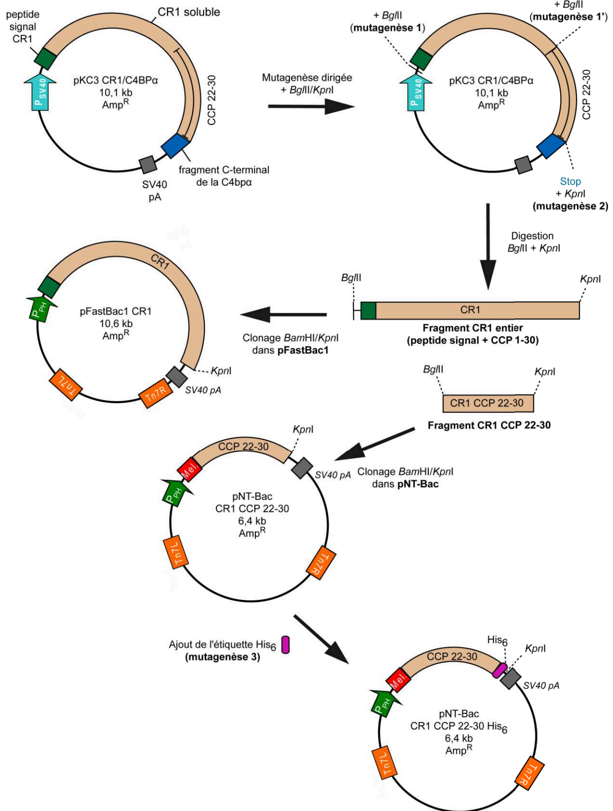
Figure 2.3 : Schéma de la construction des vecteurs pFastBac1 CR1 et pNT-Bac CR1 CCP 22-30 His 6 Amp R : résistance à l'ampicilline ; P SV40 : promoteur du virus Simien 40 ; pA : site de polyadénylation ; P PH : promoteur polyhedrine ; SV40 pA : signal de polyadénylation du virus Simien 40 ; Mel. : peptide signal de la melittine ; His 6 : étiquette poly-histidine.
