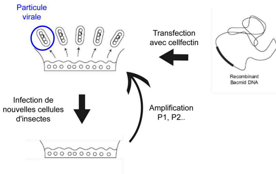
Figure 2.9 : Représentation schématique des étapes de la transfection du bacmide et de l'amplification virale (Adapté du manuel d'utilisateur du système Bac-To-Bac)
