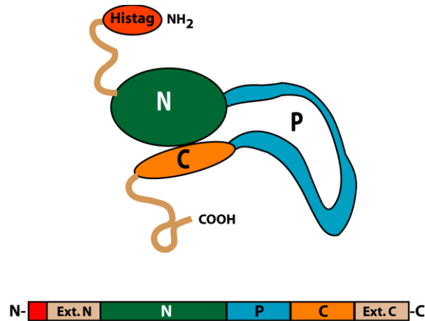
Figure 3.1 : Représentation schématique de la TcCRT issue de la construction d'A. Ferreira
