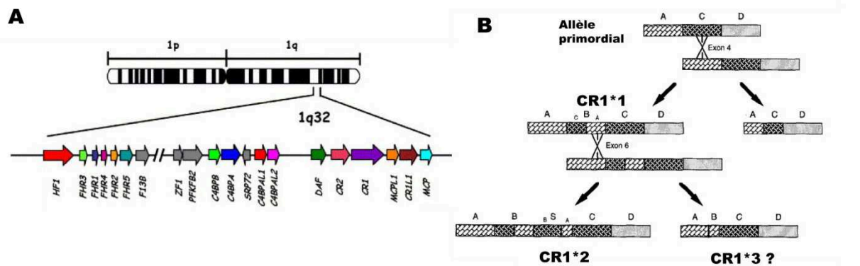
Figure 1.10 : Organisation génétique de CR1
