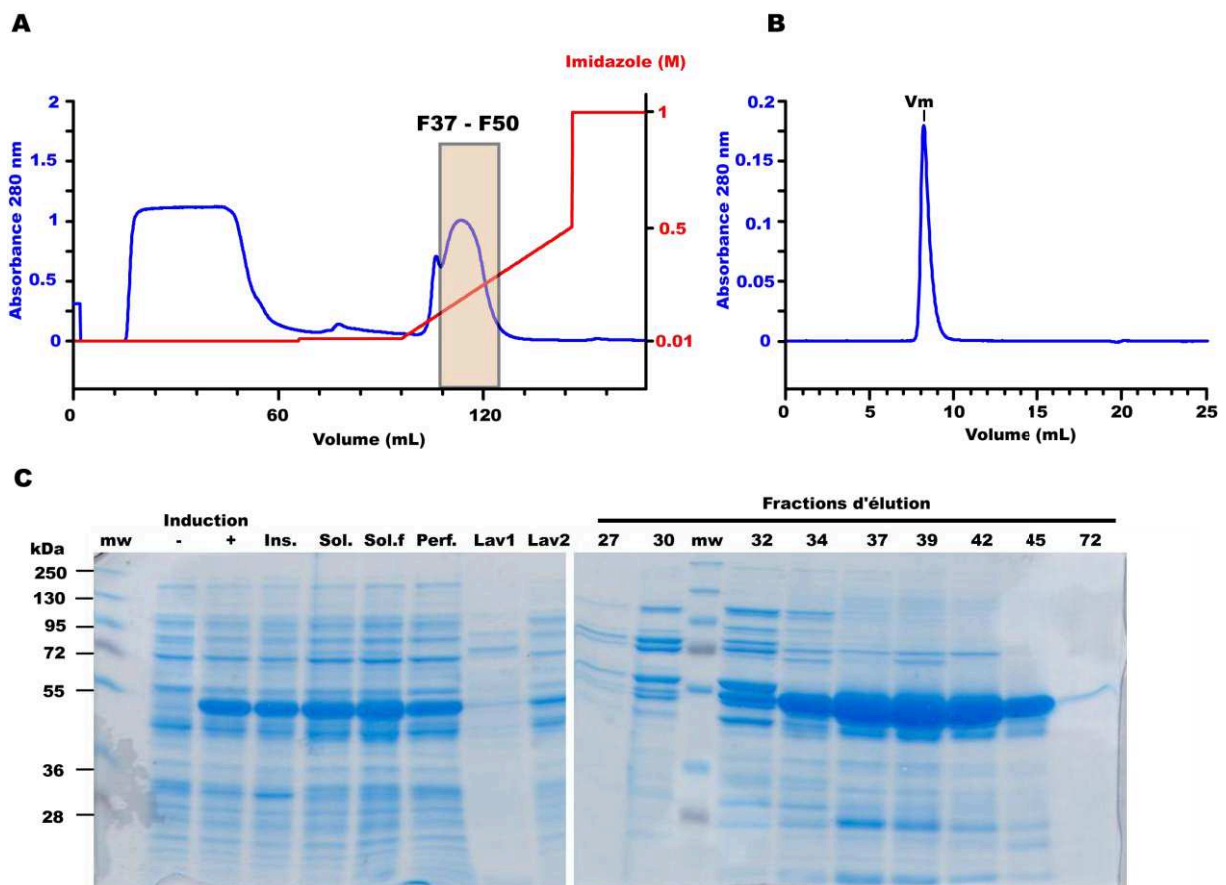
Figure 3.7 : Purification de la TcCRT « clean » produite en souche Shuffle
