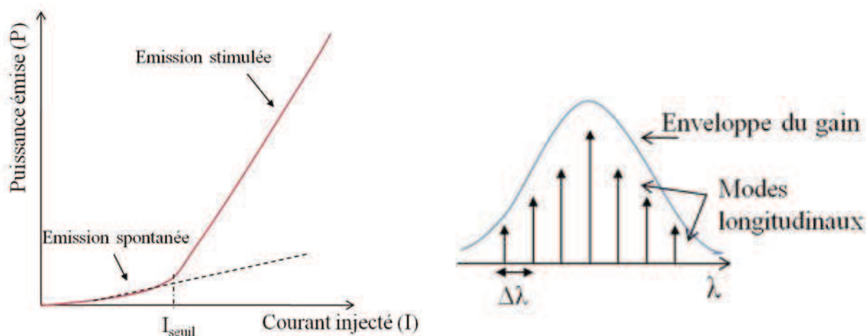
Figure 1.6 : A gauche : Courbe P(I) puissance émise en fonction du courant injecté. A droite : Schéma d'un spectre laser d'une cavité Fabry Péroth.
