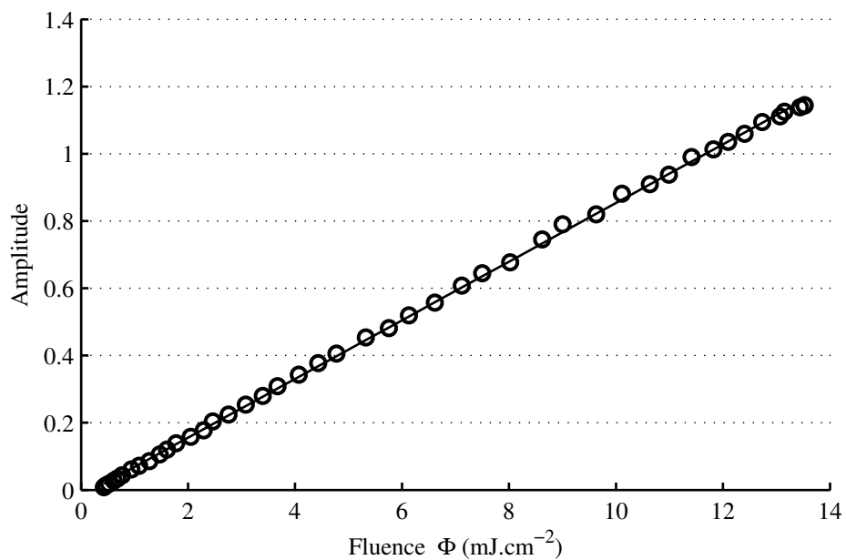
Figure VI.9 – Amplitude du signal photoacoustique émis par la solution de nanopshère d'or ( R_s = 10 nm) en fonction de la fluence incidente. Les points correspondent aux valeurs déterminées par l'expérience. La courbe en trait plein représente un ajustement linéaire des données de R^2 = 94.9 %.
