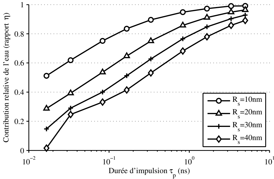
Figure V.11 – Contribution relative de l'eau à l'énergie photoacoustique totale générée, \eta(\tau_p, R_s) , en régime linéaire, en fonction de la durée d'impulsion \tau_p et du rayon de la nanosphère R_s , pour T_0 = 20^\circ\text{C} .
