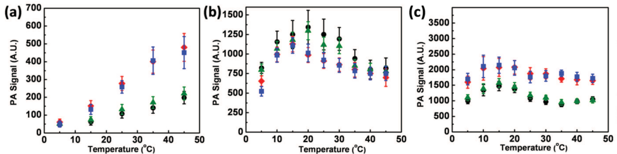
Figure III.5 – Amplitude du signal photoacoustique en fonction de la température, généré par une solution de nanosphères enrobées de PEG (ronds noirs), de nanosphères enrobées de silice d'épaisseur 6 nm (triangle verts), 18 nm (carré bleus), 38 nm (losange rouges), dans l'eau (a), l'huile de silicone (b) et le toluène (c). Comme on peut le voir sur ces trois graphiques le solvant influencent grandement le signal photoacoustique émis par les nanoparticules. Dans l'eau l'amplitude tend à s'annuler lorsque le coefficient de dilatation thermique de l'eau vaut 0. Ces résultats accréditent l'hypothèse de génération dans la couche de solvant entourant la particule, et non dans la particule elle-même, dans le cas d'une illumination nanoseconde. [Chen et al., 2012]
