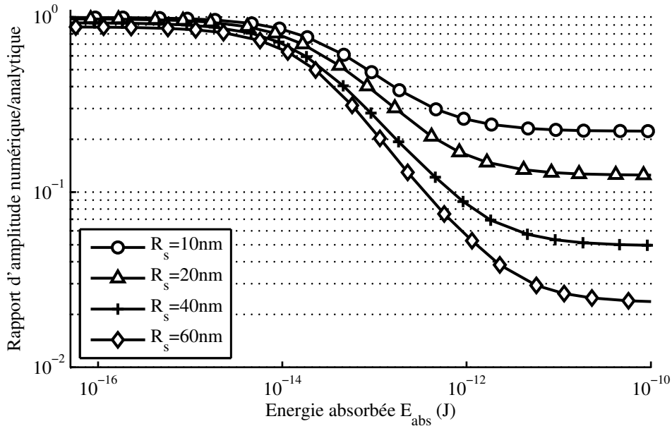
Figure V.20 – Amplitude photoacoustique générée par une nanosphère d'or et normalisée par l'amplitude du modèle de l'absorbant ponctuel, en fonction de l'énergie absorbée, et pour différentes taille R_s de particules. Lors de ces simulations la durée d'impulsion laser a été fixée à \tau_p = 5 ns et la température initiale à T_0 = 20^\circ\text{C} .
