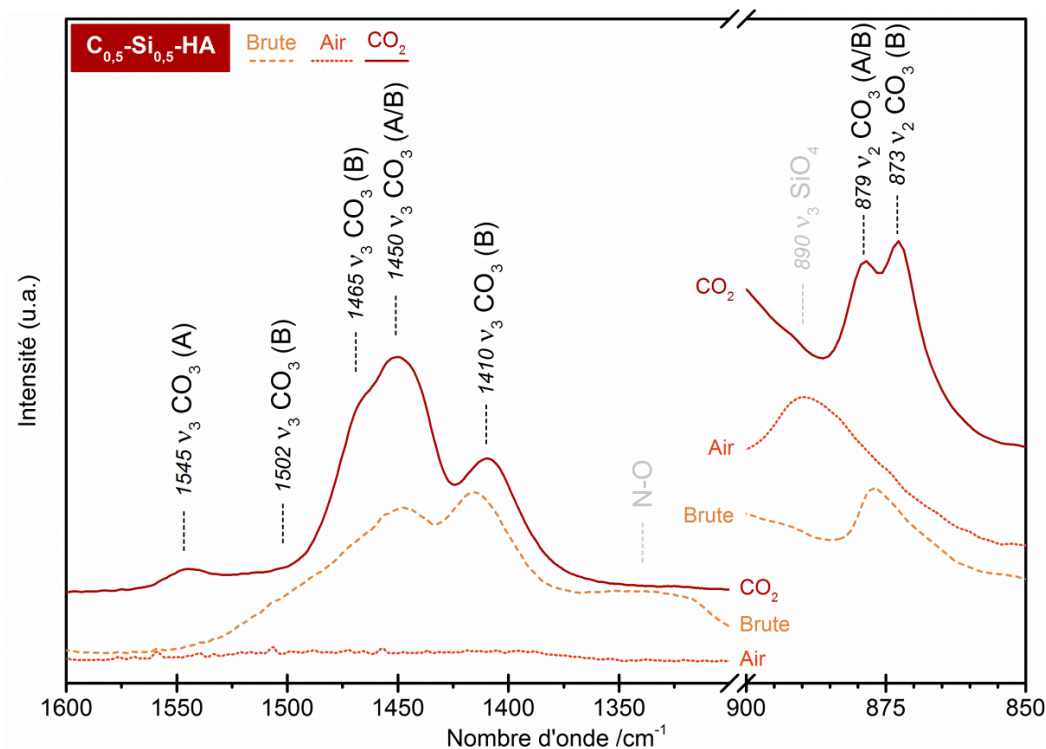
Figure 45 : Spectres IR de la poudre C_{0,5}\text{-Si}_{0,5}\text{-HA} réalisés avant calcination (tirets), après calcination à 1000^\circ\text{C} pendant 15 h sous air (pointillés), après calcination à 1000^\circ\text{C} pendant 1 h sous \text{CO}_2 (ligne continue) - domaines des \nu_2 et \nu_3 \text{CO}_3 .
