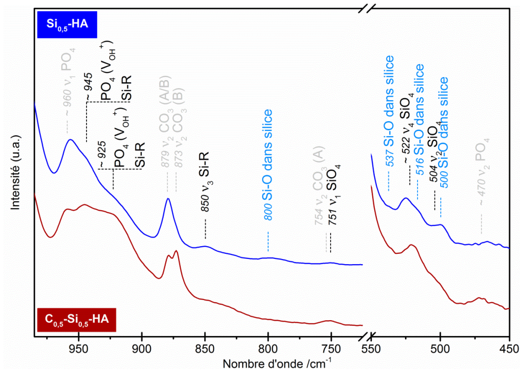
Figure 48 : Spectres IR des poudres C_{0,5}\text{-Si}_{0,5}\text{-HA} (rouge) et \text{Si}_{0,5}\text{-HA} (bleu) calcinées à 1000^\circ\text{C} pendant 1 h sous \text{CO}_2 - domaines des \text{SiO}_4 .
