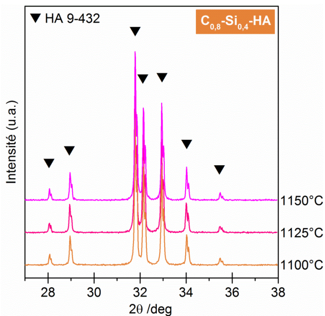
Figure 91 : Diffractogrammes des comprimés C_{0,8}-Si_{0,4}-HA frittés sous CO_2 à différentes températures pendant 1 h.
