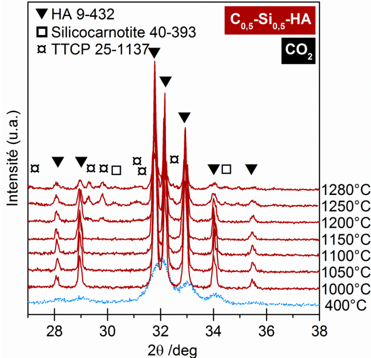
Figure 61 : Diffractogrammes de la poudre C_{0,5}-Si_{0,5}-HA calcinée sous CO_2 à différentes températures (de 400^\circ C à 1300^\circ C ).
