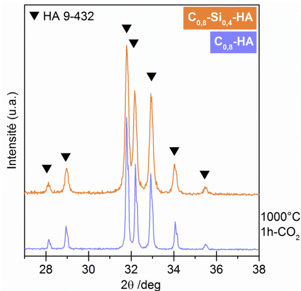
Figure 79 : Diffractogrammes des poudres C_{0,8}\text{-HA} et C_{0,8}\text{-Si}_{0,4}\text{-HA} après calcination à 1000^\circ\text{C} pendant 1 h sous \text{CO}_2 .
