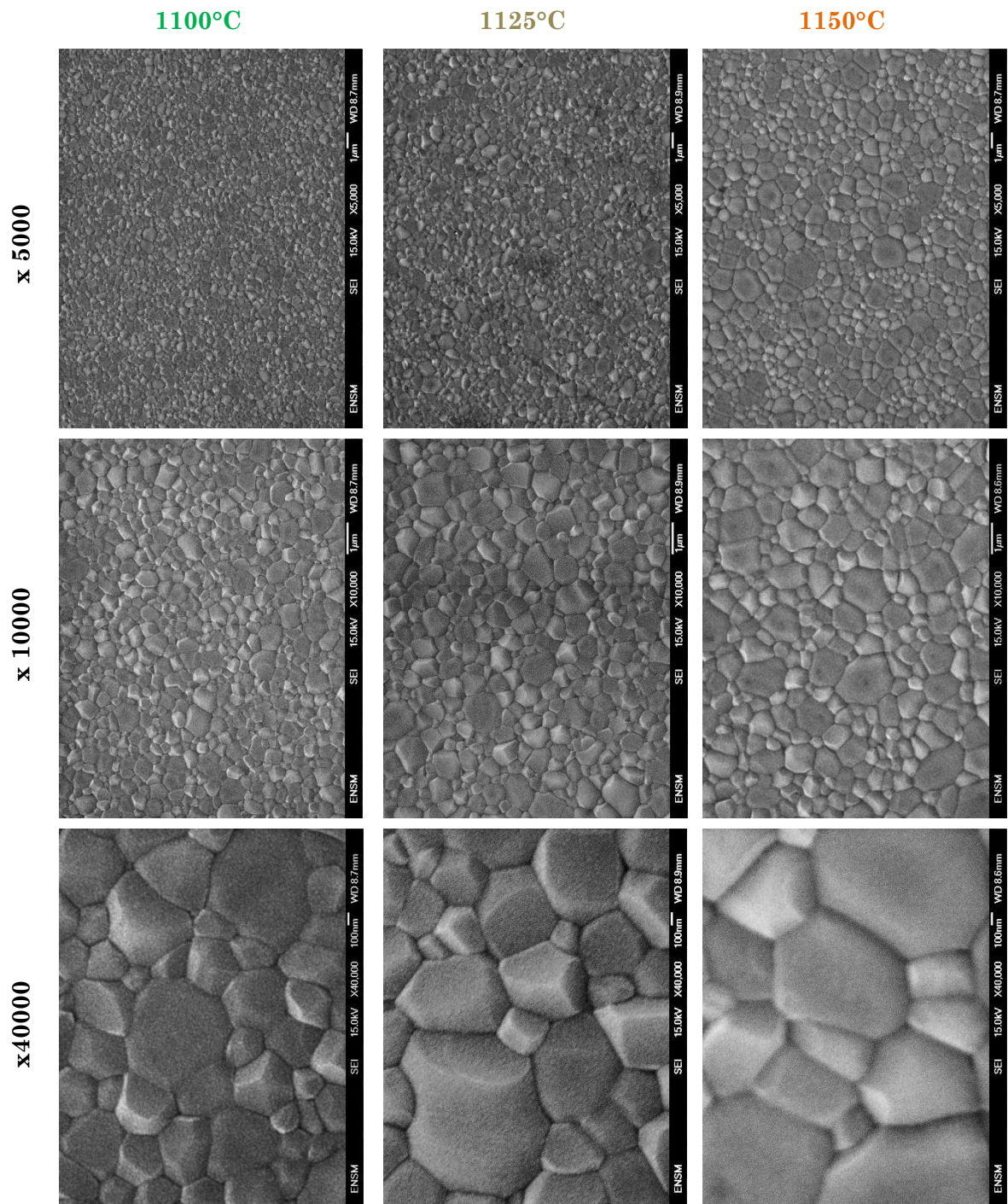
Figure 75 : Images MEB des comprimés de poudre C_{0,5}\text{-Si}_{0,5}\text{-HA} frittés sous \text{CO}_2 à 1100°C, 1125°C et 1150°C pendant 1 h.
