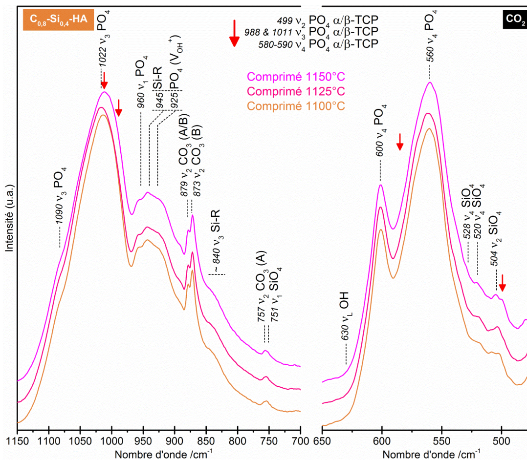
Figure 92 : Spectre IR des comprimés C_{0,8}-Si_{0,4}-HA frittés sous CO_2 à différentes températures pendant 1 h.
