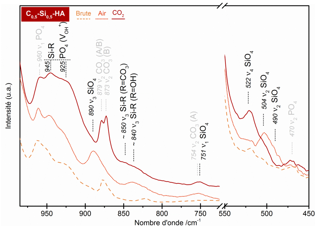
Figure 46 : Spectres IR de la poudre C_{0,5}\text{-Si}_{0,5}\text{-HA} réalisées avant calcination (tirets), après calcination à 1000^\circ\text{C} pendant 15 h sous air (pointillés), après calcination à 1000^\circ\text{C} pendant 1 h sous \text{CO}_2 (ligne continue) - domaines des \text{SiO}_4 .
