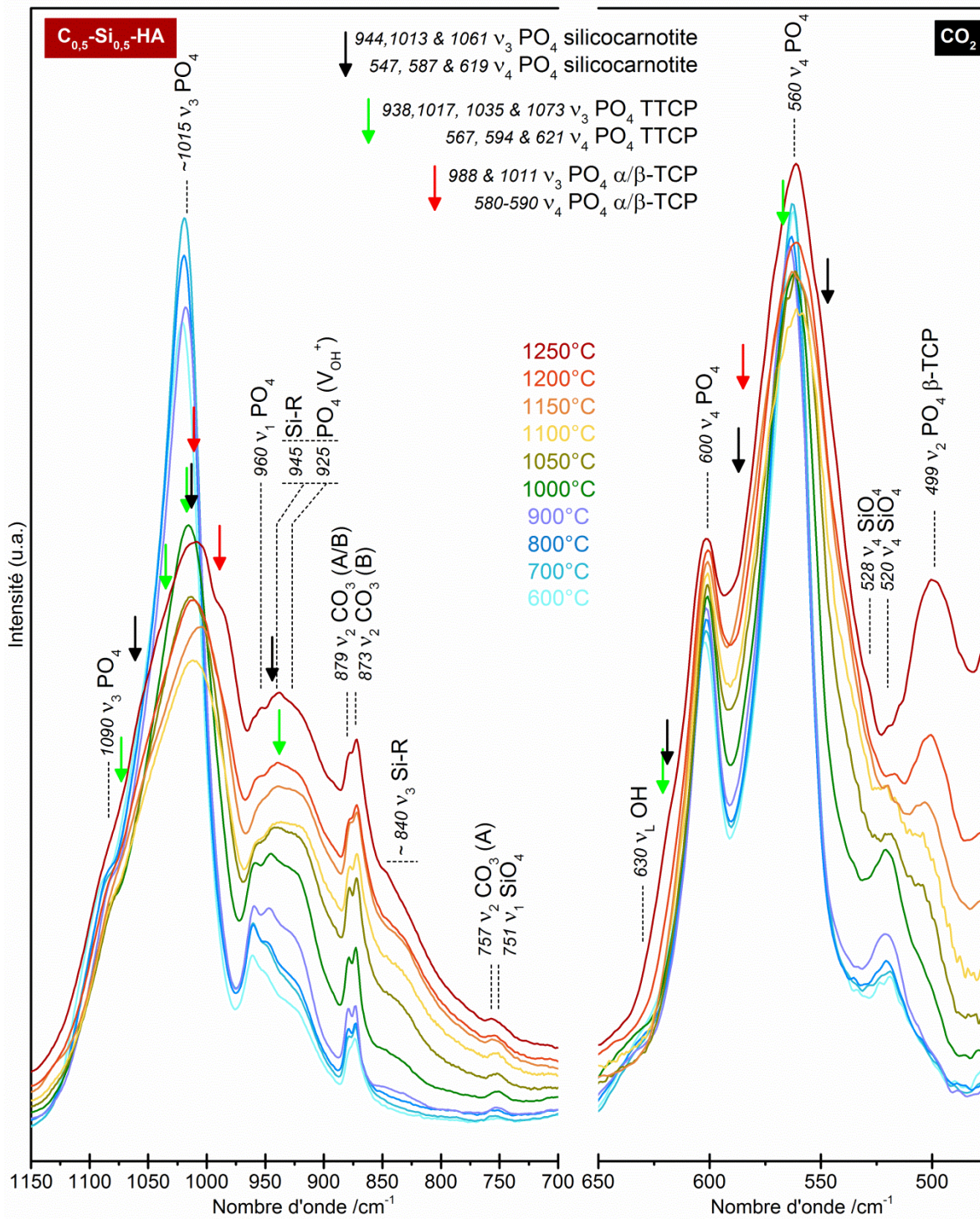
Figure 64 : Spectres IR de la poudre C_{0,5}-Si_{0,5}-HA calcinées sous CO_2 à différentes températures (de 600^\circ C à 1250^\circ C ) - domaine des v_3 et v_4 phosphates.
