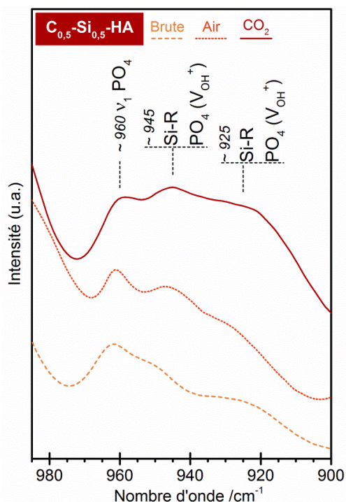
Figure 47 : Spectres IR de la poudre C_{0,5}\text{-Si}_{0,5}\text{-HA} réalisés avant calcination (tirets), après calcination à 1000^\circ\text{C} pendant 15 h sous air (pointillés), après calcination à 1000^\circ\text{C} pendant 1 h sous \text{CO}_2 (ligne continue) - domaines des dégénérescences \nu_1 \text{PO}_4 .
