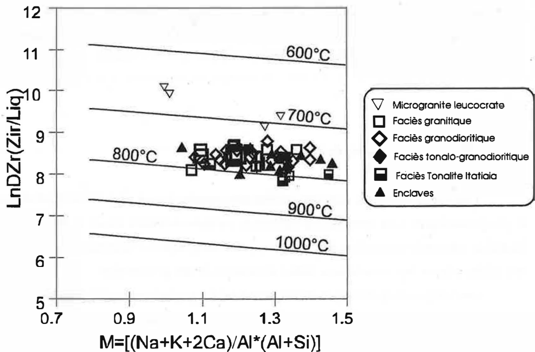
Figure III-3-1: Températures de cristallisation pour les granitoïdes de la suite Galiléa basées sur les teneurs en Zr de la roche (Watson & Harrison, 1983).
