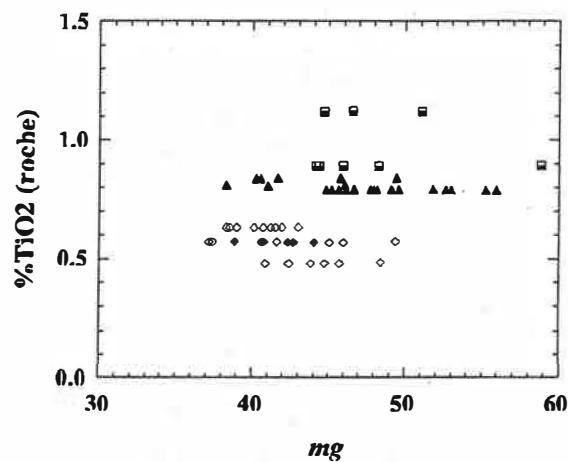
Figure III-1-2: Diagrammes MgO (A) et TiO 2 (B) de la roche hôte en fonction du mg ( =100 \cdot \text{Mg} / \text{Mg} + \text{Fe} ) des amphiboles des granitoïdes de la suite Galiléia.
