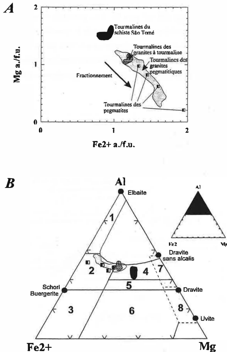
Figure V-6: A) Position des tourmalines noires des pegmatites dans le diagramme Mg en fonction de Fe^{2+} . Noter la superposition avec le champs des granites pegmatitiques; B) Position des tourmalines noires des pegmatites dans le diagramme Al-Fe-Mg (Henry & Guidotti, 1985). Les tourmalines des granitoïdes de la suite Urucum et du schiste São Tomé (voir légende dans la figure A) sont montrées à titre comparatif. Les différents champs représentent des tourmalines des: 1-pegmatites et aplites riches en Li; 2- granitoïdes, pegmatites et aplites pauvres en Li; 3- roches à quartz-tourmaline riches en Fe^{3+} ; 4- métapelites et métapsamites associées avec une phase saturée en Al; 5- métapelites et métapsamites qui ne sont pas associées avec une phase saturée en Al; 6- roches à quartz-tourmaline riches en Fe^{3+} , roches calco-silicatés et métapelites; 7- roches métaultramafiques pauvres en Ca et des métasédiments riches en V et Cr; 8- métacarbonates et meta-pyroxénites.
