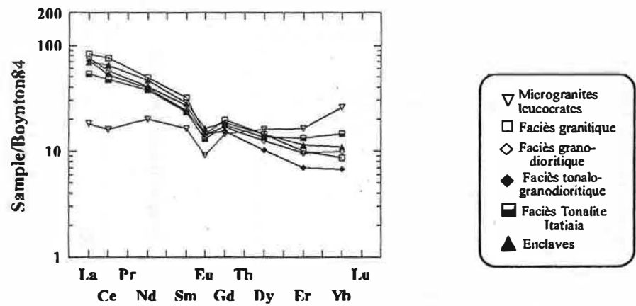
Figure III-2-11: Spectres d'éléments terres rares des certains échantillons représentatifs de la suite Galiléia. Normalisés par rapport aux valeurs des chondrites de Boynton (1984).
