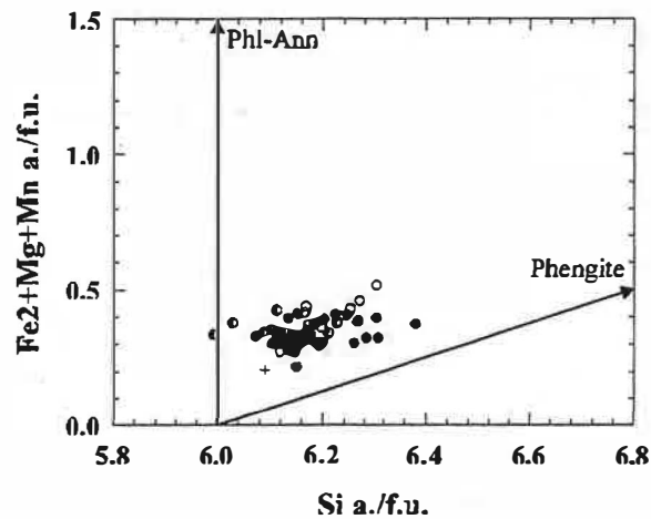
Figure IV-1-8: Position des muscovites des granites de la suite Urucum dans les digrammes Fe^{2+}+Mg+Mn en fonction du Al^{total} (diagramme A) et en fonction du Si (diagramme B). Ces diagrammes montrent l'importance de la substitution phengitique dans ces muscovites.
