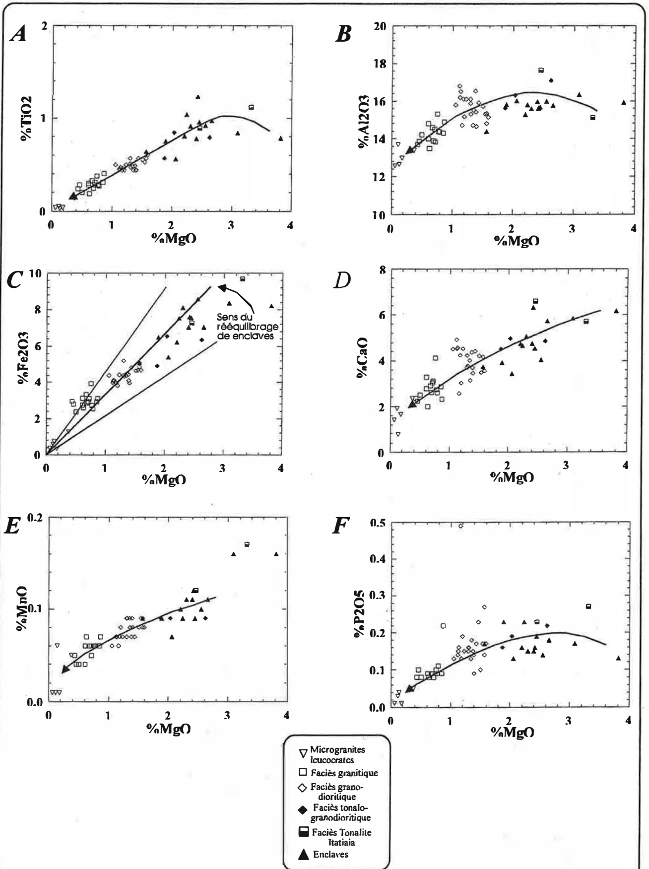
Figure III-2-4: Position des différents faciès de la suite Galiléia dans les diagrammes \text{TiO}_2 (A), \text{Al}_2\text{O}_3 (B), \text{Fe}_2\text{O}_3 (C), \text{CaO} (D), \text{MnO} (E) et \text{P}_2\text{O}_5 (F) en fonction du \text{MgO} .
