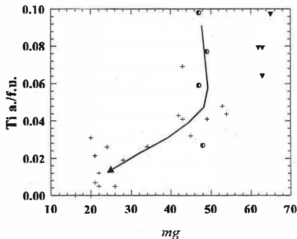
Figure IV-1-13: Evolution des compositions des tourmalines des granitoïdes de la suite Urucum. Les tourmalines du micaschiste São Tomé sont montrées à titre comparatif. Le diagramme A montre l'augmentation du Mn avec la diminution du rapport mg ( =100 \cdot Mg/(Mg+Fe) ). Le diagramme B montre la diminution du Ti avec la diminution du rapport mg .
