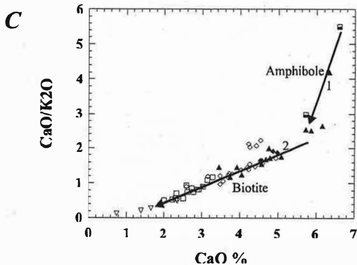
Figure III-2-5: Position des granitoïdes de la suite Galiléia dans les diagrammes FMMT versus CaO/K 2 O (diagramme A), CaO versus Na 2 O/K 2 O (B) et CaO versus CaO/K 2 O (C). Ces diagrammes soulignent le rôle du fractionnement du plagioclase, de la biotite, de l'amphibole et du feldspath potassique.
