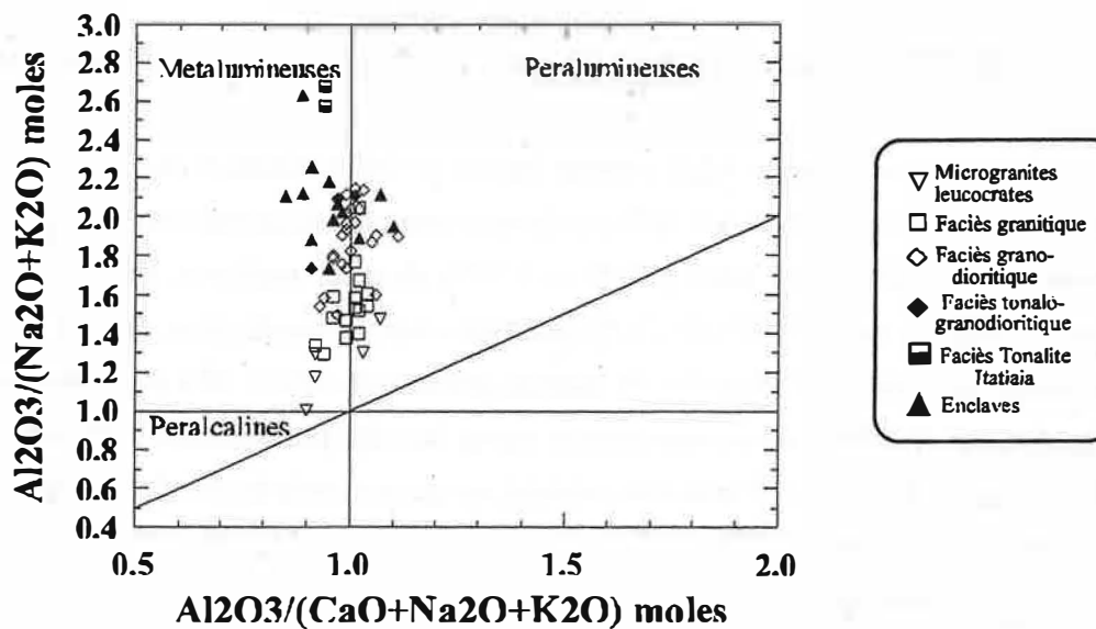
Figure III-2-1: Position des granitoïdes de la suite Galiléa dans le diagramme A/CNK (indice de saturation en alumine de Shand, 1949) versus A/NK en moles .
