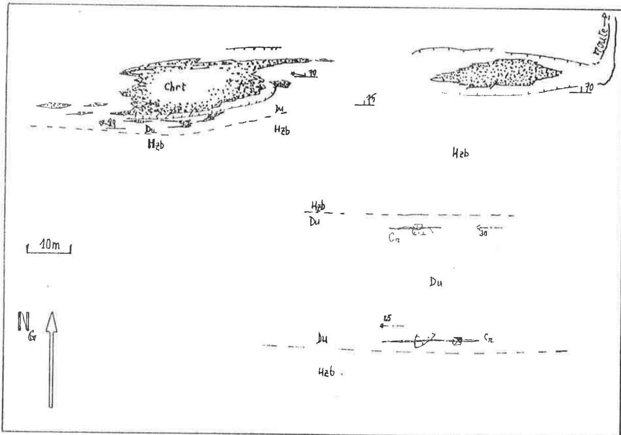
FIG. 32 . PLAN SCHEMATIQUE DE LA MINE DAMOCLÈS
