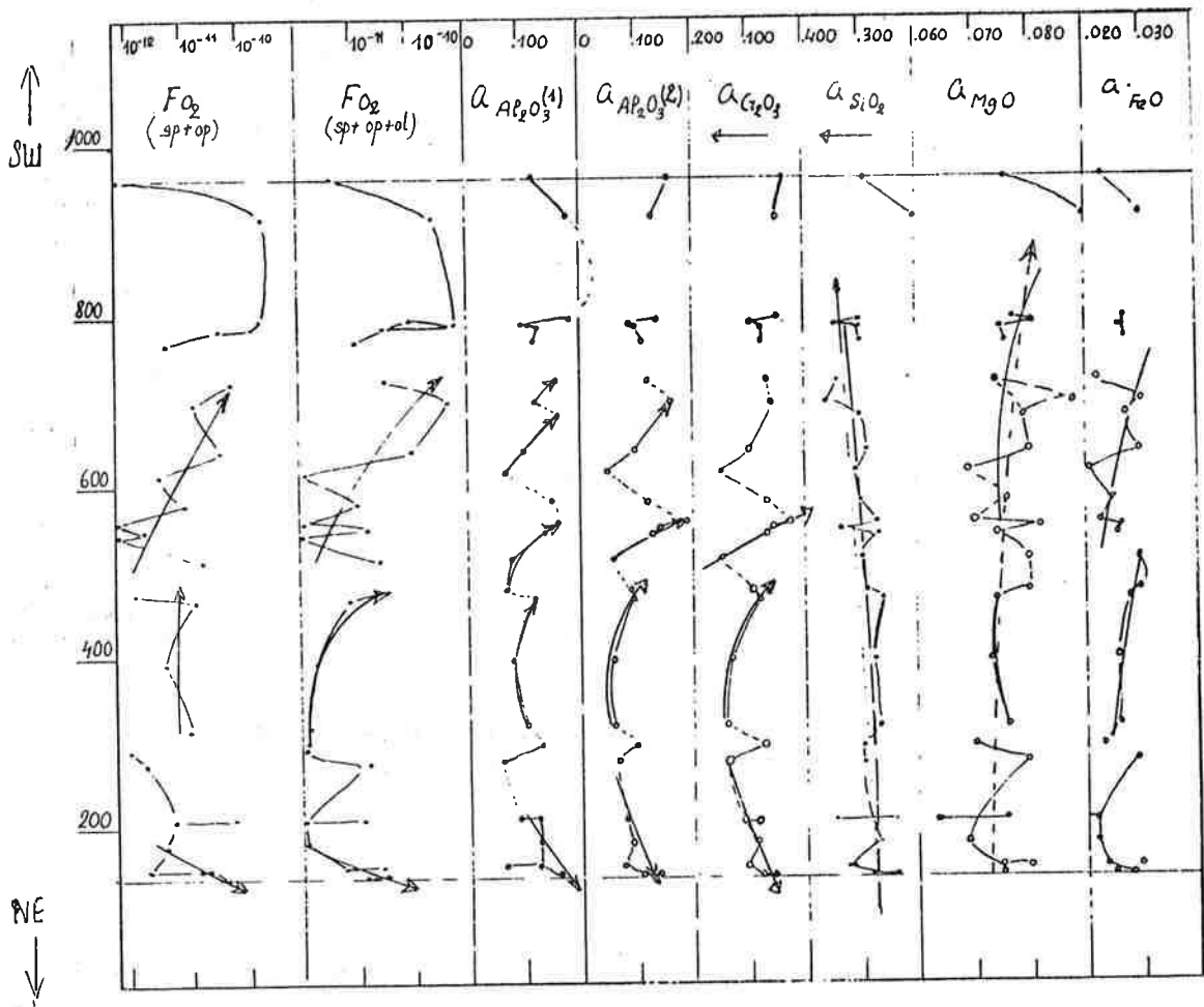
FIG. 88a - FUGACITÉS ET ACTIVITÉS CALCULÉES POUR LES ÉCHANTILLONS DU 'TUNNEL'
