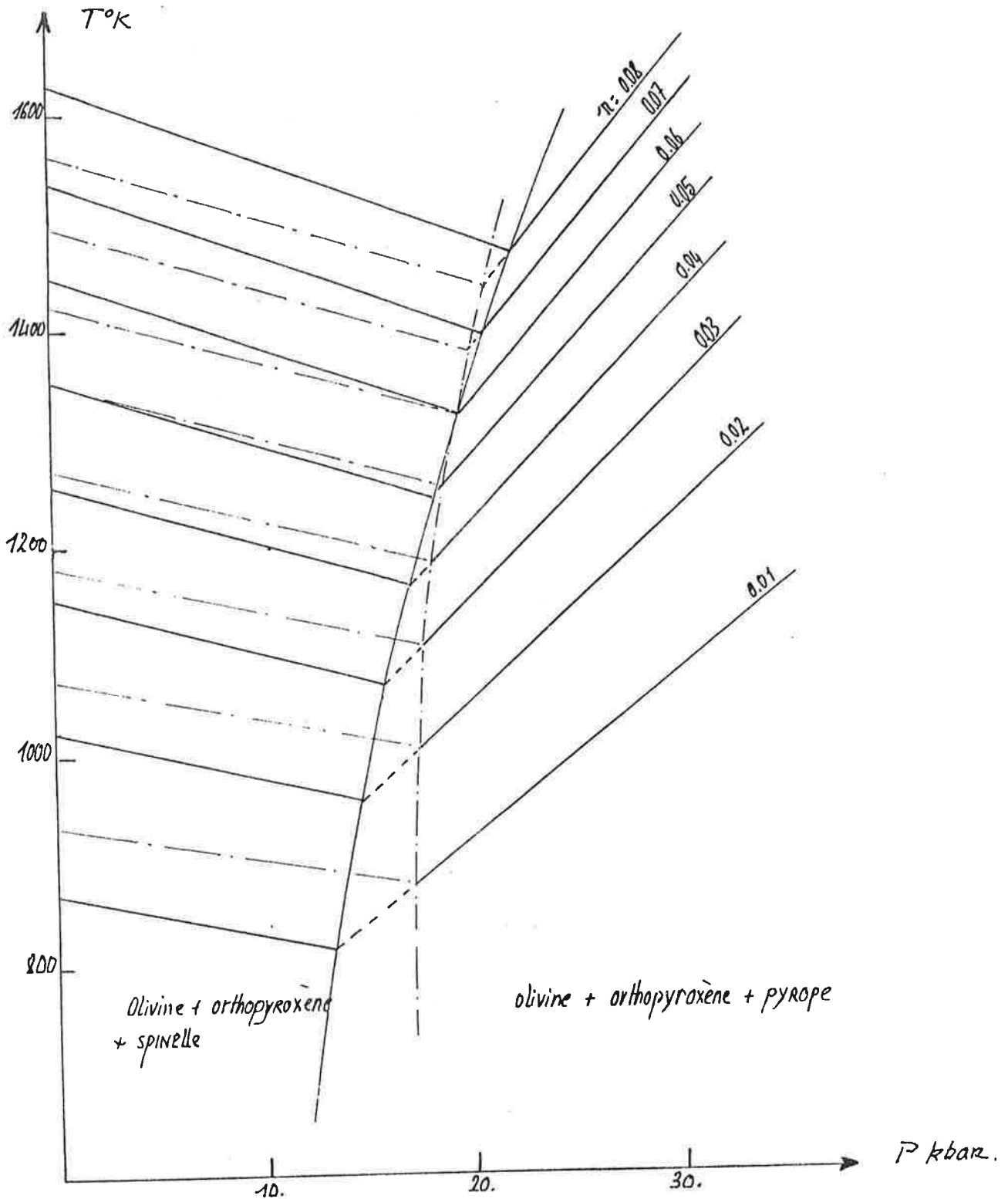
FIG. 67 - COURBES D'ISOTENEUR EN ALUMINE DANS LE PYROXÈNE, DANS LE SYSTÈME (MgO, Al 2 O 3 , SiO 2 ) — PREMIÈRE MÉTHODE - - - DEUXIÈME MÉTHODE (voir texte)
