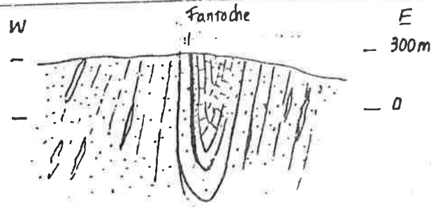
fig. 40 Coupes structurales du Massif de Tiébaghi
