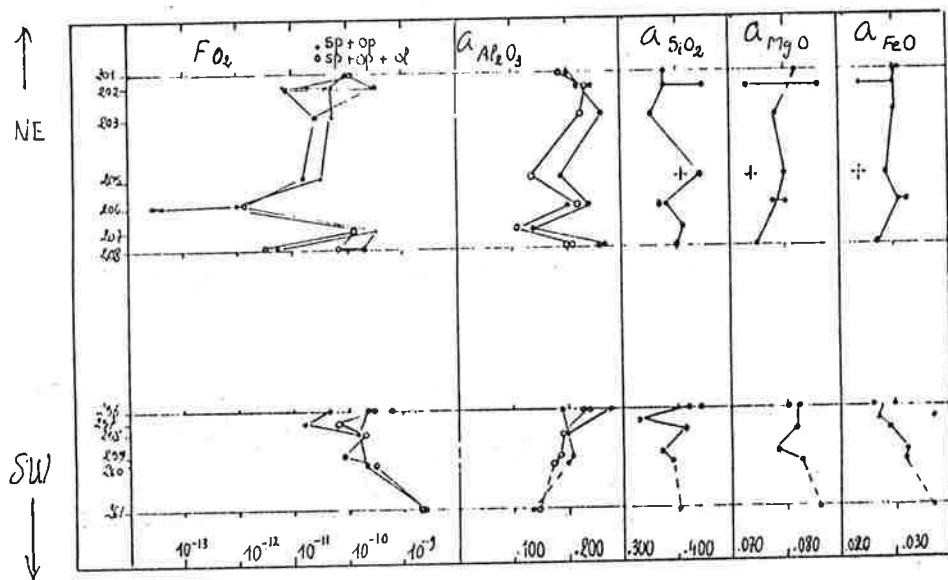
FIG. 88b - FUGACITÉS ET ACTIVITÉS CALCULÉES POUR LES ÉCHANTILLONS DU TELEBENIVE
