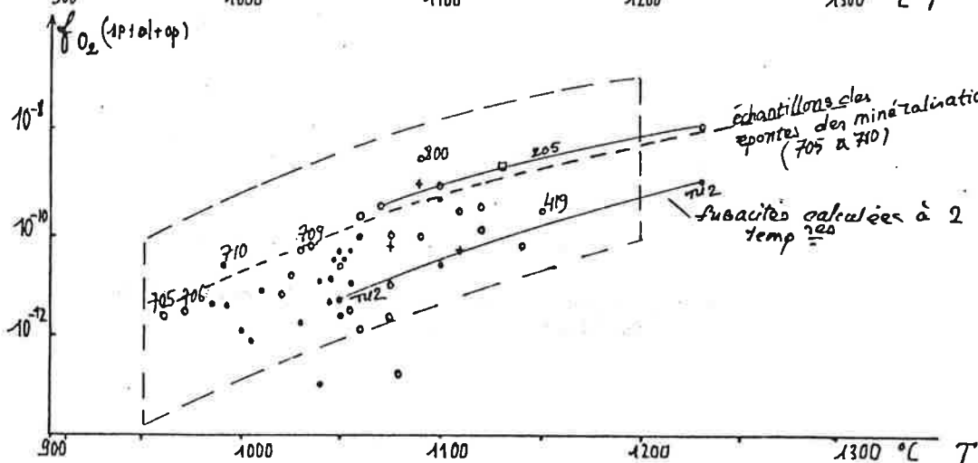
FIG. 70 — DIAGRAMMES ( T, f_{O_2} ) POUR LES ROCHES DE TIÉBAGHI
