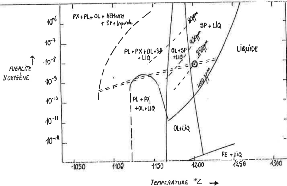
FIG 77 - DIAGRAMME DE HILL ET ROEDER, (1974)
