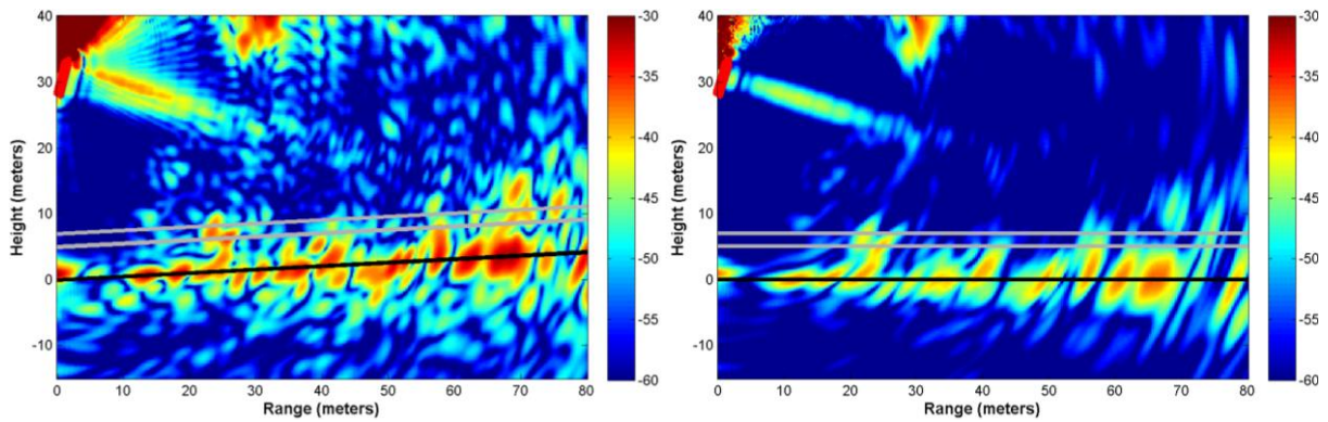
Figure 52. Tomogrammes bruts de P0 (gauche) puis avec apodisation et correction de la pente (droite) pour les polarisations, de haut en bas, HH, HV, VH et VV. Les positions des antennes sont dessinées en rouge en haut à gauche, le niveau du sol en noir, et les mesures de hauteur de la canopée en gris.
