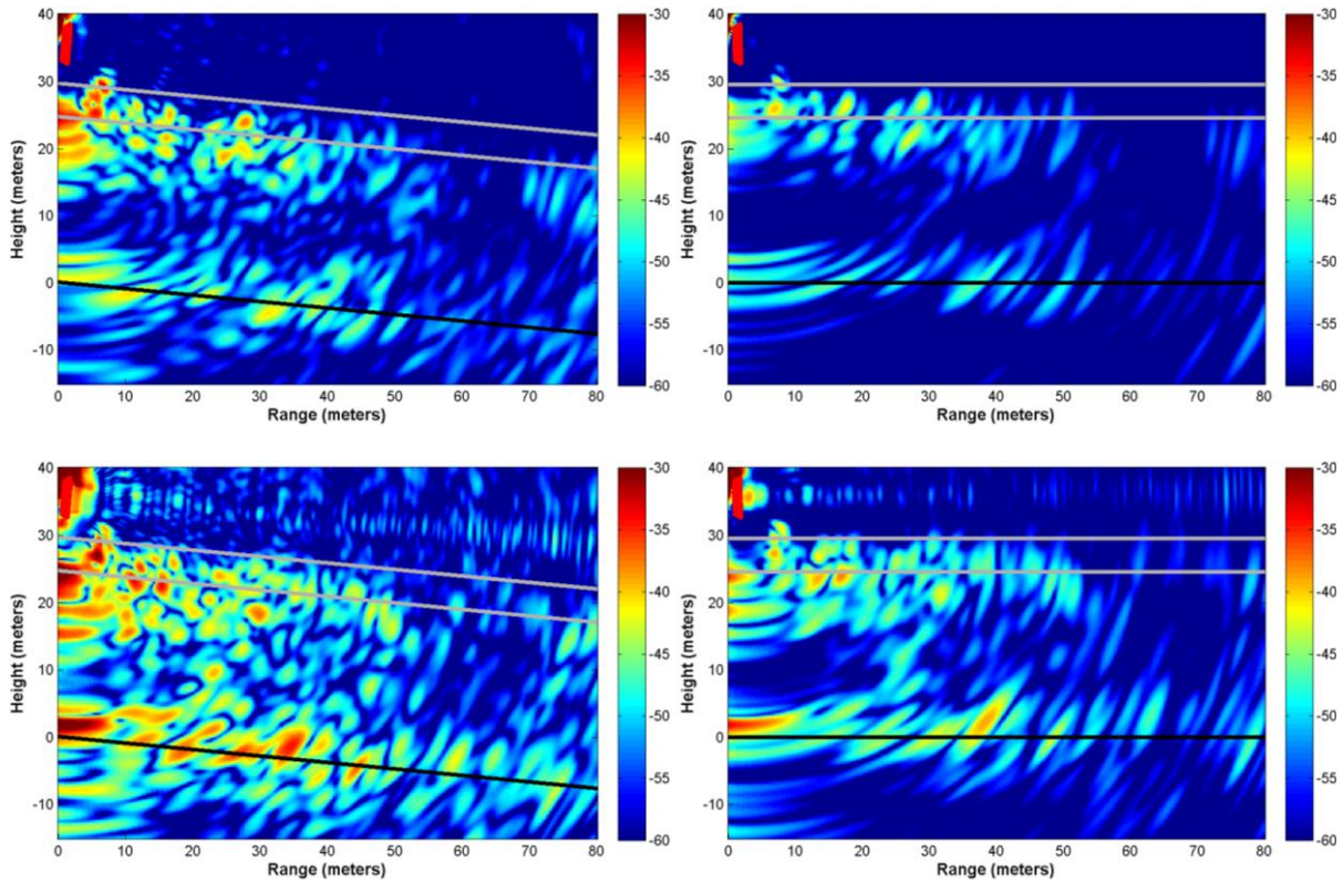
Figure 64. Tomogrammes bruts de P5 (gauche) puis avec apodisation et correction de la pente (droite) pour les polarisations, de haut en bas, HH, HV, VH et VV. Les positions des antennes sont dessinées en rouge en haut à gauche, le niveau du sol en noir, et les mesures de hauteur de la canopée en gris.
