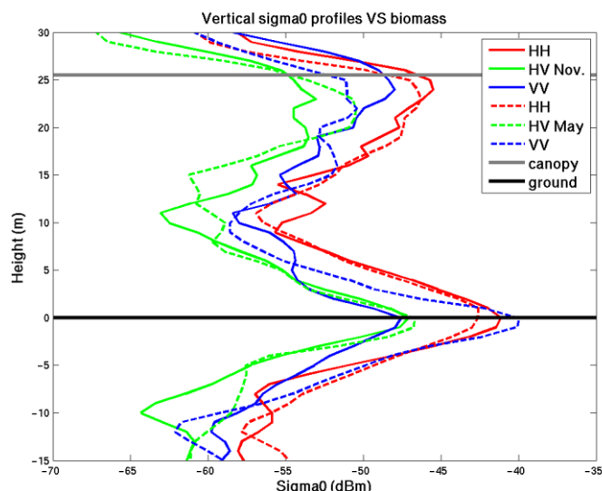
Figure 73. Profils verticaux de rétrodiffusion de P1 en novembre (P1N) et en mai (P1M).
