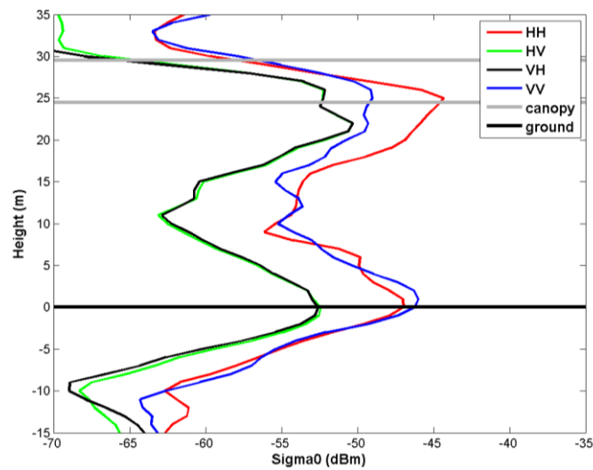
Figure 65. Profils verticaux de rétrodiffusion de P5 obtenus à partir des tomogrammes avec apodisation.
