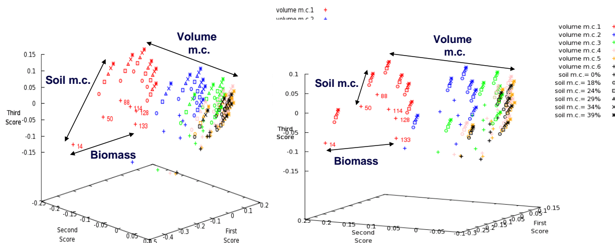
Figure 40. Résultat d'une Analyse en Composantes Principales sur des coefficients de rétrodiffusion radar HH, HV, VV ainsi que sur des indices optiques NDVI, GVMI, NINSOL (gauche) et sur les mêmes données à l'exception du coefficient de rétrodiffusion en VV (droite).
