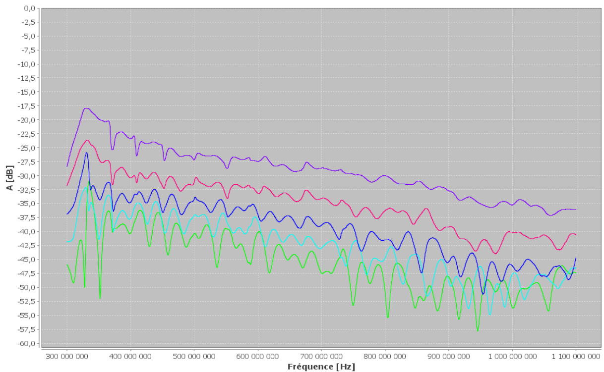
Figure 42. Couplage entre antennes pour la polarisation HV (S12) ; l'espacement varie de 30 à 70 cm, respectivement du violet au vert.
