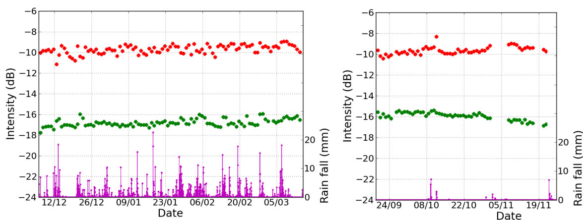
Figure 37. Séries temporelles des coefficients de rétrodiffusion HH (rouge) et HV (vert) acquis à 18:00 avec l'expérimentation TropiScat, sur la forêt complète, pour la saison humide (gauche) et pour la saison sèche (droite).
