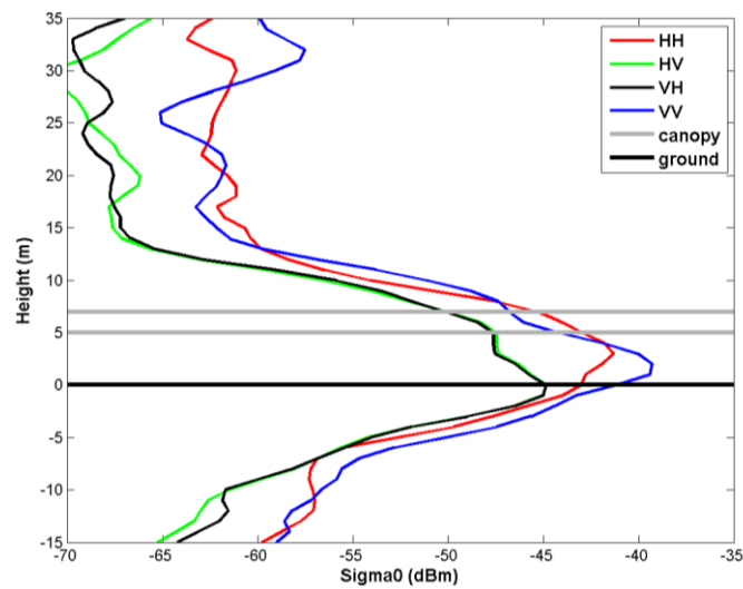
Figure 69. Profils verticaux de rétrodiffusion de P7 obtenus à partir des tomogrammes avec apodisation.
