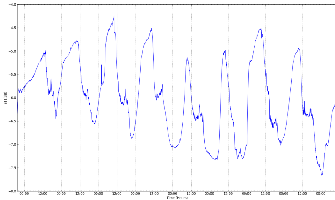
Figure 33. Coefficient de rétrodiffusion tracé en fonction du temps.
