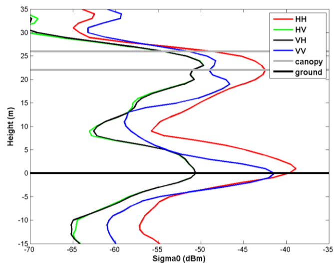
Figure 61. Profils verticaux de rétrodiffusion de P3 obtenus à partir des tomogrammes avec apodisation.
