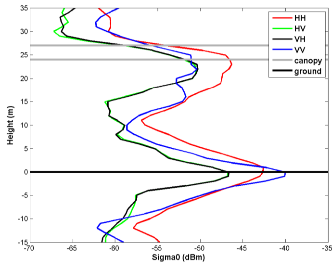
Figure 57. Profils verticaux de rétrodiffusion de P1M obtenus à partir des tomogrammes avec apodisation.
