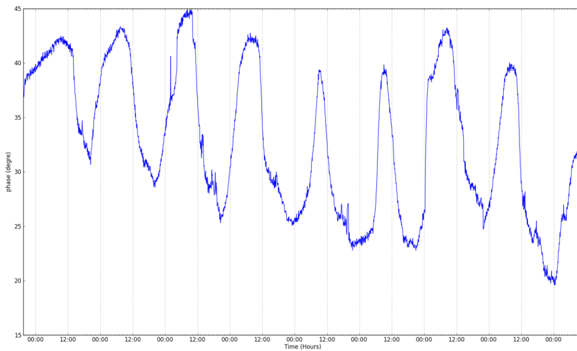
Figure 34. Phase Coefficient de rétrodiffusion tracé en fonction du temps.
