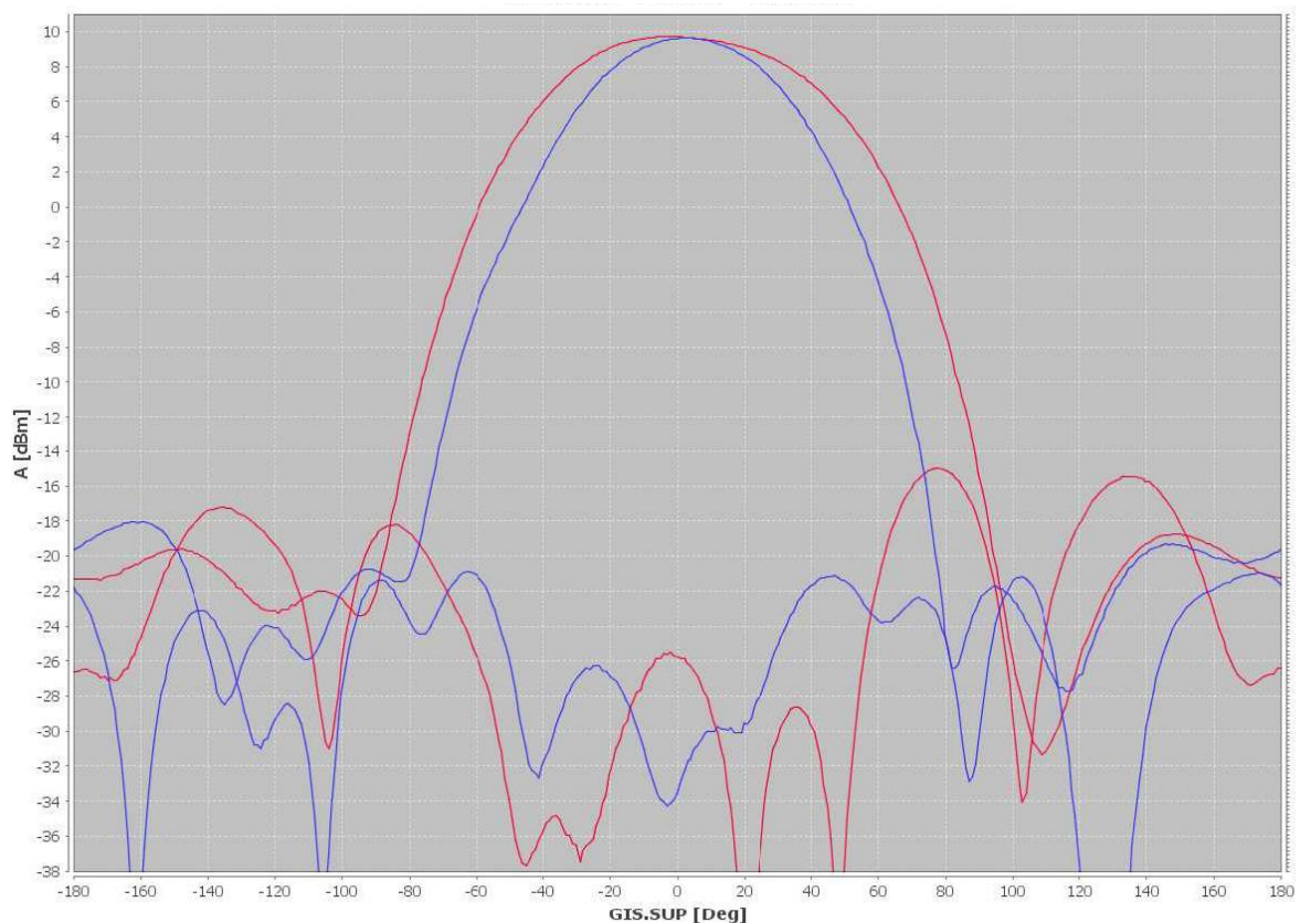
Figure 41. Diagrammes de rayonnement pour les plans E et H, respectivement bleu et rouge, en polarisation croisée et en co-polarisation.
