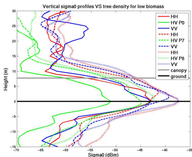
Figure 72. Profils verticaux de rétrodiffusion de P0, P7 et P8.
