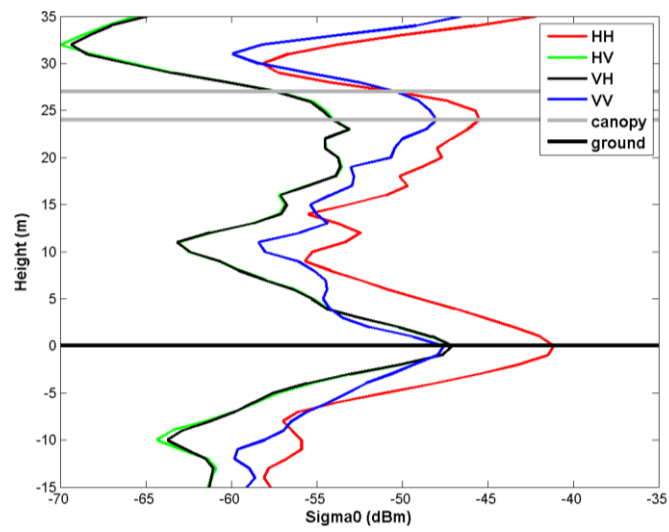
Figure 55. Profils verticaux de rétrodiffusion de P1N obtenus à partir des tomogrammes avec apodisation.
