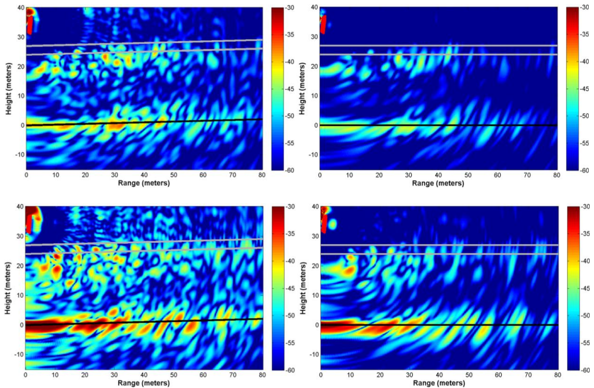
Figure 56. Tomogrammes bruts de P1M (gauche) puis avec apodisation et correction de la pente (droite) pour les polarisations, de haut en bas, HH, HV, VH et VV. Les positions des antennes sont dessinées en rouge en haut à gauche, le niveau du sol en noir, et les mesures de hauteur de la canopée en gris.
