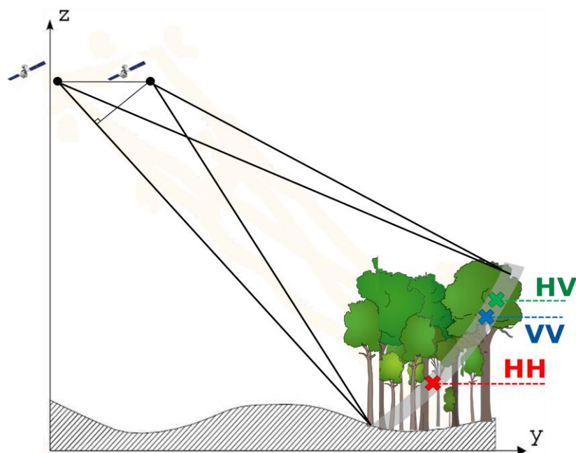
Figure 11. Lignes de vol de l'instrument et hauteurs du centre de phase interférométrique pour chaque polarisation. Les positions des centres de phases obtenues permettent d'estimer la hauteur de la canopée
