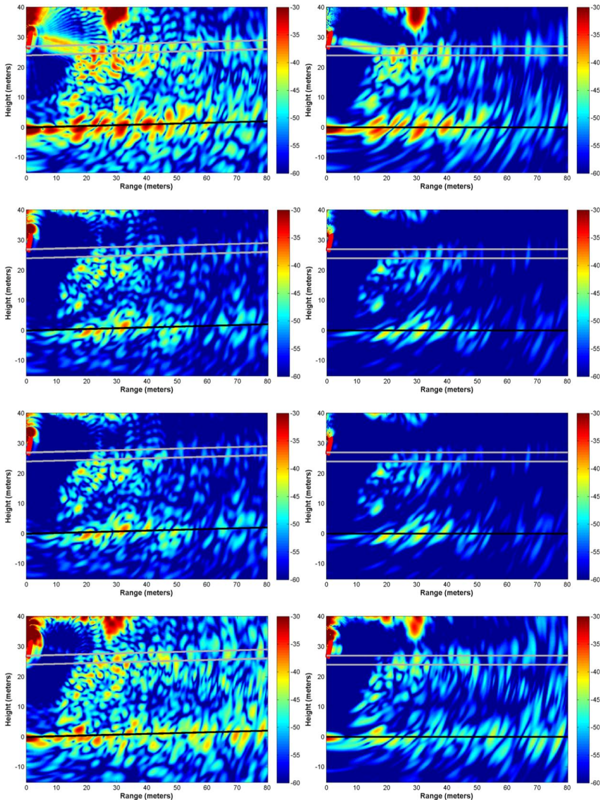
Figure 54. Tomogrammes bruts de P1N (gauche) puis avec apodisation et correction de la pente (droite) pour les polarisations, de haut en bas, HH, HV, VH et VV. Les positions des antennes sont dessinées en rouge en haut à gauche, le niveau du sol en noir, et les mesures de hauteur de la canopée en gris.
