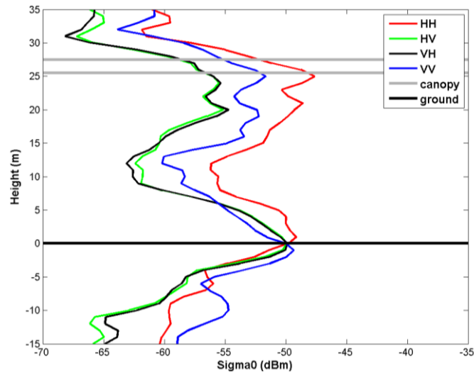
Figure 63. Profils verticaux de rétrodiffusion de P4 obtenus à partir des tomogrammes avec apodisation.
