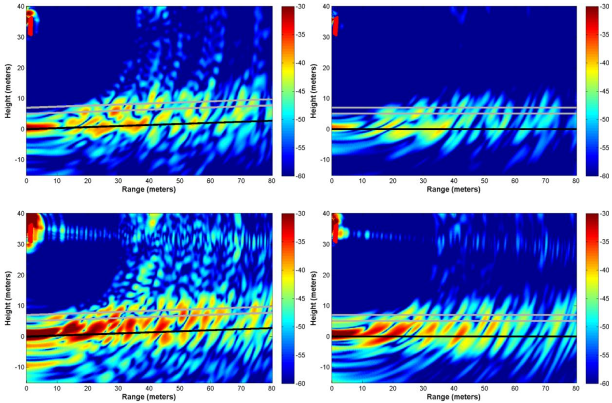
Figure 68. Tomogrammes bruts de P7 (gauche) puis avec apodisation et correction de la pente (droite) pour les polarisations, de haut en bas, HH, HV, VH et VV. Les positions des antennes sont dessinées en rouge en haut à gauche, le niveau du sol en noir, et les mesures de hauteur de la canopée en gris.
