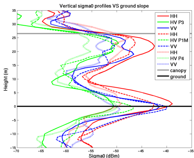
Figure 77. Profils verticaux de rétrodiffusion de P3, P1M et P4.
