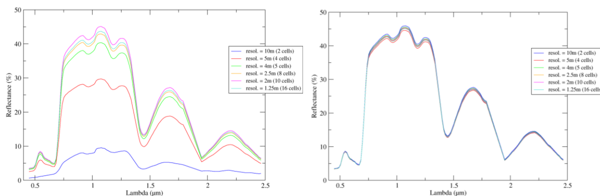
Figure 26. Spectres en réflectance avant refonte des modules (gauche) et après refonte (droite).
