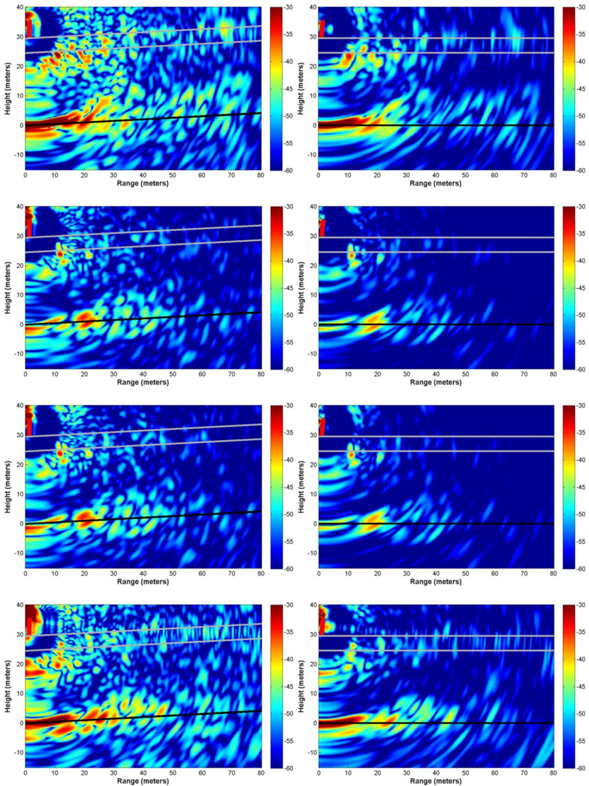
Figure 66. Tomogrammes bruts de P6 (gauche) puis avec apodisation et correction de la pente (droite) pour les polarisations, de haut en bas, HH, HV, VH et VV. Les positions des antennes sont
