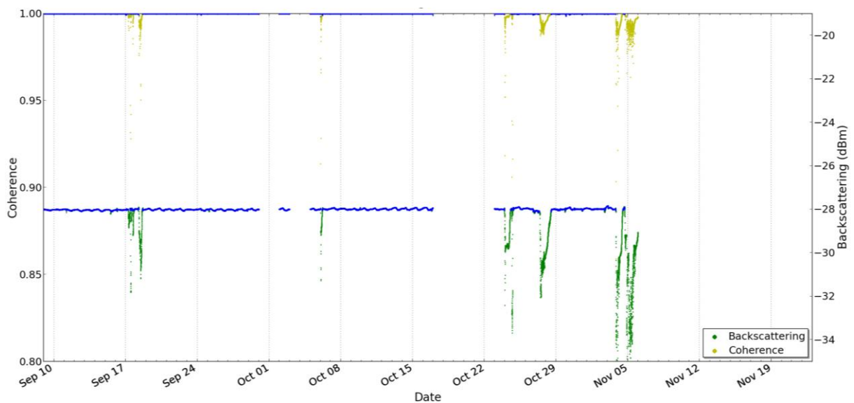
Figure 45. Coefficient de rétrodiffusion et cohérence du couplage pour TS-AUTUMN ; les données filtrées conservées sont indiquées en bleu.
