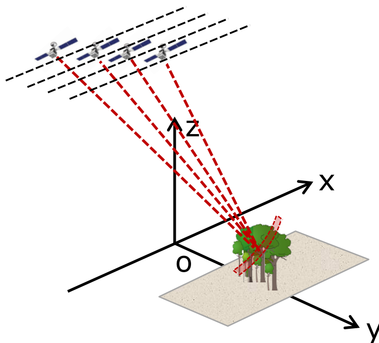
Figure 12. Lignes de vol de l'instrument et reconstruction verticale de la forêt (crédits: Le Toan et al.)
