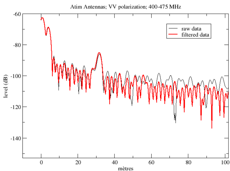
Figure 30. Réponse impulsionnelle acquise depuis le drone en polarisation VV. La réponse du trièdre est visible à 30 m.
