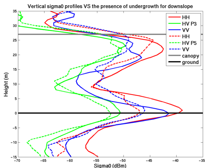
Figure 75. Profils verticaux de rétrodiffusion de P3 et P5.
