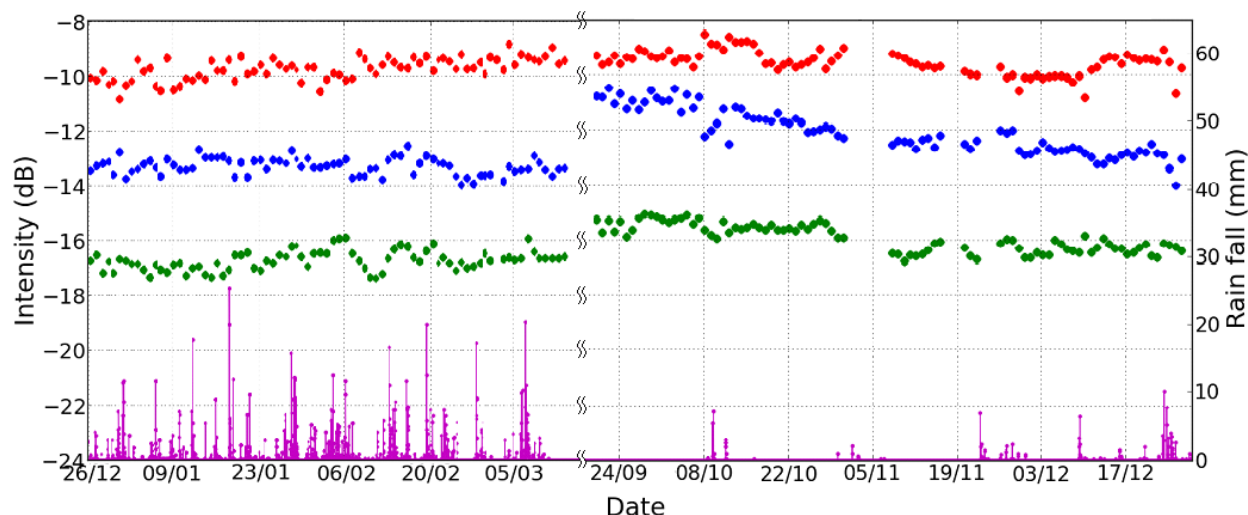
Figure 38. Variation du coefficient de rétrodiffusion mesuré lors de l'expérimentation TropiScat, sur la forêt complète, pris à 6:00 et moyenné sur 16 couples d'antennes le premier et le dernier trimestre de l'année 2012.
