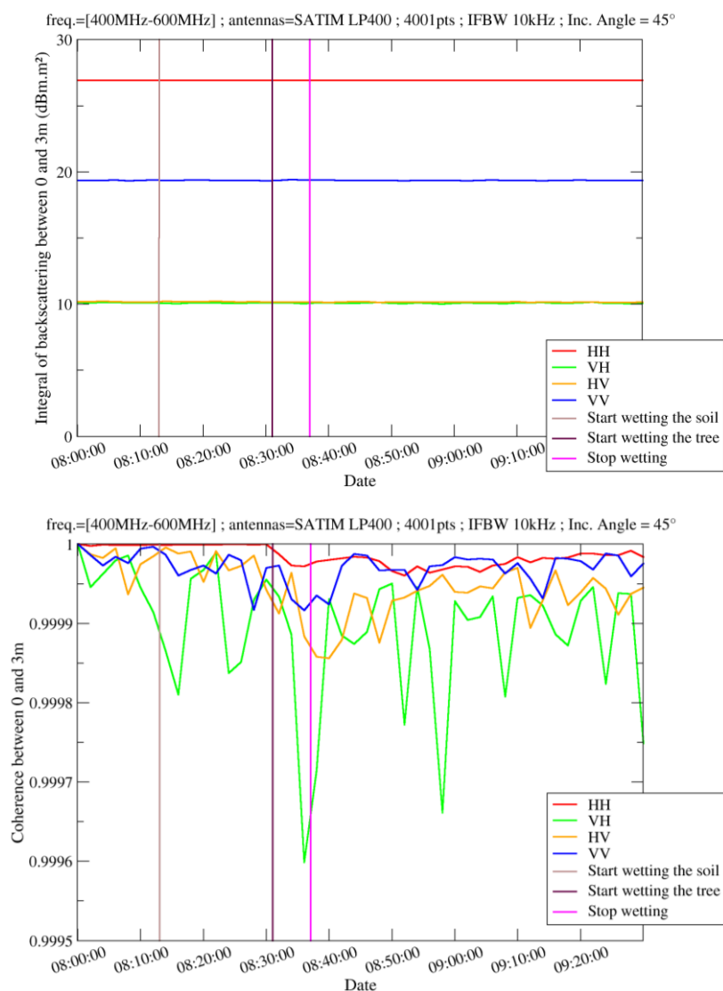
Figure 44. Coefficient de rétrodiffusion et cohérence du couplage pour STS.
