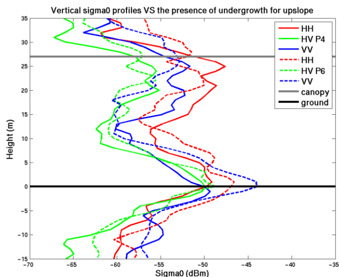
Figure 76. Profils verticaux de rétrodiffusion de P4 et P6.
