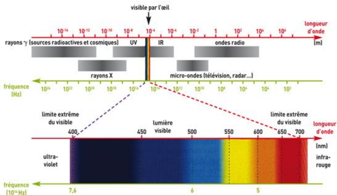
Figure 5. Spectre électromagnétique incluant le domaine visible et le domaine des ondes radio [Durandeau et al., 2002].
