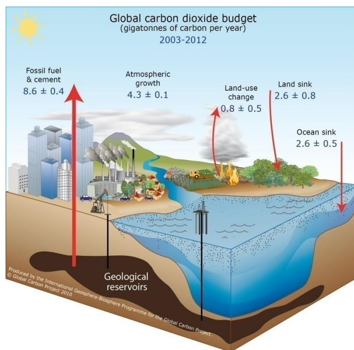
Figure 1. Echanges de CO 2 à l'échelle de mondiale, en gigatonne de carbone par an [Le Quéré et al., 2013].
