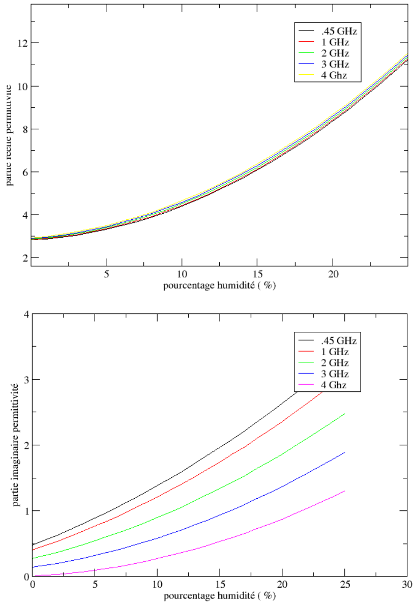
Figure 9. Partie réelle (haut) et partie imaginaire (bas) de la permittivité du sable en fonction du taux d'humidité [Crédits : Borderies et al.]
