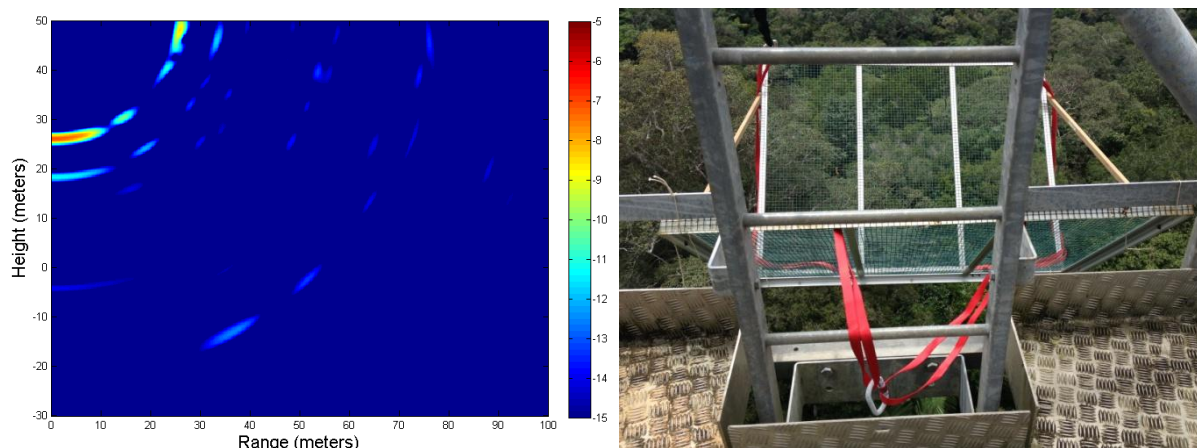
Figure 21. TropicScat : Réponse du trièdre à 25 m de haut en tomographie verticale (gauche) et dièdre installé sur la tour de façon durable à 35 m de haut (droite).
