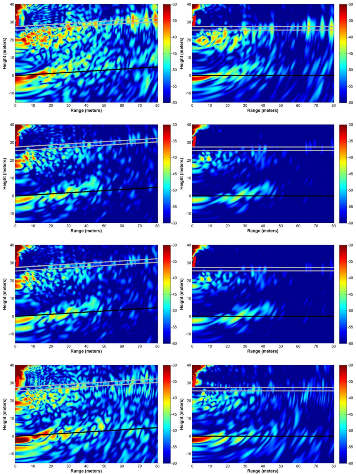
Figure 62. Tomogrammes bruts de P4 (gauche) puis avec apodisation et correction de la pente (droite) pour les polarisations, de haut en bas, HH, HV, VH et VV. Les positions des antennes sont
