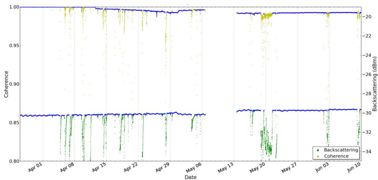
Figure 47. Coefficient de rétrodiffusion et cohérence du couplage pour TS-SPRING ; les données filtrées conservées sont indiquées en bleu.
