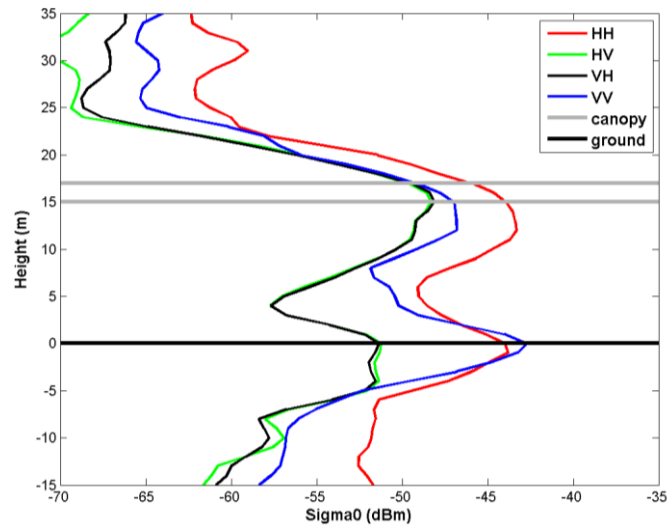
Figure 59. Profils verticaux de rétrodiffusion de P2 obtenus à partir des tomogrammes avec apodisation.
