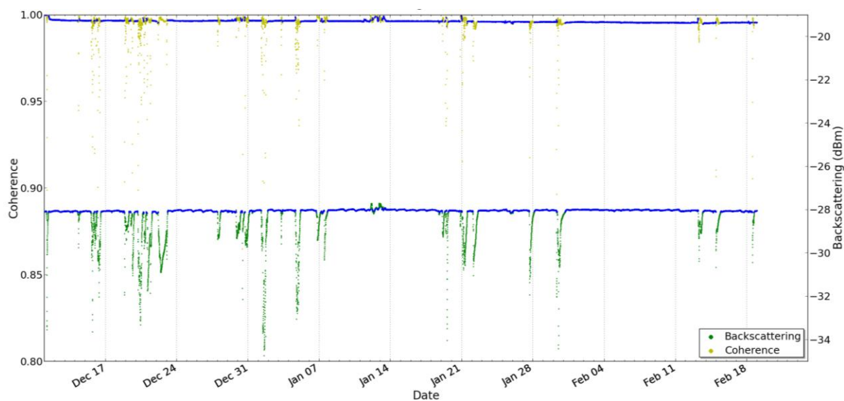
Figure 46. Coefficient de rétrodiffusion et cohérence du couplage pour TS-WINTER ; les données filtrées conservées sont indiquées en bleu.
