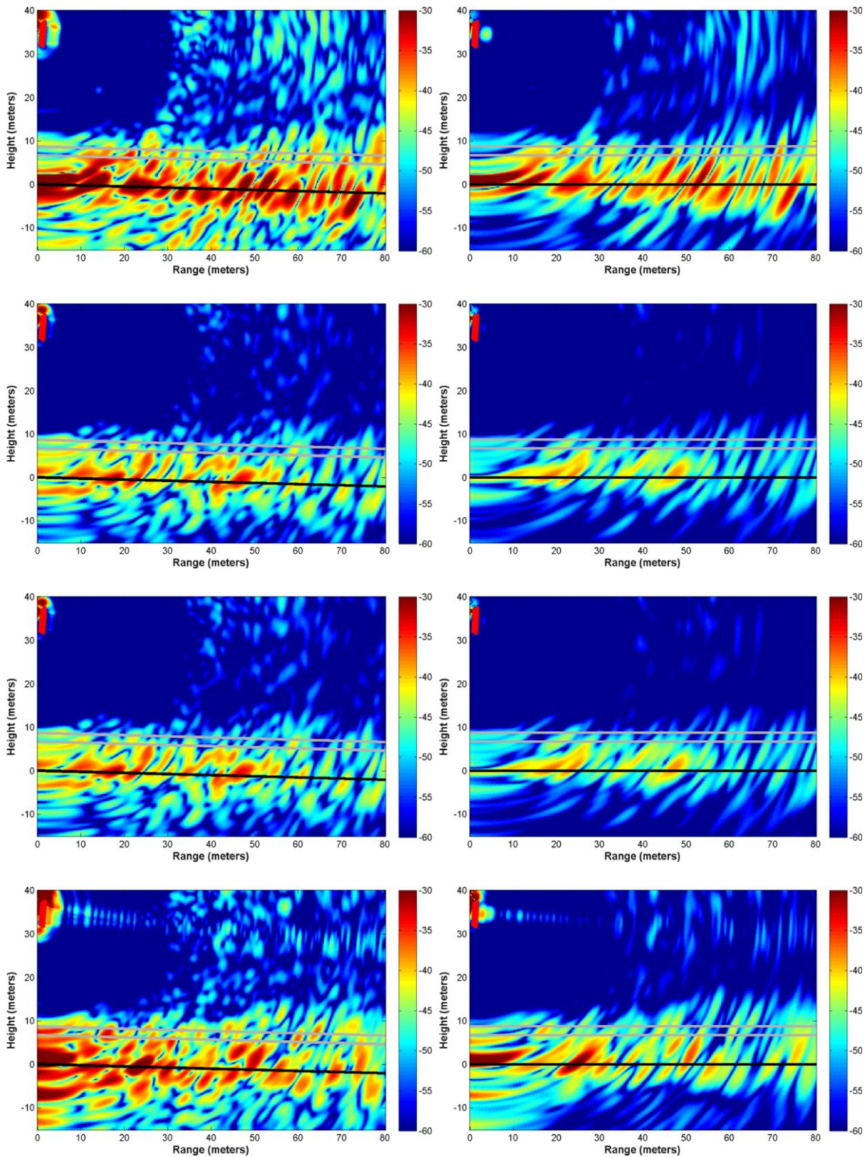
Figure 70. Tomogrammes bruts de P8 (gauche) puis avec apodisation et correction de la pente (droite) pour les polarisations, de haut en bas, HH, HV, VH et VV. Les positions des antennes sont
