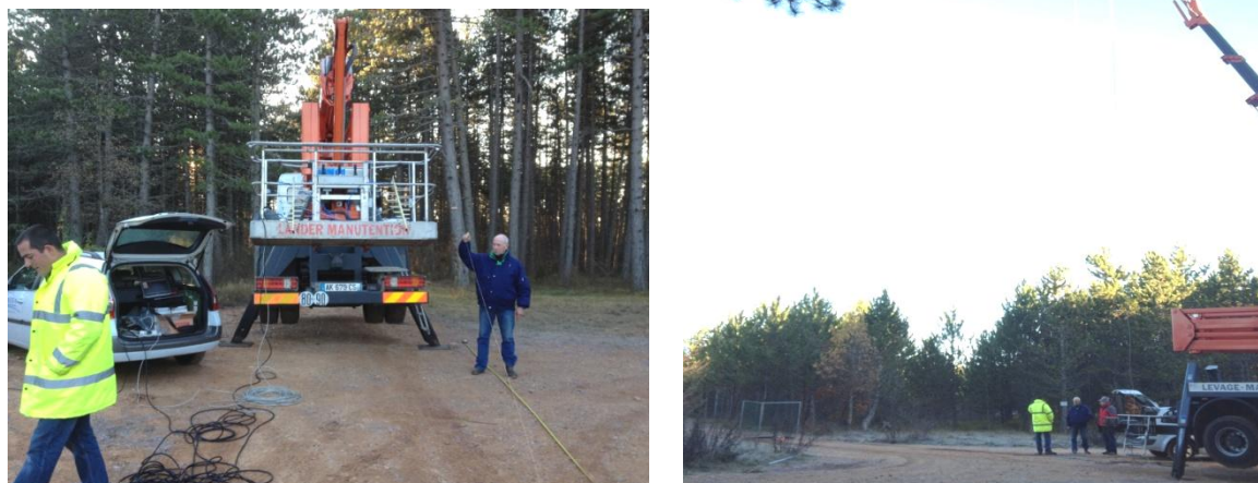
Figure 24. PC de pilotage dans le coffre de la voiture et nacelle équipée du VNA et des antennes (gauche) et mesure de validation du système d'acquisition à l'aide d'un réflecteur radar (droite).
