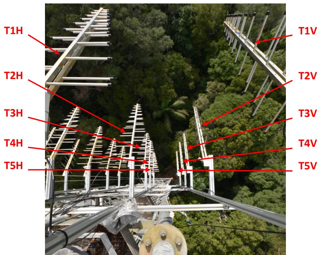
Figure 49. Montage sur la tour des antennes correspondant à la transmission des polarisations en H et V.
