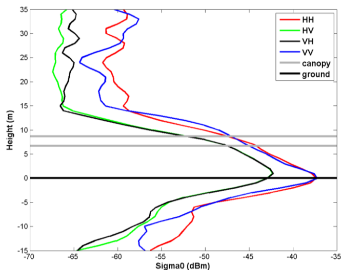
Figure 71. Profils verticaux de rétrodiffusion de P8 obtenus à partir des tomogrammes avec apodisation.
