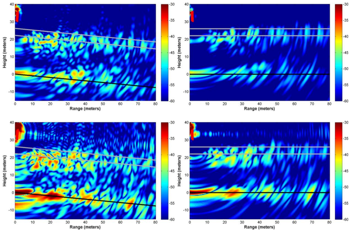
Figure 60. Tomogrammes bruts de P3 (gauche) puis avec apodisation et correction de la pente (droite) pour les polarisations, de haut en bas, HH, HV, VH et VV. Les positions des antennes sont dessinées en rouge en haut à gauche, le niveau du sol en noir, et les mesures de hauteur de la canopée en gris.
