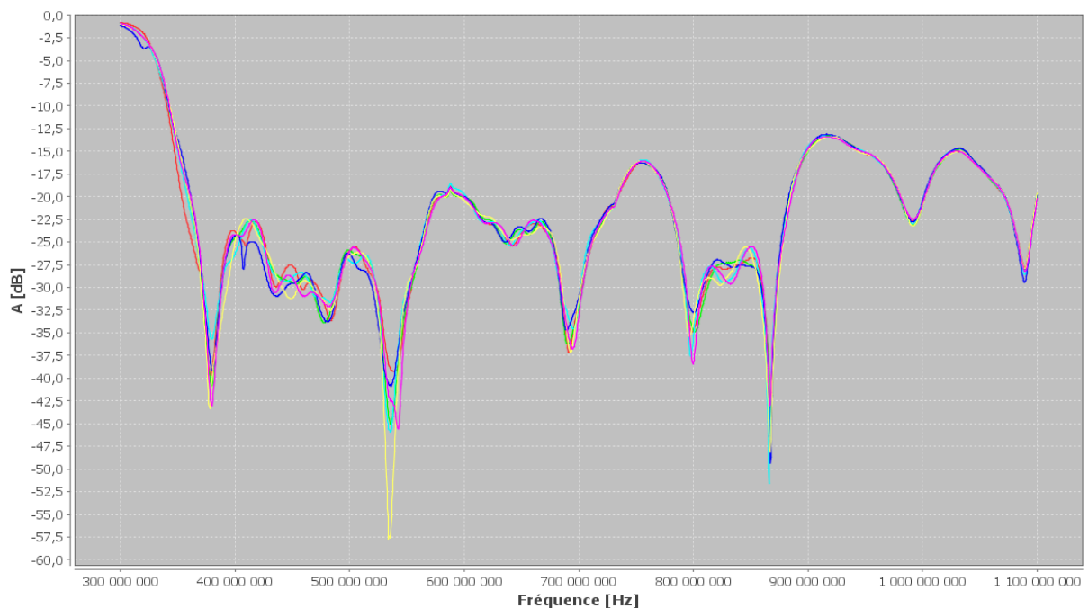
Figure 43. Perte de retour d'une antenne avec couplage inclus, c.à.d. pour les polarisations HH ou VV (S11 ou S22) ; la mesure pour une antenne seule est donné en bleu, et celles correspondant à un espacement de 30 à 70 cm, respectivement de bleu foncé à vert.
