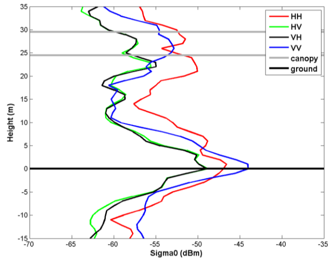
Figure 67. Profils verticaux de rétrodiffusion de P6 obtenus à partir des tomogrammes avec apodisation.
