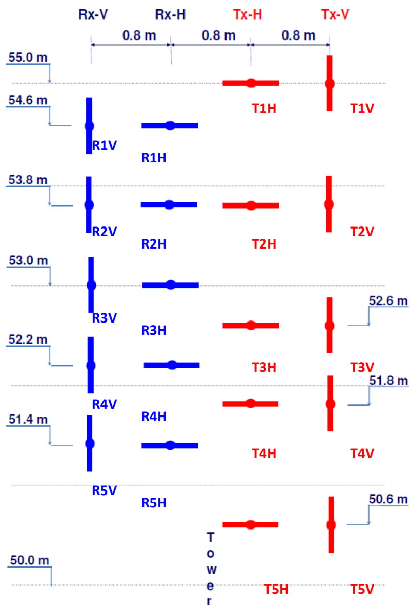
Figure 48. Vue d'arrière du réseau d'antenne monté sur la tour. Les termes « R » et « T » correspondent respectivement aux voies de réception et de transmission, et les termes H et V à la polarisation horizontale ou verticale de l'antenne.
