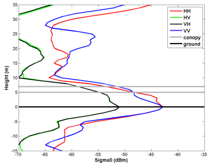
Figure 53. Profils verticaux de rétrodiffusion de P0 obtenus à partir des tomogrammes avec apodisation.
