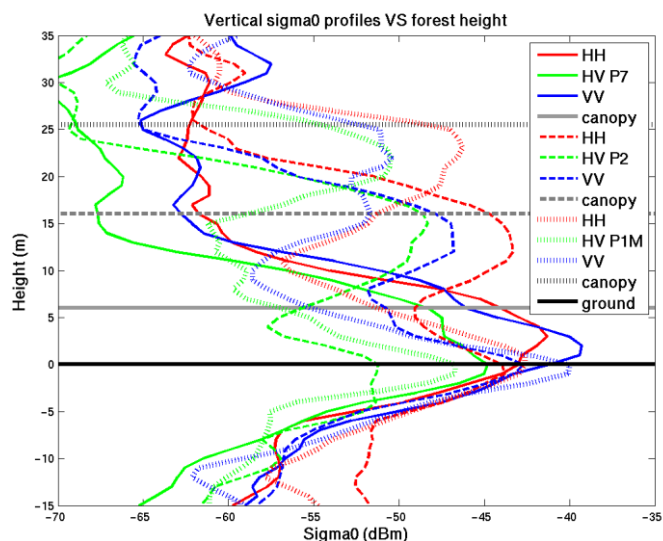
Figure 74. Profils verticaux de rétrodiffusion de P7, P2 et P1M.
