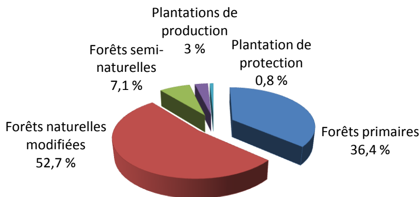
Figure 4. Caractéristiques des forêts du monde [FAO, 2005].
