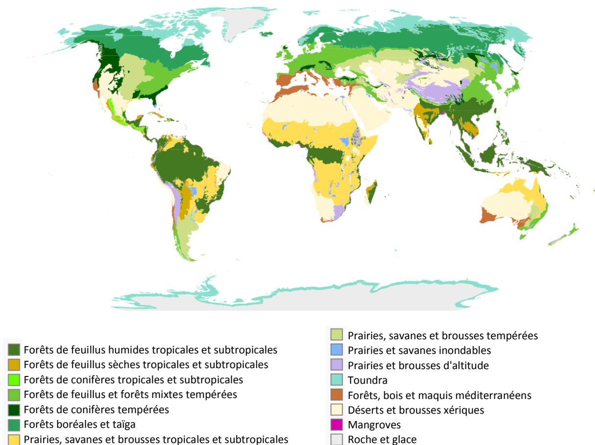
Figure 3. Répartition des principaux biomes terrestres à l'échelle du globe [WWF, 2006].
