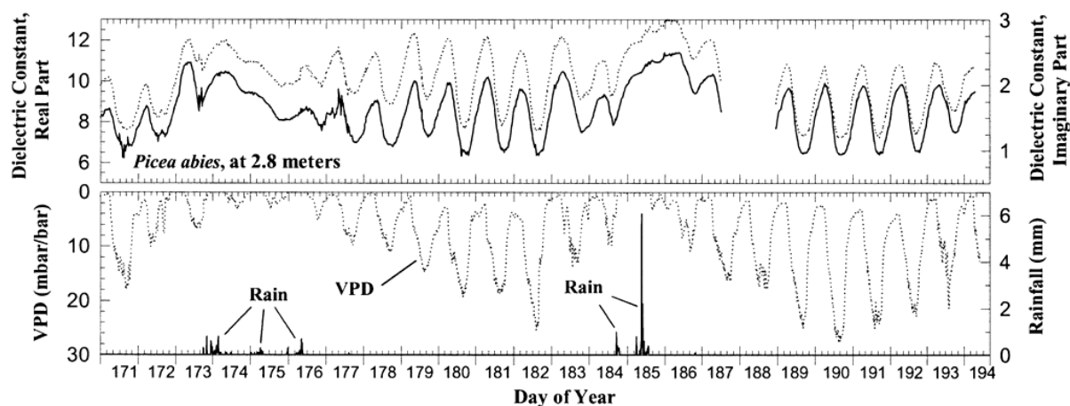
Figure 13. Série temporelle sur 23 jours de 1995 de constante diélectrique en bande P de troncs d'épicéas. Le Déficit en Pression de Vapeur (VPD) et la pluviométrie (en millimètre toutes les 10 minutes) sont aussi traces [Mc Donald et al., 2002].
