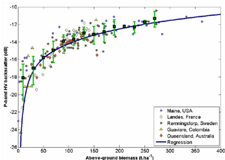
Figure 10. Courbe de l'intensité du canal HV en bande P en fonction de la biomasse [ESA, 2008]
