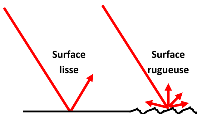
Figure 7. Interaction spéculaire (surface lisse) et diffuse (surface rugueuse) d'une surface.
