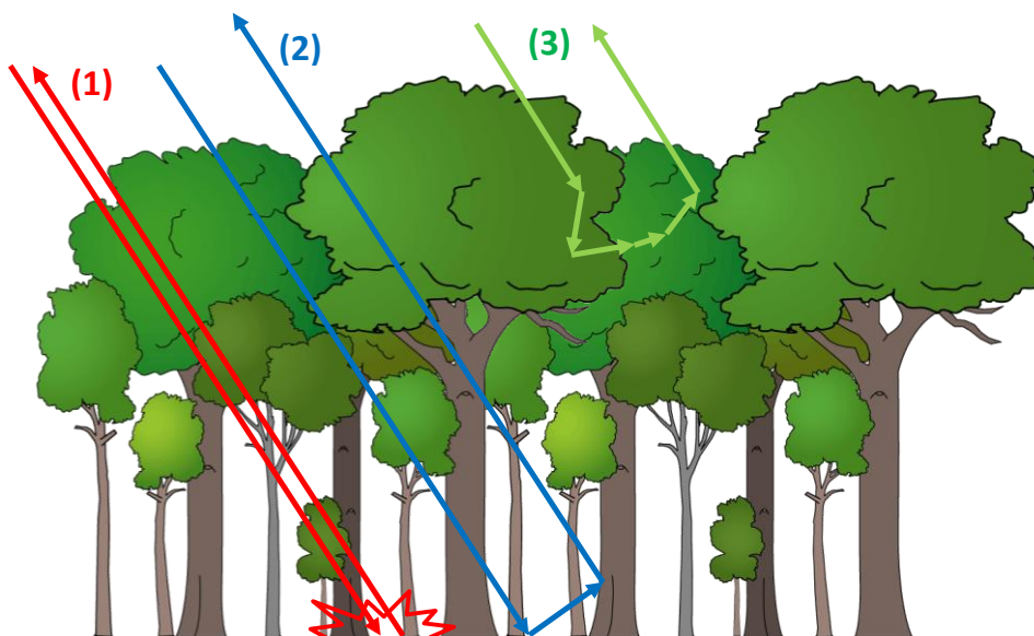
Figure 6. Principaux mécanismes intervenant dans la rétrodiffusion radar d'une forêt : interactions de surface (1), interactions de double-rebond (2) et interactions de volume (3).
