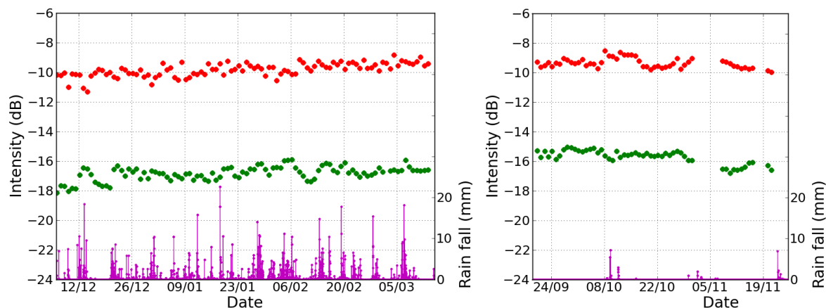
Figure 36. Séries temporelles des coefficients de rétrodiffusion HH (rouge) et HV (vert) acquis à 6:00 avec l'expérimentation TropiScat, sur la forêt complète, pour la saison humide (gauche) et pour la saison sèche (droite).
