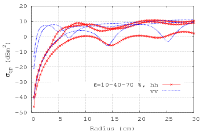
Figure 8. Coefficient de rétrodiffusion radar en bande P d'un cylindre en fonction de son diamètre et de son humidité [Borderies et al., 2009].
