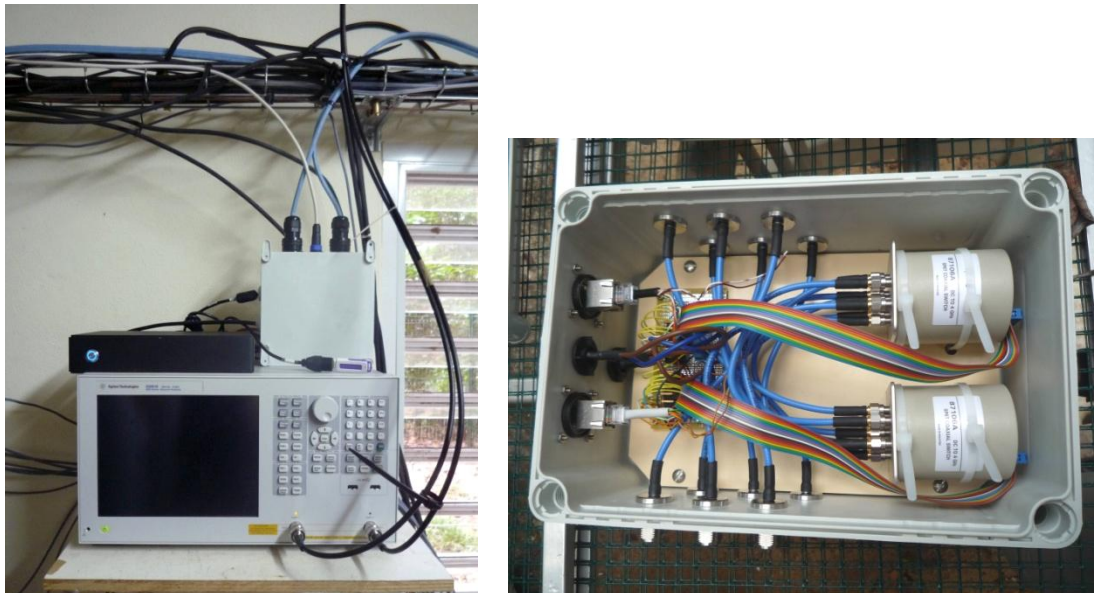
Figure 16. TropiScat : PC de pilotage en noir, VNA et boîtier blanc de pilotage des commutateurs au pied de la tour (gauche) et intérieur d'un boîtier de commutation (droite).
