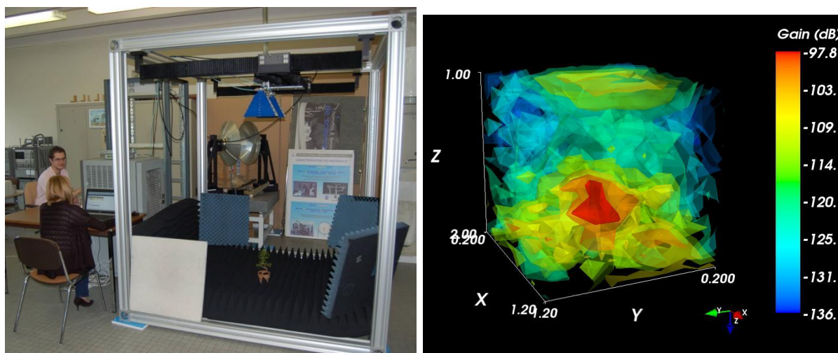
Figure 31. Etudiants, positionneur 2D et bonzaï durant une mesure (gauche), et tomogramme 3D obtenu (droite).
