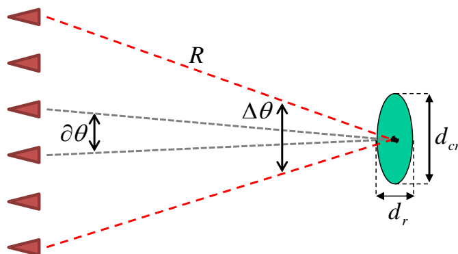
Figure 23. Schéma représentant le réseau virtuel formé par les points de mesures (en rouge) et la réponse d'une cible ponctuelle (en vert).
