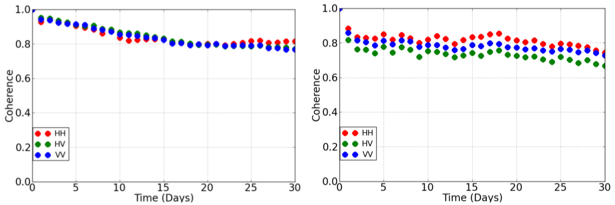
Figure 39. Evolution de la cohérence temporelle en fonction de la baseline temporelle pour la saison sèche (gauche) et pour la saison des pluies (droite).
