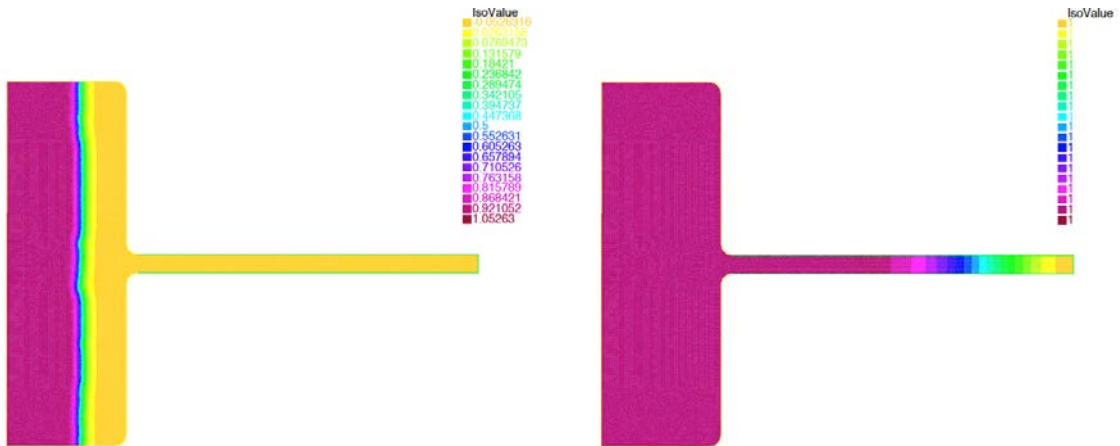
FIGURE 5 – Dans le cas d'un cylindre qui se rétrécit, l'onde se propage dans tout le domaine. De gauche à droite : valeur de la solution u pour différentes valeurs de t croissantes. Dans les parties jaunes la solution est proche de 0 et dans les parties violettes la solution est proche de 1
