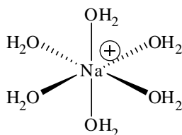
Figure 1.1 : Exemple d'interaction ion-dipôle entre un cation \text{Na}^+ et des molécules d'eau
