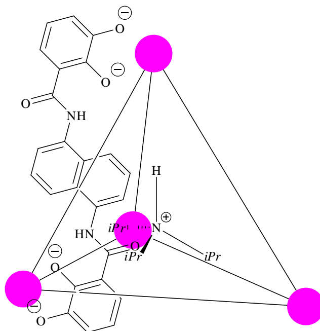
Figure 1.5 : Exemple d'assemblage supramoléculaire encapsulant un ammonium. Les points rose représentent les cations Ga^{3+}
