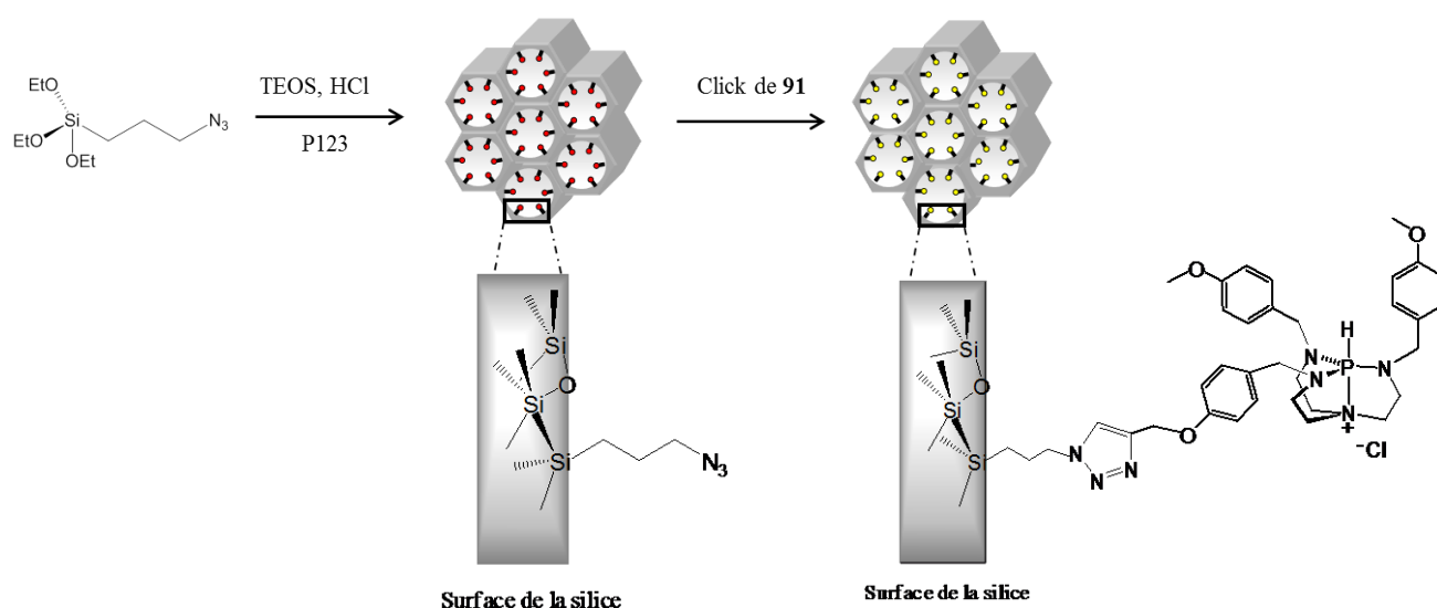
Figure 3.28 : Synthèse de la silice mésoporeuse SBA-15 fonctionnalisée par des groupements azidopropyle et greffage de l'azaphosphatane 91 par réaction de « click chemistry »
