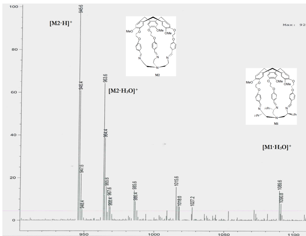
Figure 2.59 : Spectres de masse montrant la présence des deux hémicyptophanes imine après ajout du tren achiral (haut) et ajout d'un large excès du tren achiral
