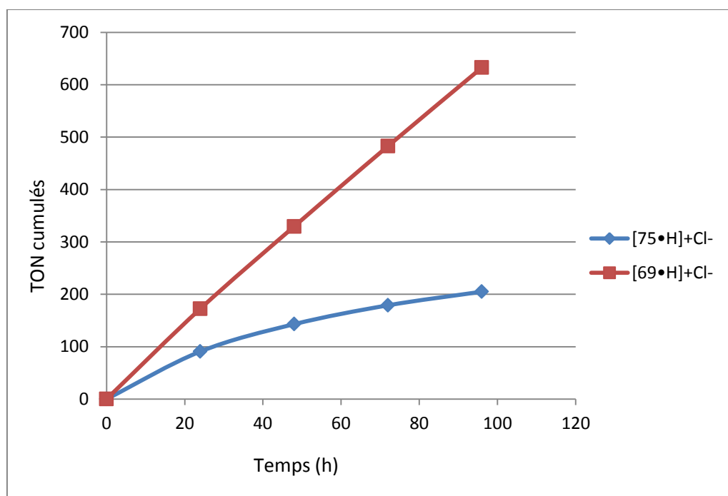
Figure 3.19 : Comparaison des performances des catalyseurs [\mathbf{69}\cdot\mathbf{H}]^+\text{Cl}^- et [\mathbf{75}\cdot\mathbf{H}]^+\text{Cl}^- . Conditions : SO (50mmol), catalyseur (0,05 mmol), \text{CO}_2 (1 atm.), 100^\circ\text{C} . Les TON ont été déterminés par RMN ^1\text{H} en utilisant le 2,4-dibromomésitylène comme étalon interne (2 mmol)
