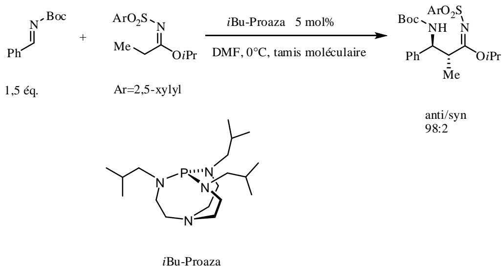
Figure 1.44 : R\u00e9action de type Mannich entre une imine et un sulfonylimidate
