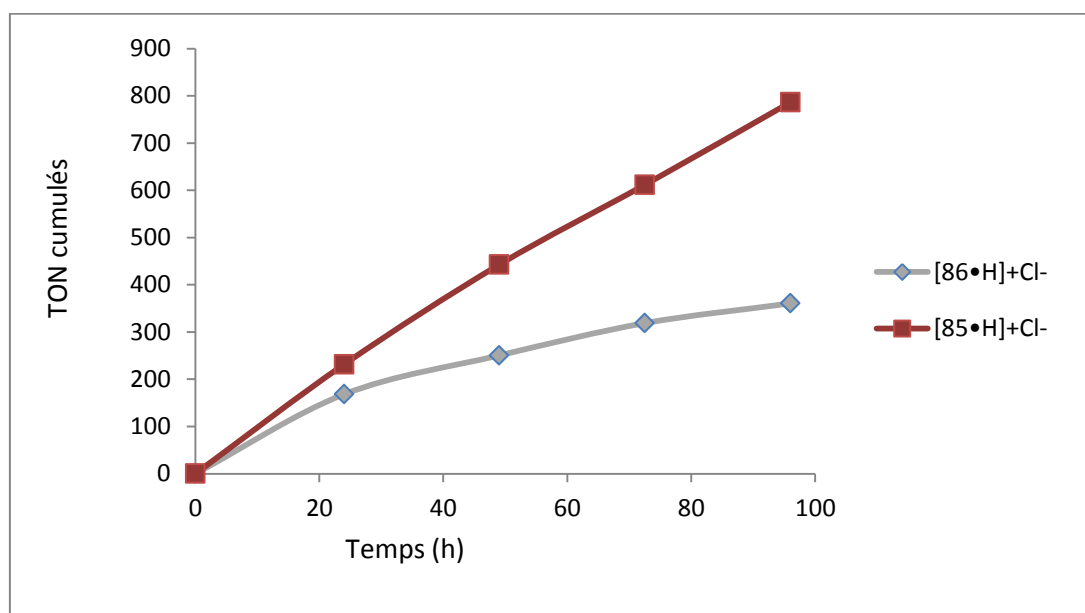
Figure 3.22 : Comparaison des performances des catalyseurs [85 \cdot H]^+ Cl^- et [86 \cdot H]^+ Cl^- . Conditions : SO (50mmol), catalyseur (0,05 mmol), CO_2 (1 atm.), 100^\circ C . Les TON ont été déterminés par RMN ^1H en utilisant le 2,4-dibromomésitylène comme étalon interne (2 mmol)
