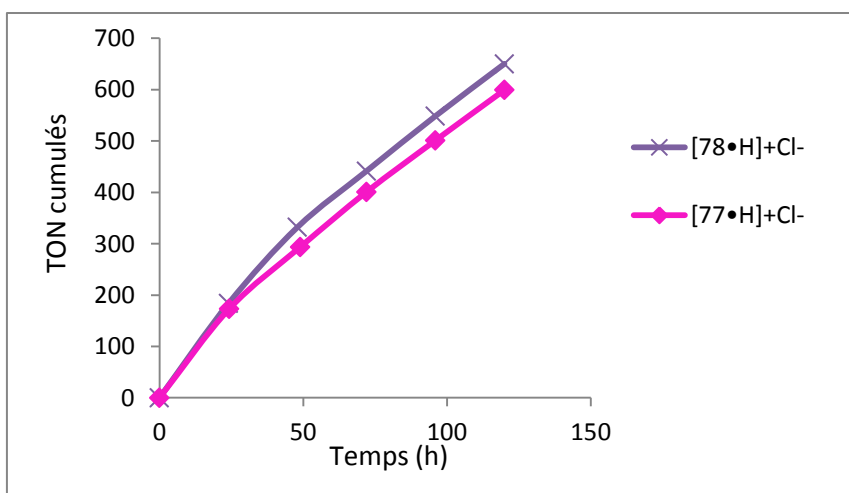
Figure 3.25 : Comparaison des performances des catalyseurs [77·H] + Cl - et [78·H] + Cl - . Conditions : SO (50mmol), catalyseur (0,05 mmol), CO 2 (1 atm.), 100°C. Les TON ont été déterminés par RMN 1 H en utilisant le 2,4-dibromomésitylène comme étalon interne (2 mmol)
