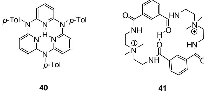
Figure 2.1 : Exemples de macrocycles complexant des protons
