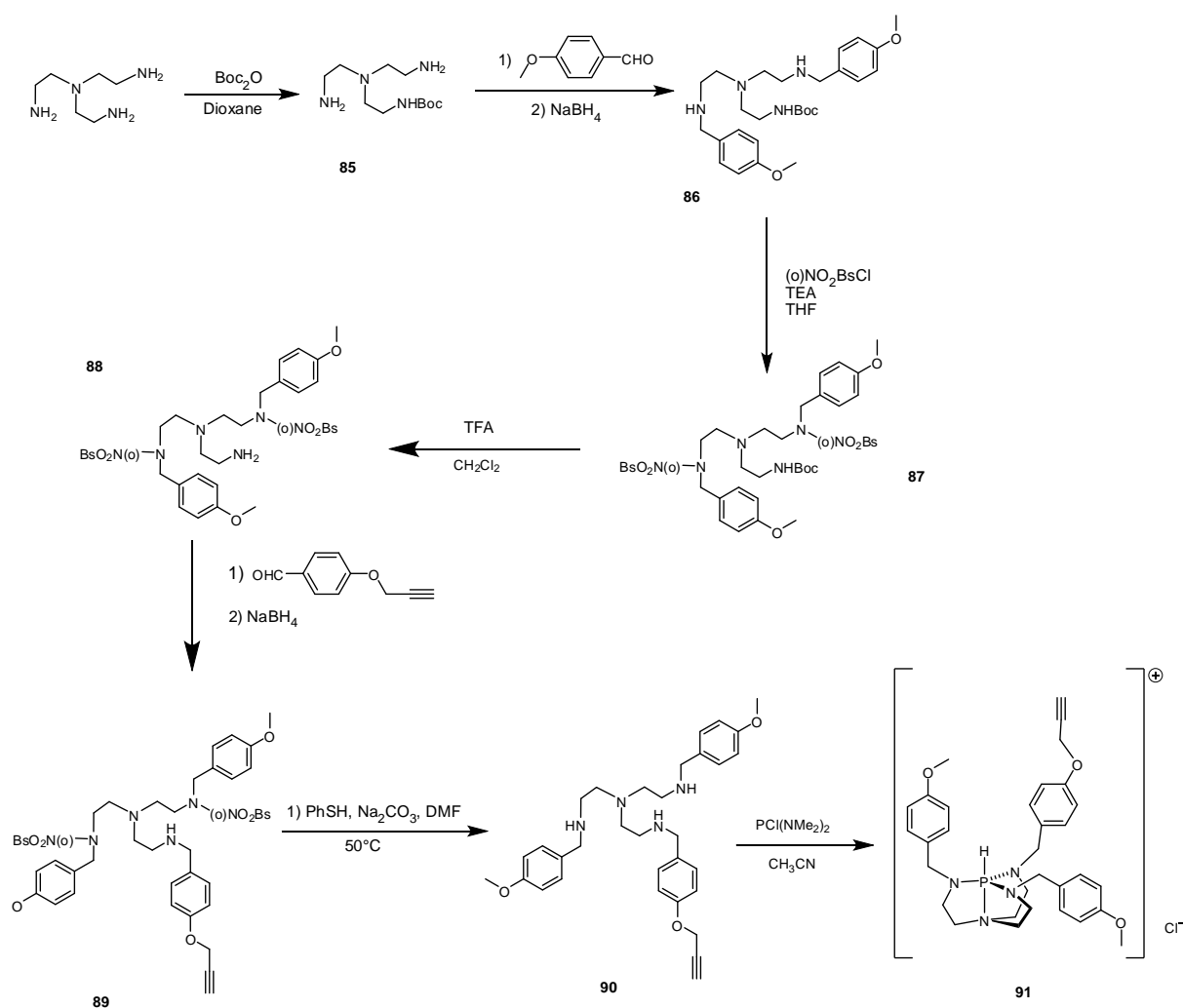
Figure 3.27 : Voie de synthèse permettant d'accéder à l'azaphosphatrane désymétrisé possédant un bras propargyle
