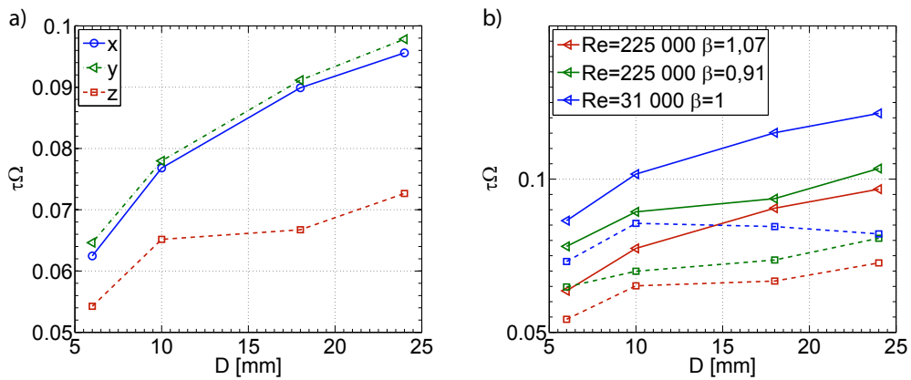
FIGURE III.24 – a) Temps de corrélation (définis par l'intégrale jusqu'au passage à 50%) de la vitesse fluctuante pour des particules légères dans l'eau à \Omega = 4 Hz en fonction de leur diamètre et selon les trois composantes. b) Temps de corrélation de la vitesse fluctuante pour les différentes densités et Reynolds en fonction du diamètre, selon la composante axiale et la composante transverse moyenne ( \tau_v^t = (\tau_v^x + \tau_v^y)/2 ).
