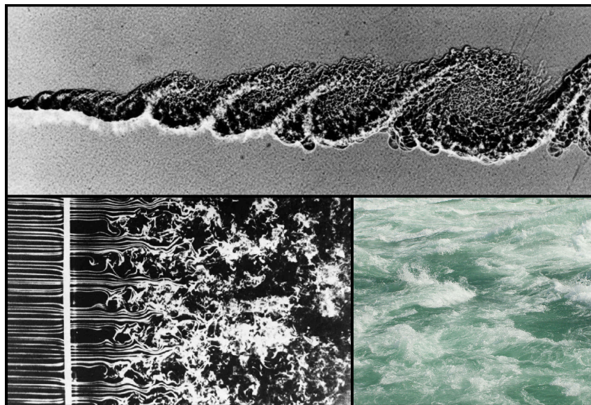
FIGURE I.1 – En haut : Couche de mélange entre deux gaz allant à des vitesses différentes (1 et 0,4 \text{ m}\cdot\text{s}^{-1} ). En bas à gauche : écoulement derrière une grille (1 cm de pas de maille) à Re = 1500 . Ces deux premières images sont issues de An Album of Fluid Motion [73]. En bas à droite : photographie de la rivière Niagara peu après les chutes.
