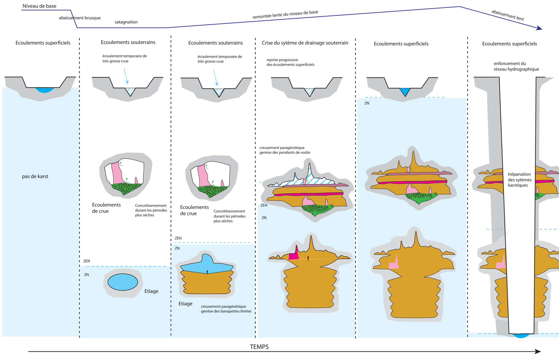
Figure 5.74 Hypothèses d'évolution spéléogénique du secteur d'étude en relation avec la structuration du réseau de drainage superficiel.
