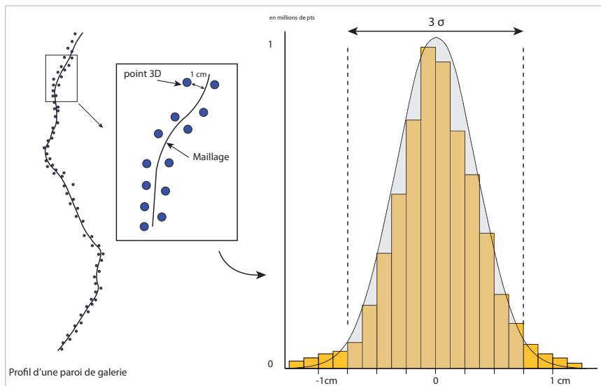
Figure 5.10 Le contrôle géométrique de ce modèle TIN (triangulated irregular network), pour vérifier sa conformité vis-à-vis du terrain, a été réalisé en calculant (1) l'écart type du nuage de point par rapport au modèle triangulé et (2) au moyen de profils topographiques si les triangles se situaient bien au milieu du nuage de points. Sur la carte des écarts du nuage de points, autant de points du nuage se situent de part et d'autre le plan du maillage. Le nuage de points est entaché d'un bruit gaussien.
