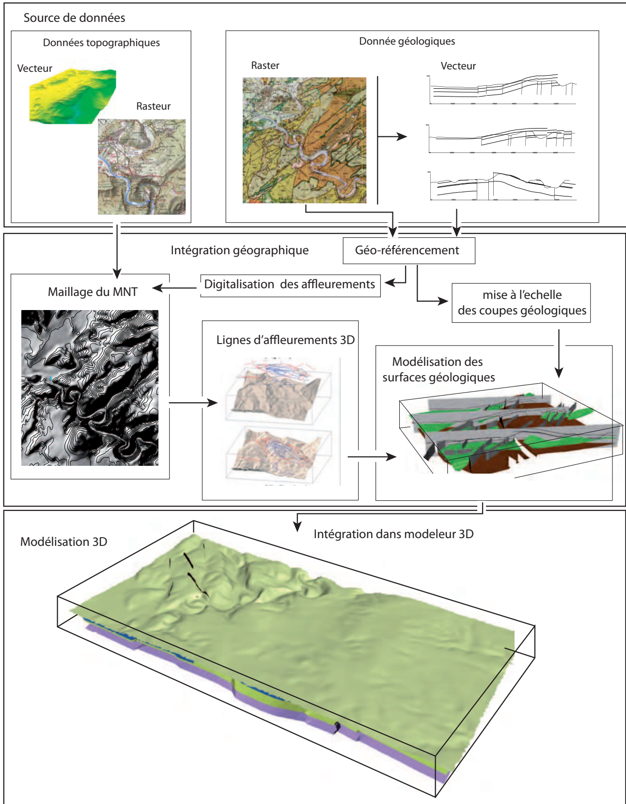
Figure 2.8 Organigramme de la méthodologie utilisée pour la construction du modèle géologique 3D.
