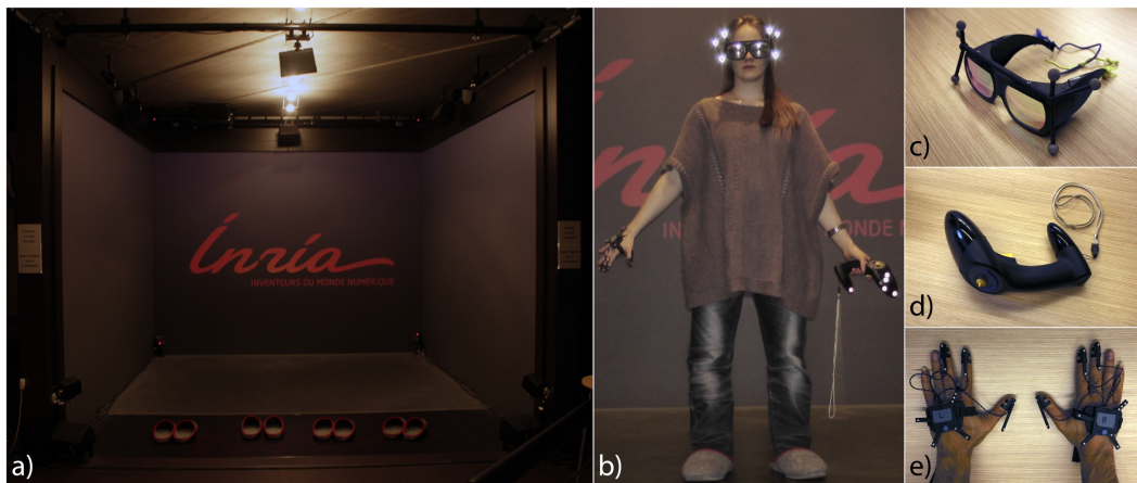
Figure B.1: Installation expérimentale. Le cube immersif est visible en a) avec huit caméras infrarouges et un système de son spatialisé. Au milieu, b) un utilisateur porte les appareils détectés: c) les lunettes Infitec avec balises, d) la manette ART et e) les gants ART de suivi des doigts.
