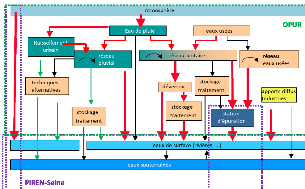
Figure 2 : cycle de l'eau en milieu urbain (Bertrand-Krajewski, communication personnelle)
