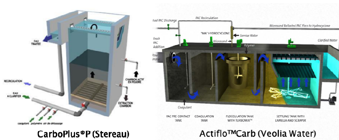
Figure 15 : technologies prochainement étudiées (CarboPlus®P et Actiflo™Carb)
