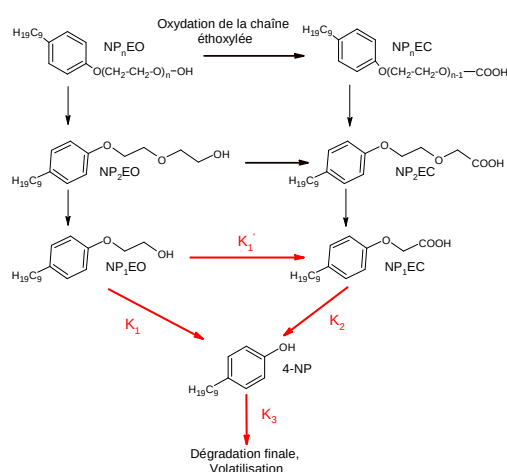
Figure 17 : mécanismes réactionnels considérés dans le modèle ProSe (en rouge) et linéaire de Seine considéré pour le suivi de masse d'eau
