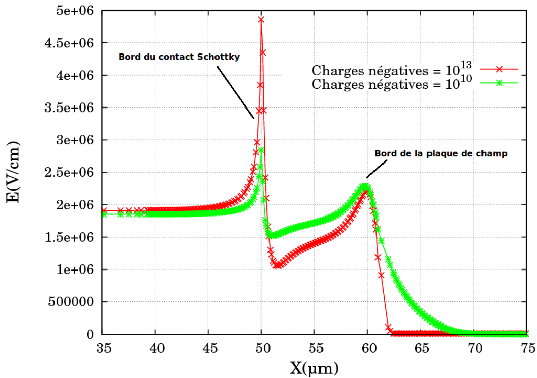
FIGURE 2.25 – Répartition du champ électrique selon l’axe AA’ pour la même tension qui correspond au claquage dans le cas de 10^{13} charges.cm -2 .
