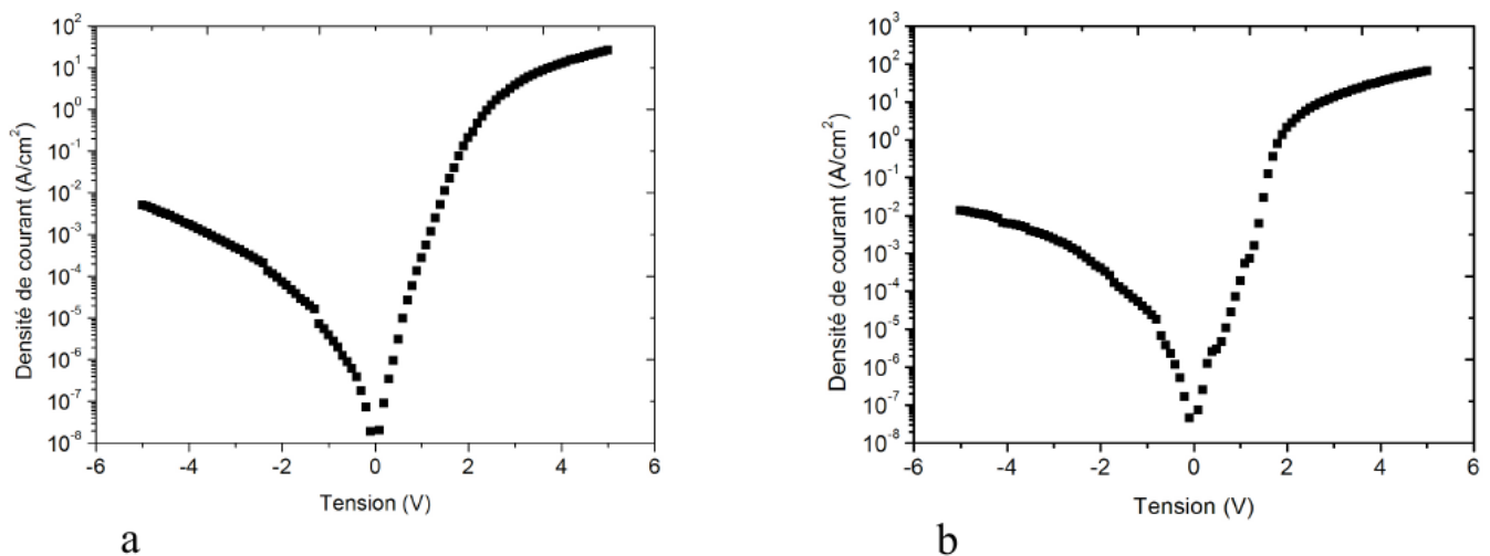
FIGURE 4.18 – Caractéristique I(V) d'une diode Schottky verticale Ni/diamant à température ambiante (a) B90, zone p^+ dopée à 3.10^{19} \text{ cm}^{-3} et (b) B92, zone p^+ dopée à 3.10^{20} \text{ cm}^{-3} tiré de [94].
