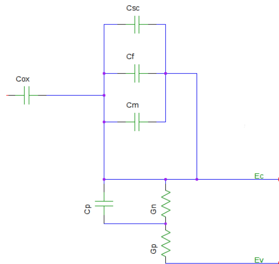
FIGURE 3.13 – Modèle équivalent complet d'une structure MOS avec tous les types de défauts. Un seul niveau d'énergie de piège à l'interface est considéré pour simplifier.
