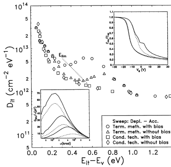
FIGURE 3.35 – Distribution des états d’interface dans le gap de SiC selon les travaux de Berberich et al. [136].
