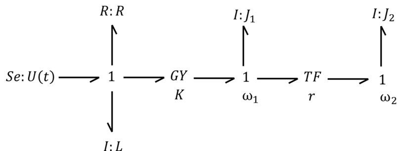
Figure 61. Bond graph acausal du moteur associé au réducteur
