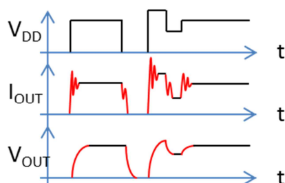
Figure 92. Exemple de comportements analogiques dans les systèmes numériques
