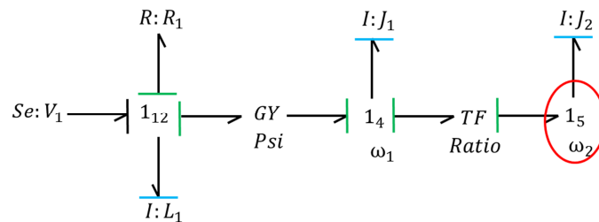
Figure 78. Bond graph non causal obtenu au premier tour
