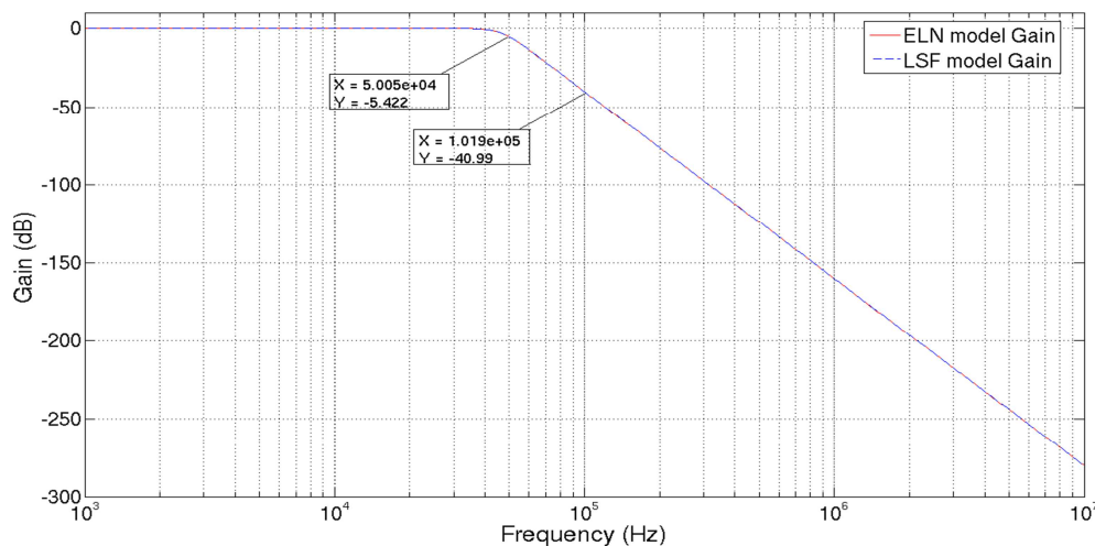
Figure 24. Diagramme de gain du circuit comparé à la fonction de transfert de départ.
