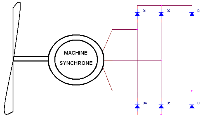
Figure 85. Schéma de principe de l'éolienne
