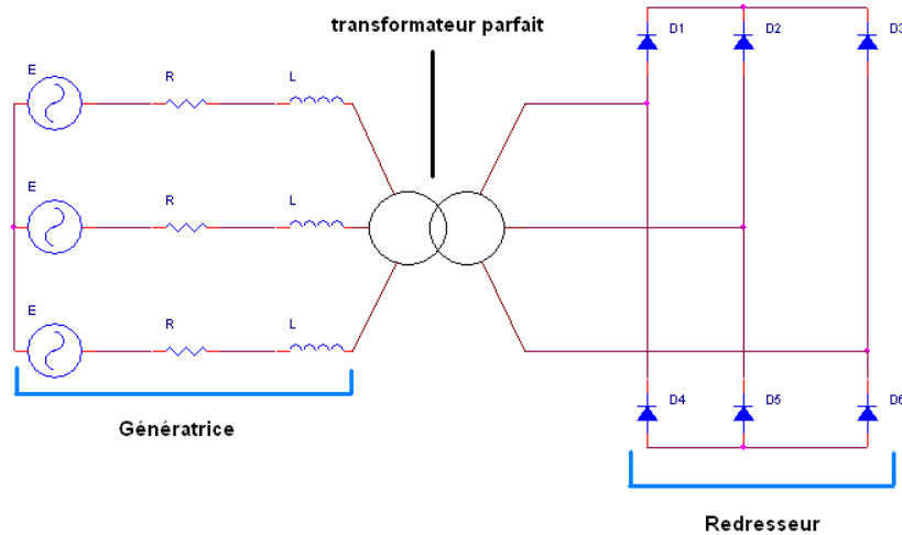
Figure 87. Schéma détaillé de la partie électrique de l'éolienne
