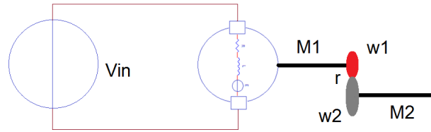
Figure 59. Moteur électrique à courant continu couplé à un réducteur
