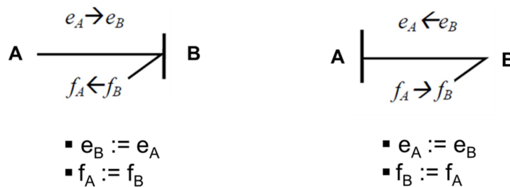
Figure 62. Les deux cas possibles de causalité
