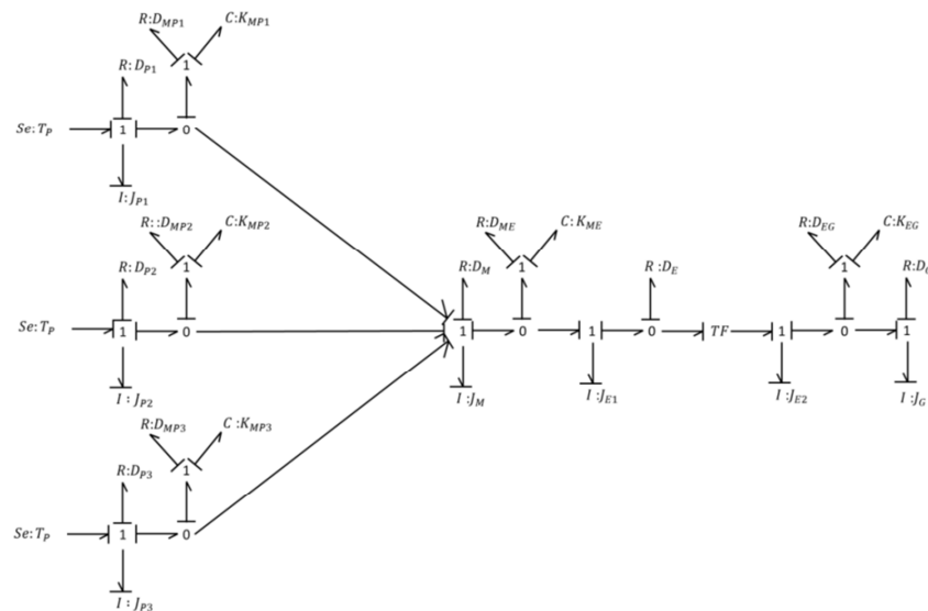
Figure 88. Bond graph de la partie linéaire du système
