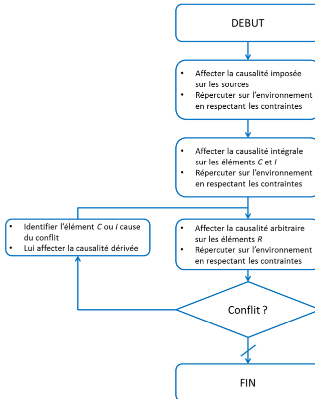
Figure 63. Procédure d'affectation de la causalité
