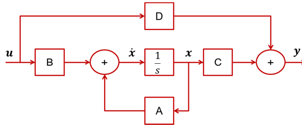
Figure 27. Diagramme schéma-bloc d'un système linéaire dynamique
