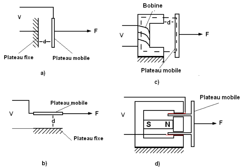
Figure 41. Différents types de transducteurs électromécaniques
