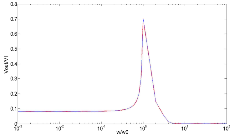
Figure 48. Comparaison entre le modèle LSF et le modèle ELN du filtre électromécanique
