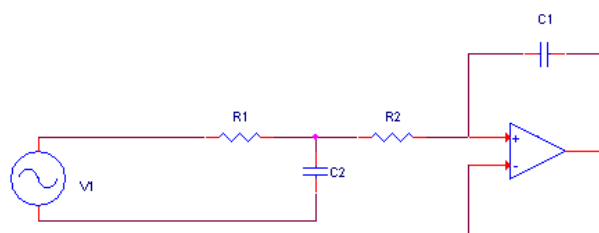
Figure 22. Schéma d'une cellule de Sallen Key du second ordre
