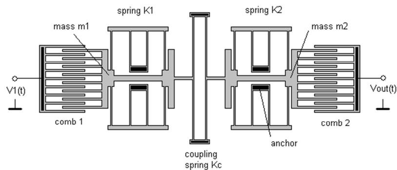
Figure 46. Filtre électromécanique constitué par une association de deux micro-résonateurs
