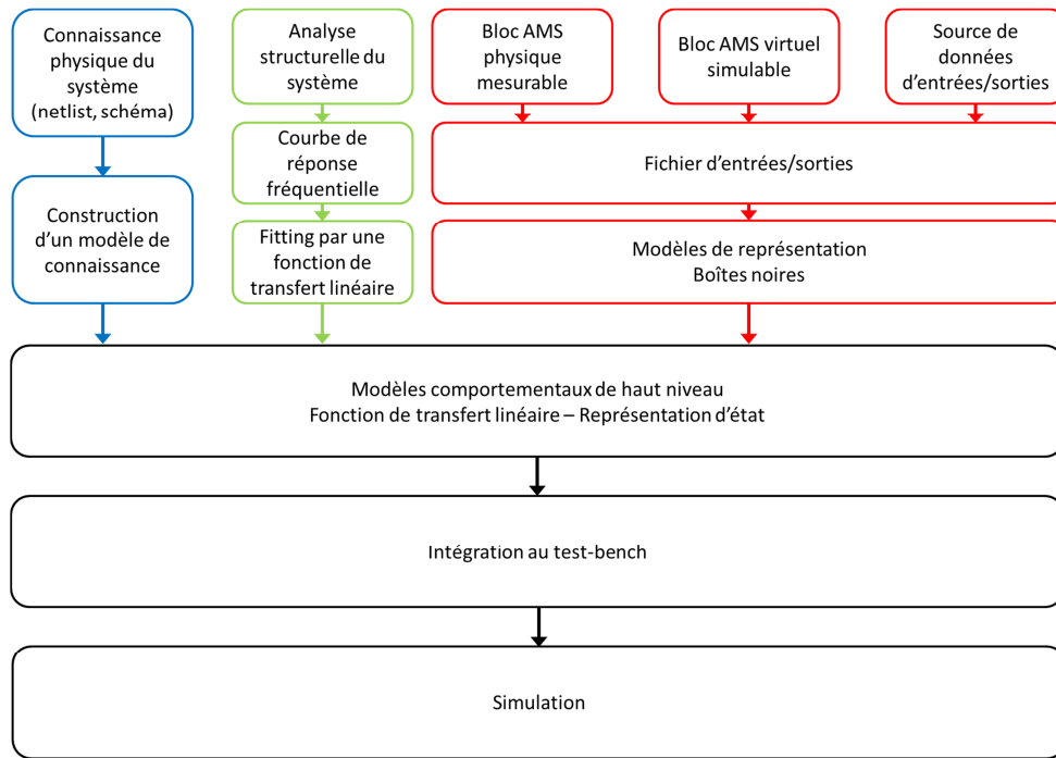
Figure 2. Travaux menés à TIMA sur la modélisation AMS à haut niveau
