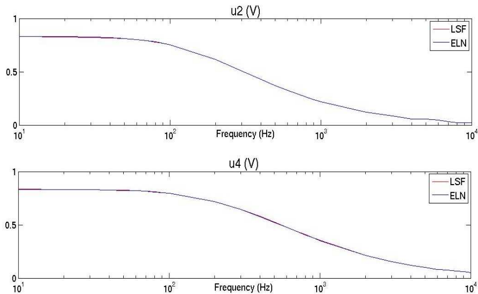
Figure 33. Comparaison LSF/ELN pour le filtre du quatrième ordre
