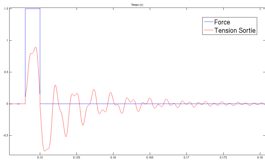
Figure 55. Simulation du capteur de force (zoom)
