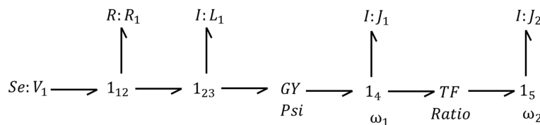
Figure 76. Bond graph du motoréducteur après la 2 nde partie de la 1 ère étape de la simplification
