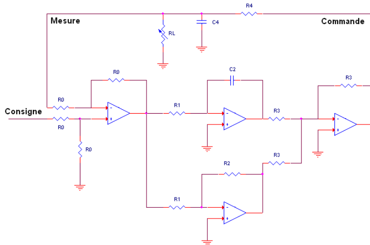
Figure 17. Modèle ELN du four
