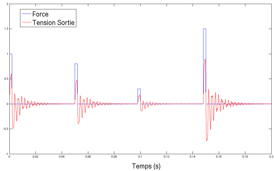
Figure 54. Simulation du capteur de force
