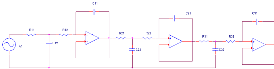
Figure 23. Filtre réalisant la fonction de transfert définie par le Tableau 7
