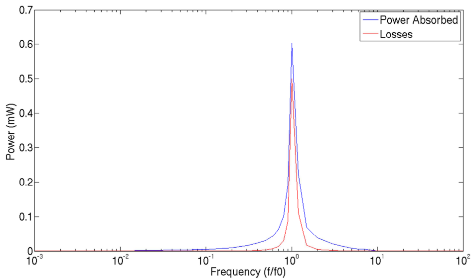
Figure 50. Bilan des puissances du filtre électromécanique
