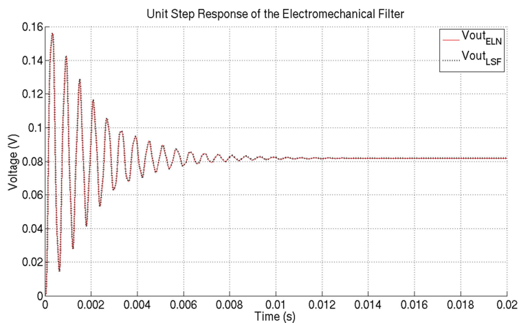
Figure 48. Comparaison entre le modèle LSF et le modèle ELN du filtre électromécanique
