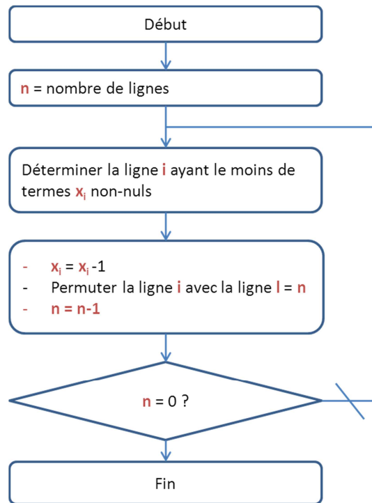
Figure 29. Algorithme des permutations de lignes
