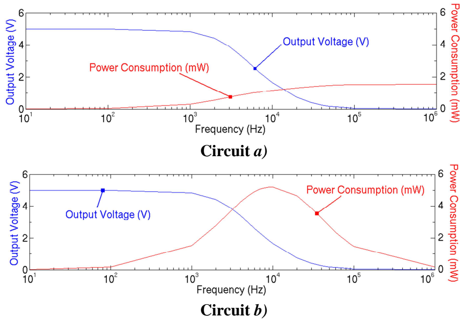
Figure 37. Comparaison tensions de sortie et puissances
