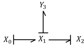
Figure 69. Bond graph déduit de la seconde ligne de la matrice BG
