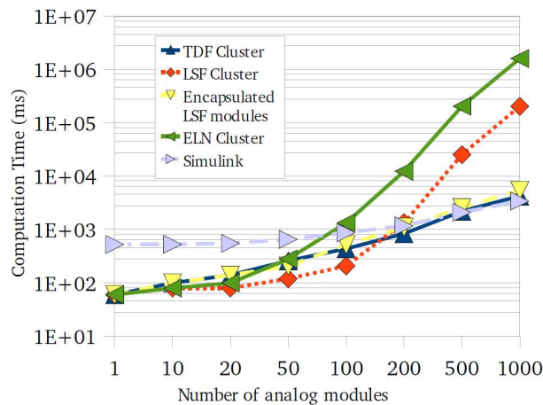
Figure 12. Durées d'élaboration et de simulation en fonction de l'ordre du filtre
