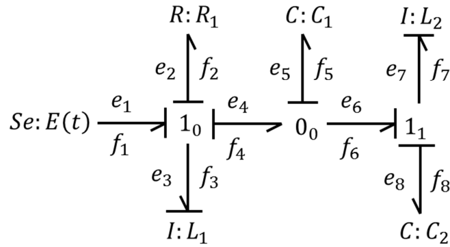
Figure 66. Bond graph simplifié de l'exemple
