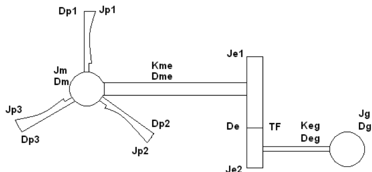
Figure 86. Schéma détaillé de la partie mécanique de l'éolienne
