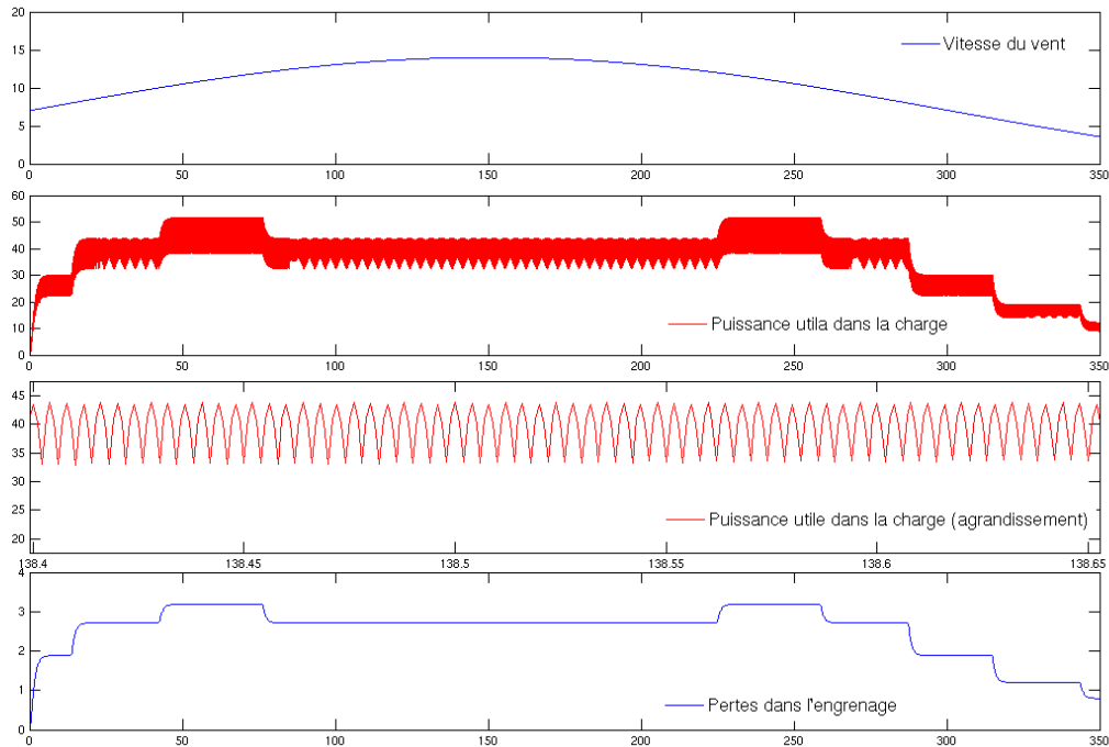
Figure 91. Simulation de l'éolienne – Aspects puissance
