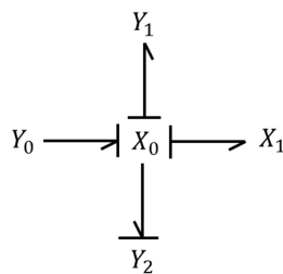
Figure 68. Bond graph déduit de la première ligne de la matrice BG
