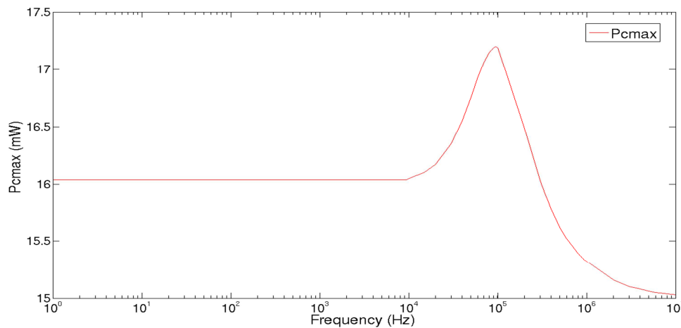
Figure 40. Consommation de puissance du filtre à variables d'état
