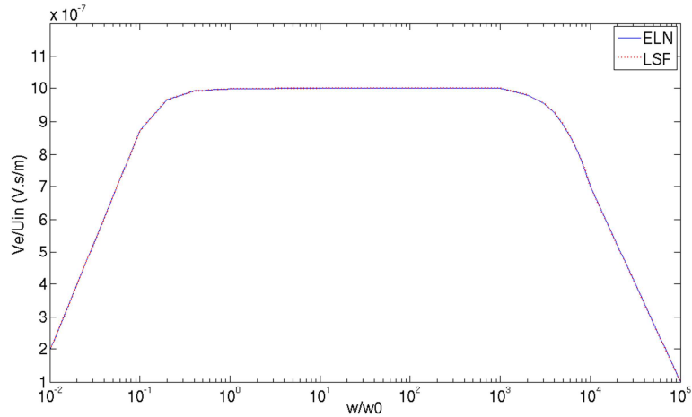
Figure 45. Comparaison entre le modèle LSF et le modèle ELN du capteur de vibrations
