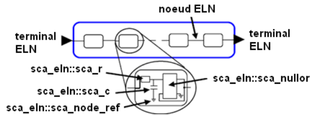
Figure 10. Modèle de filtre basé sur le MoC ELN
