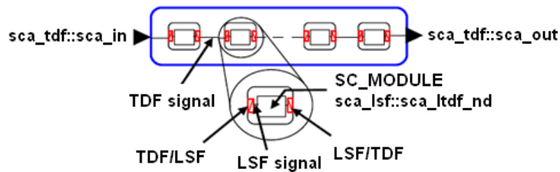
Figure 11. Modèle de filtre basé sur le style LSF encapsulé
