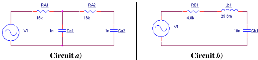
Figure 36. Deux topologies différentes pour un même comportement
