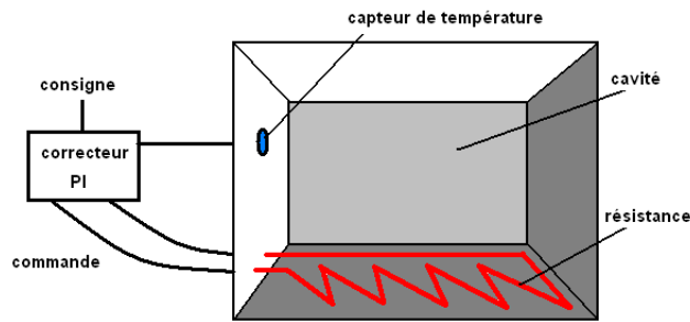
Figure 14. Modèle du Four
