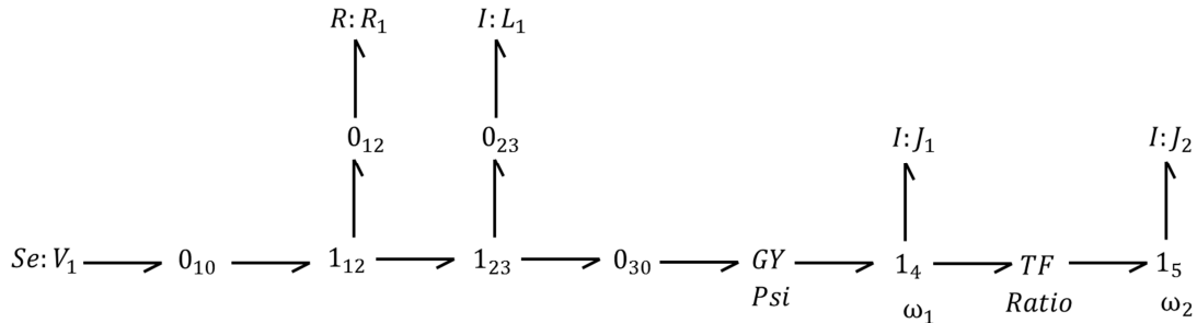
Figure 75. Bond graph du motoréducteur après la 1 ère partie de la 1 ère étape de la simplification
