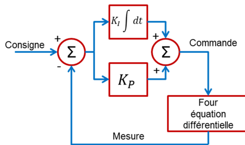
Figure 18. Modèle LSF encapsulé du four
