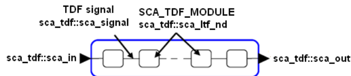
Figure 8. Modèle de filtre basé sur le MoC TDF
