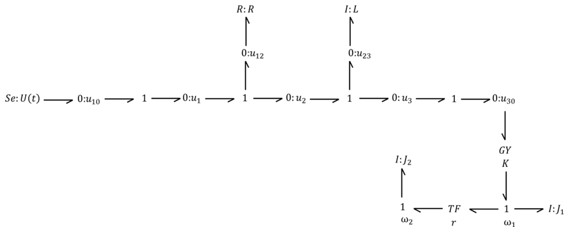
Figure 60. Bond graph non simplifié du moteur associé au réducteur
