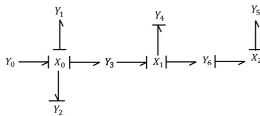
Figure 83. Bond graph global déduit à partir de la matrice BG du motoréducteur
