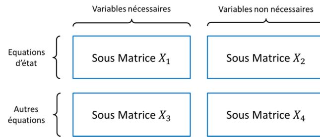
Figure 28. Les différentes sous matrices de la matrice du circuit
