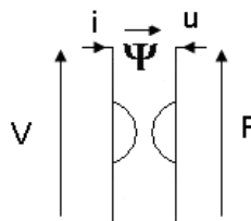
Figure 26. Schéma du gyrateur idéal
