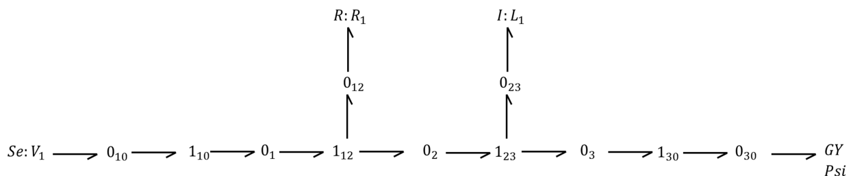
Figure 72. Bond graph de la partie électrique du système moteur-réducteur
