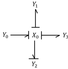
Figure 80. Bond graph déduit de la première ligne de la matrice BG du motoréducteur
