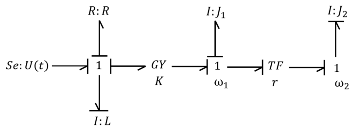
Figure 64. Bond graph causal du moteur associé au réducteur
