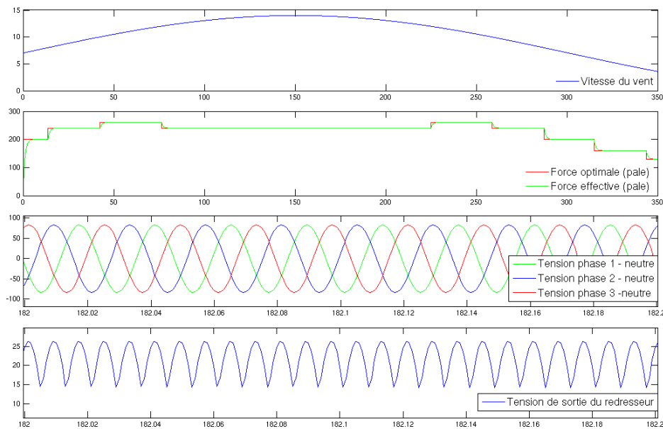
Figure 90. Simulation de l'éolienne - Comportement
