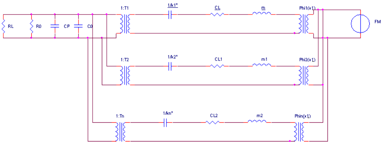
Figure 53. Circuit équivalent au capteur de force
