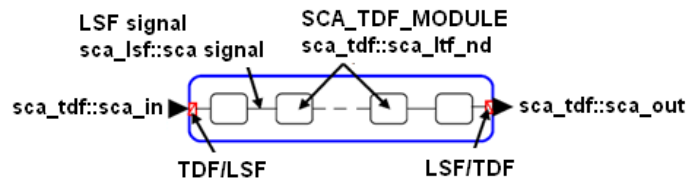
Figure 9. Modèle de filtre basé sur le MoC LSF
