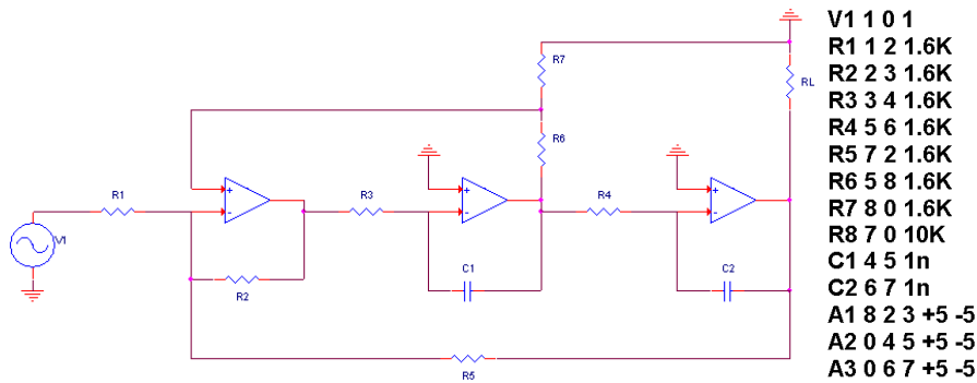
Figure 38. Filtre à variables d'état du second ordre et sa netlist
