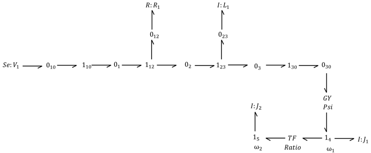
Figure 74. Bond graph non simplifié du système moteur-réducteur
