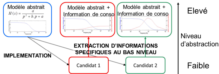
Figure 21. Méthode de raffinement et d'abstraction avec enrichissement
