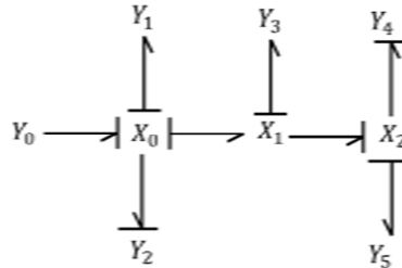
Figure 71. Bond graph global déduit à partir de la matrice BG
