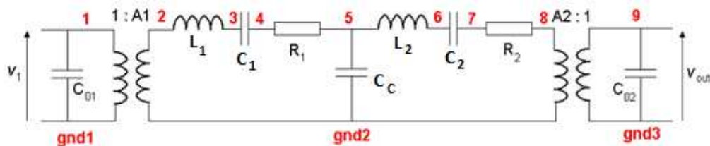
Figure 47. Filtre électromécanique constitué par une association de deux micro-résonateurs
