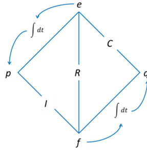
Figure 56. Tétraèdre de Paynter
