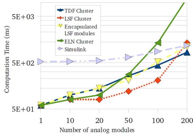
Figure 13. Durées d'élaboration et de simulation (zoom)
