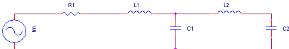
Figure 65. Exemple de circuit
