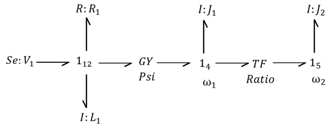
Figure 77. Bond graph du motoréducteur après la seconde étape de la simplification
