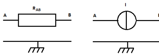
Figure 25. Une branche résistive et une source de courant
