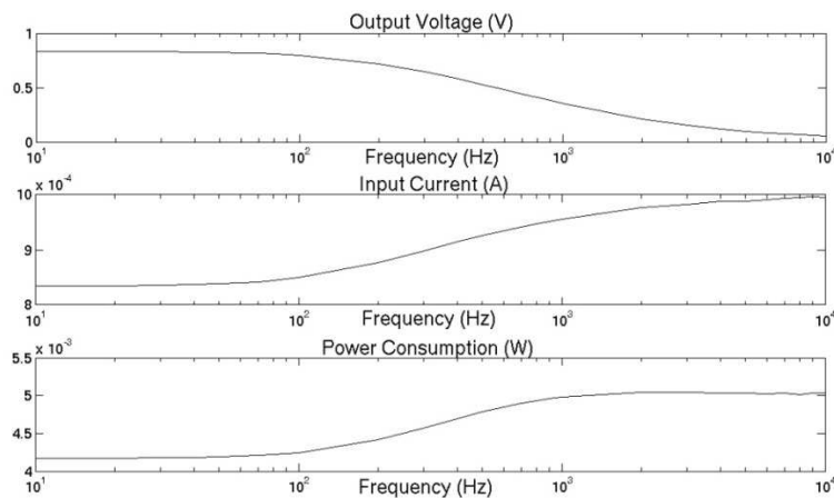
Figure 35. Tension de sortie, courant d'entrée et consommation du filtre d'ordre 4
