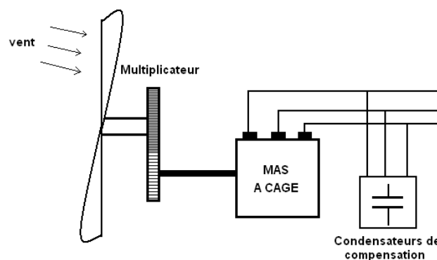
Figure 84. Eolienne à vitesse fixe basée sur un MAS à cage
