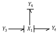
Figure 81. Bond graph déduit de la seconde ligne de la matrice BG du motoréducteur
