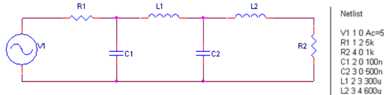
Figure 32. Filtre passif du quatrième ordre
