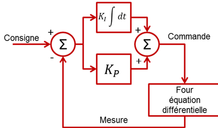
Figure 16. Modèle LSF du four
