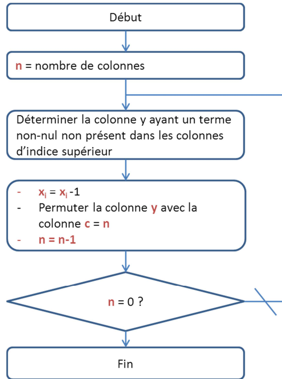
Figure 30. Algorithme des permutations de colonnes
