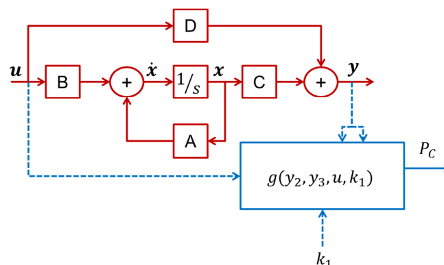
Figure 34. Diagramme schéma bloc d'un système linéaire avec calcul de la consommation
