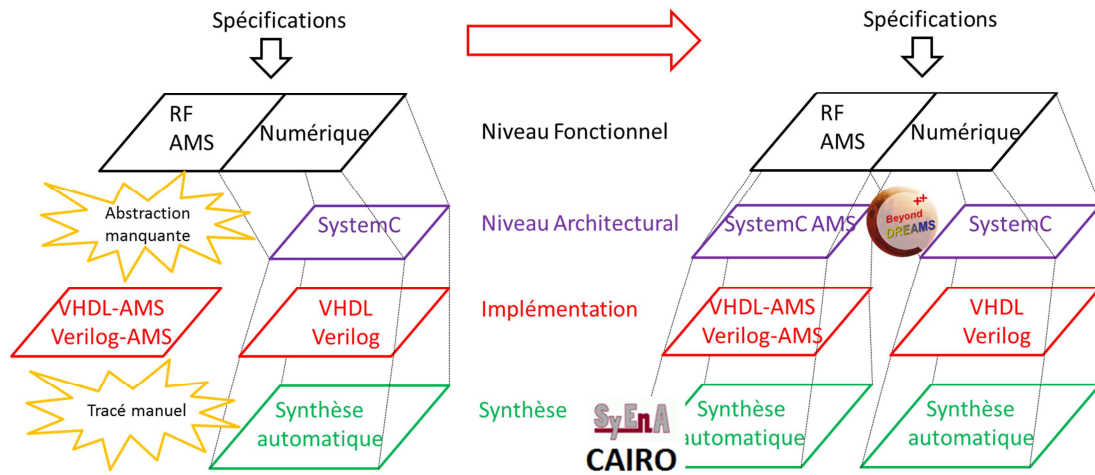
Figure 1. Positionnement de B-DREAMS par rapport au flot AMS
