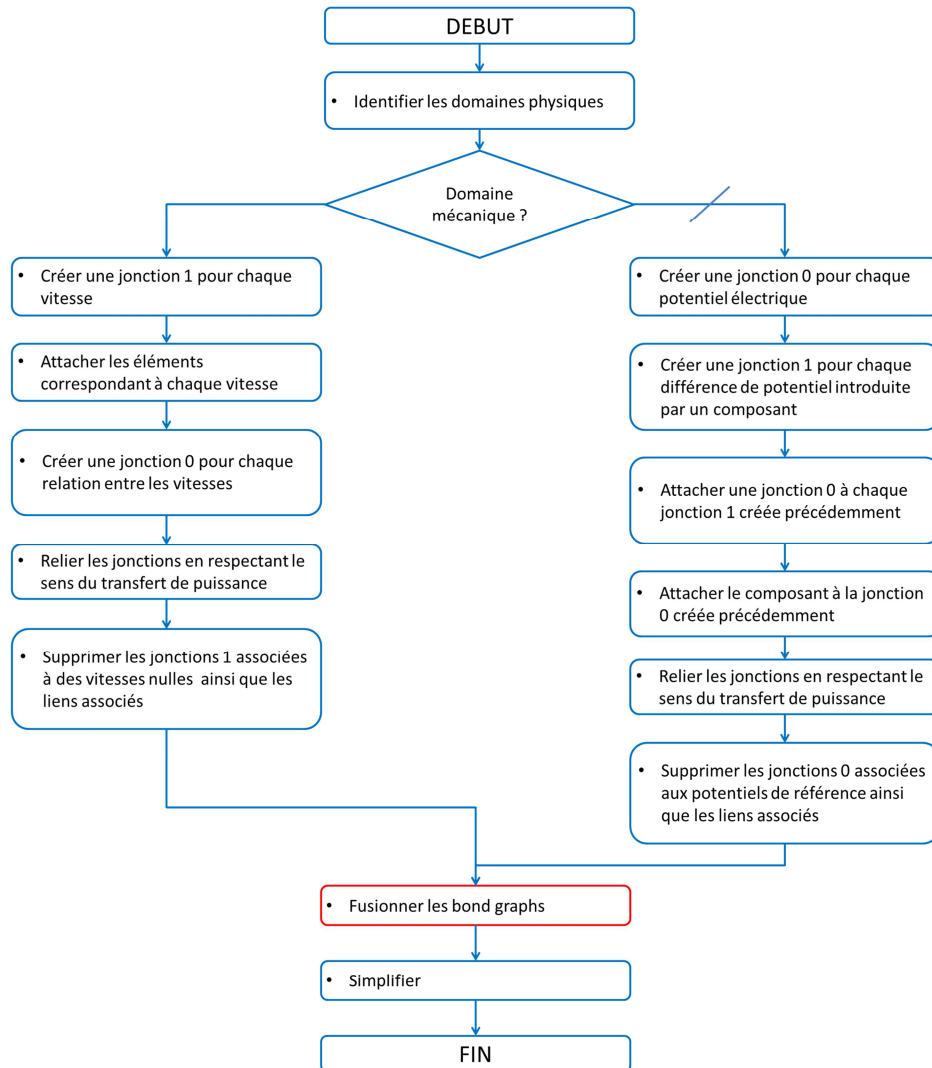
Figure 58. Méthode de construction du bond graph d'un système électromécanique
