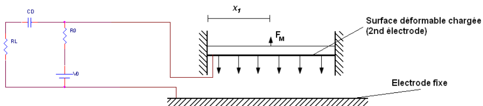
Figure 52. Représentation du capteur de force
