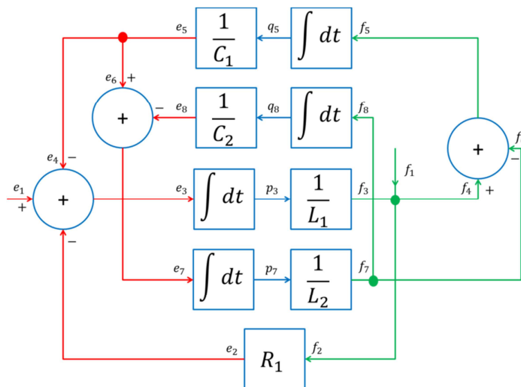
Figure 67. Schéma-bloc conservatif de l'exemple
