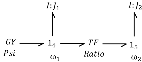
Figure 73. Bond graph de la partie mécanique du système moteur-réducteur
