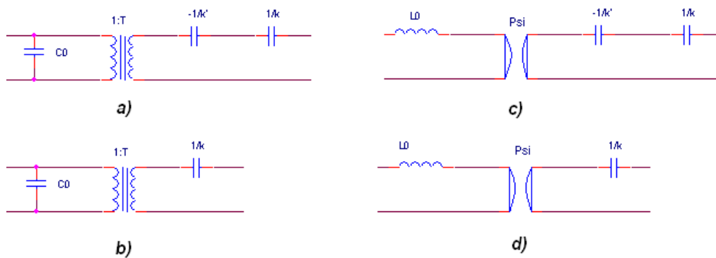
Figure 42. Circuits équivalents des transducteurs électromécaniques couplés à un ressort
