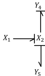
Figure 70. Bond graph déduit de la troisième ligne de la matrice BG
