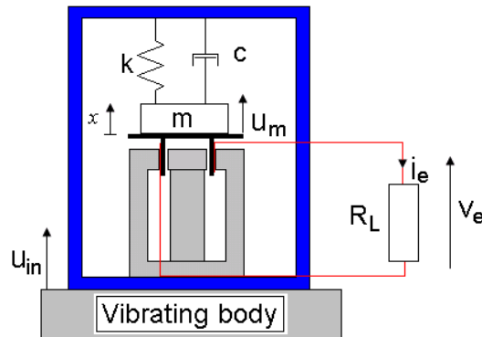
Figure 43. Capteur de vibrations
