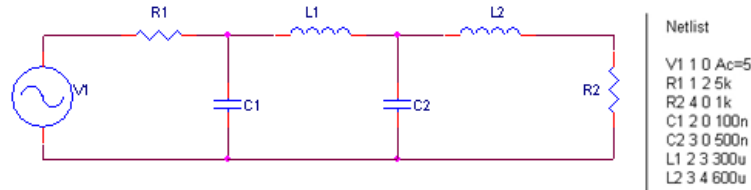
Figure 32. Filtre passif du quatrième ordre
