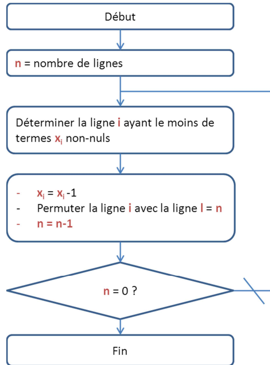
Figure 29. Algorithme des permutations de lignes
