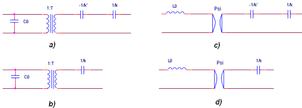
Figure 42. Circuits équivalents des transducteurs électromécaniques couplés à un ressort
