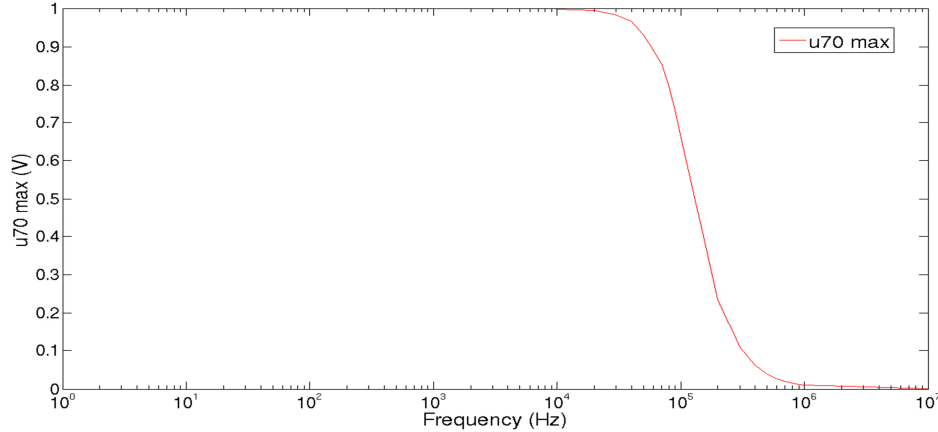
Figure 39. Tension de sortie du filtre à variables d'état
