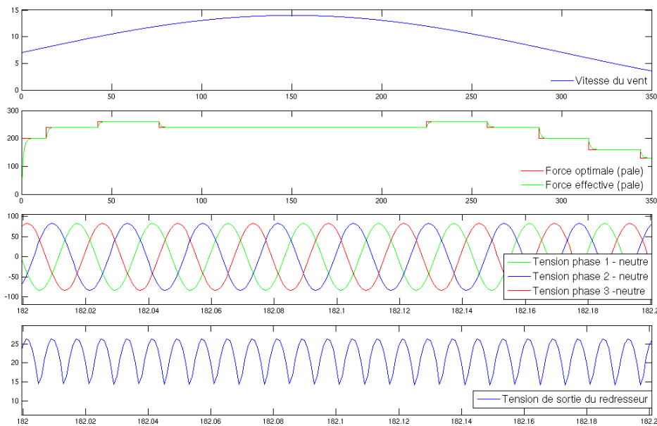
Figure 90. Simulation de l'éolienne - Comportement
