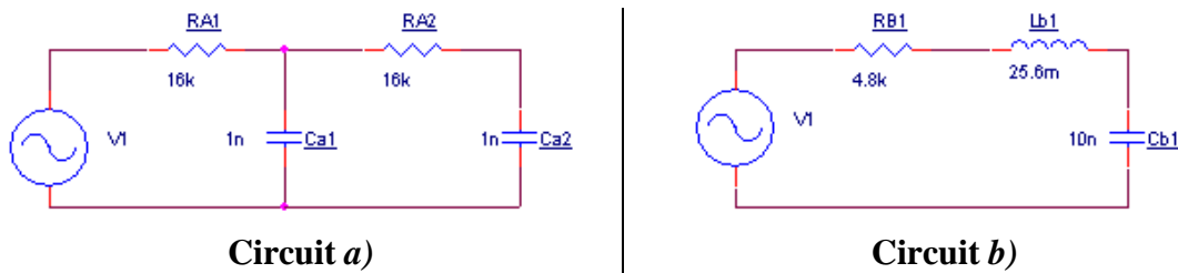
Figure 36. Deux topologies différentes pour un même comportement
