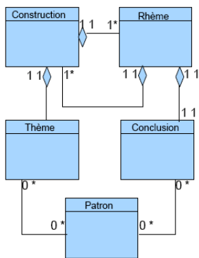
Figure 3.9. Diagramme UML structure des données du modèle
