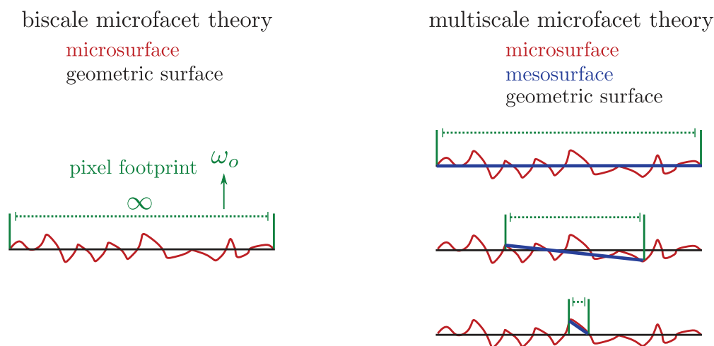
FIGURE 5.1 – (gauche) La théorie standard des micro-facettes est bi-échelles et suppose que la micro-surface soit très petite par rapport à l'échelle d'observation. (droite) Cette hypothèse ne tient plus dans une théorie multi-échelles où l'échelle d'observation est ajustée en fonction de la distance de l'observateur.
