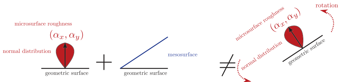
FIGURE 5.3 – La micro-surface décentrée n'est pas la micro-surface tournée et alignée autour de la méso-normale. Les statistiques de rugosité de la micro-surface ne sont pas conservées lorsqu'on change de repère. Il n'est donc pas possible de se ramener au modèle bi-échelles où la méso-surface et la surface géométrique sont confondues en faisant une rotation du repère géométrique.
