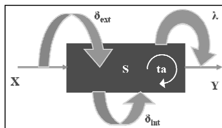
Figure I-8 : Modèle atomique DEVS
