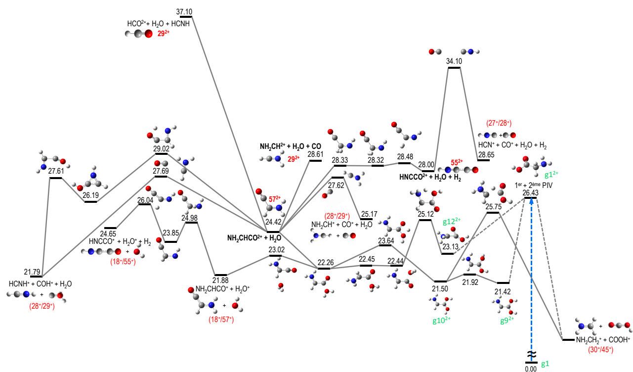
Figure 5.26 : Voies de fragmentation du dication de glycine à partir des isomères g9 2+ , g10 2+ et g12 2+ donnant des fragments doublement chargés. La voie d'entrée est donnée par le premier potentiel d'ionisation verticale à partir du conformère de glycine neutre le plus stable (g1). Les énergies relatives sont données en électron-volt par rapport à (g1).
