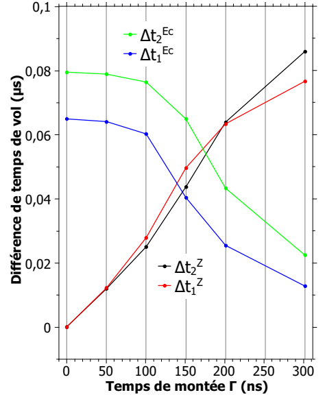
Figure 3.48 : Évolution des différents paramètres caractérisant la forme d'un îlot de corrélation ( \Delta t_i^Z , \Delta t_i^{E_c} ) en fonction du temps de montée des électrodes d'extraction. Exemple pour la corrélation des fragments 1/2 de la glycine.
