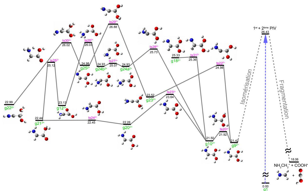
Figure 5.16 : Isomères stationnaires du dication de glycine (en vert) ainsi que les états de transition associés (en violet). Les énergies relatives sont données en électron-volt par rapport au conformère de glycine neutre le plus stable (g1). La voie de droite correspond à la fragmentation du dication de glycine par rupture de la liaison C-C α .
