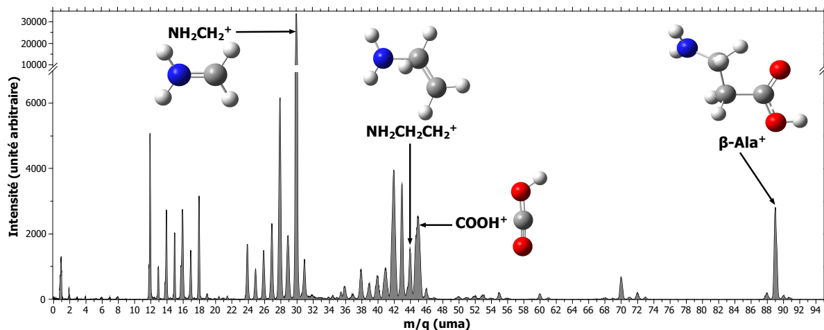
Figure 5.29 : Spectre de masse des produits cationiques résultant de l'interaction de la molécule neutre de β-alanine avec des ions O 6+ ayant une énergie de 48 keV.
