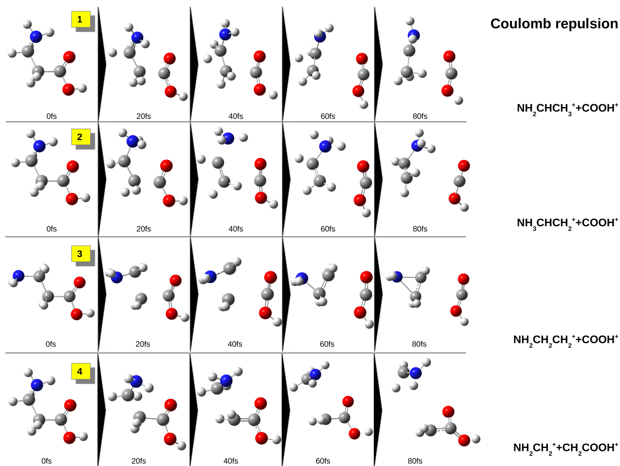
Figure A.6 : Capture des simulation de dynamique moléculaire du dication de \beta -alanine dans l'état fondamental singulet à différents instants de 0 à 80 fs.
